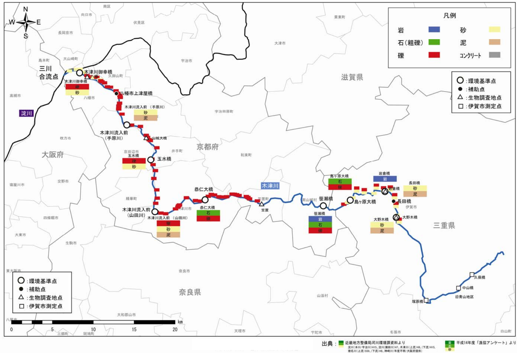
図10.10 河床材料図(木津川)
