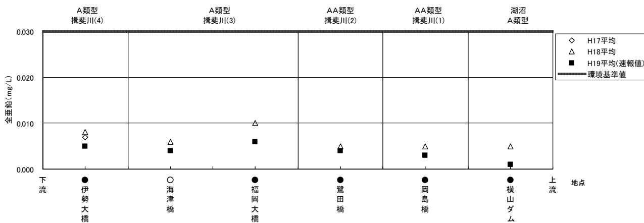
揖斐川 全垂鉛濃度縦断分布図
