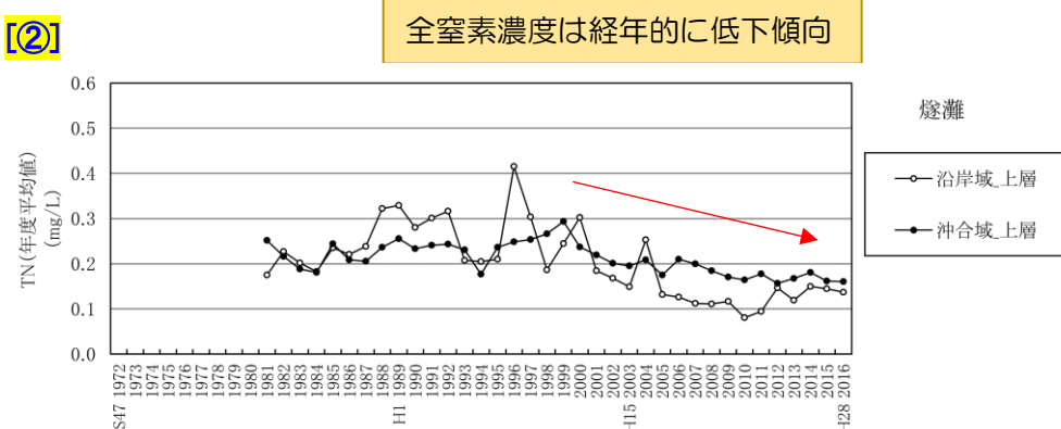
図 全窒素濃度の推移
