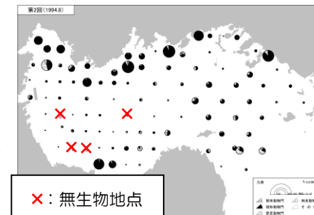
図 底質及び底生生物の水平分布図
