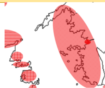
図 赤潮発生場所例(2015年8月)
