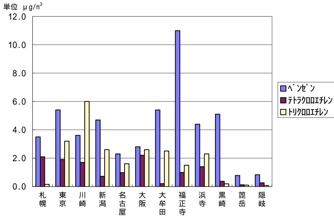
図2 ベンゼン、トリクロロエチレン、テトラクロロエチレンの大気環境濃度
