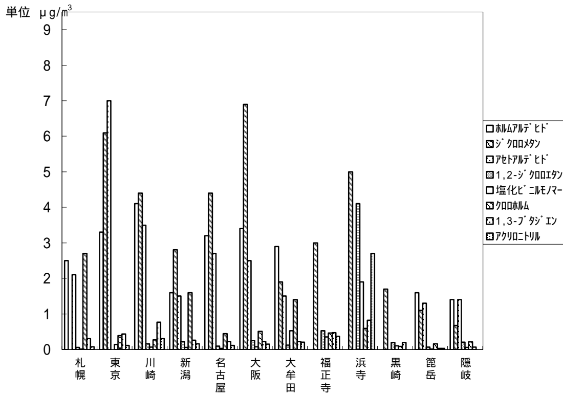
図3 その他の物質の大気環境濃度
