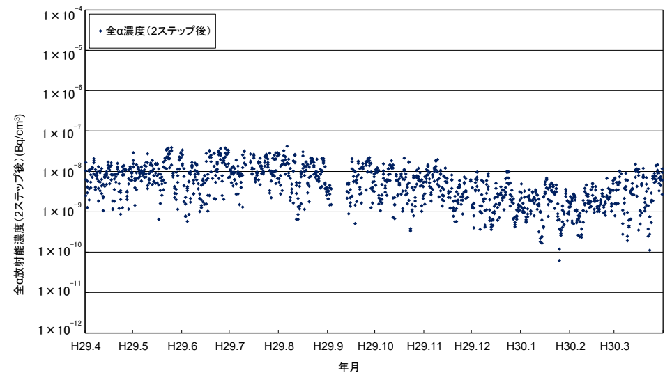
越前岬測定所における大気浮遊じん全α放射能濃度(2ステップ後)の経時変化
