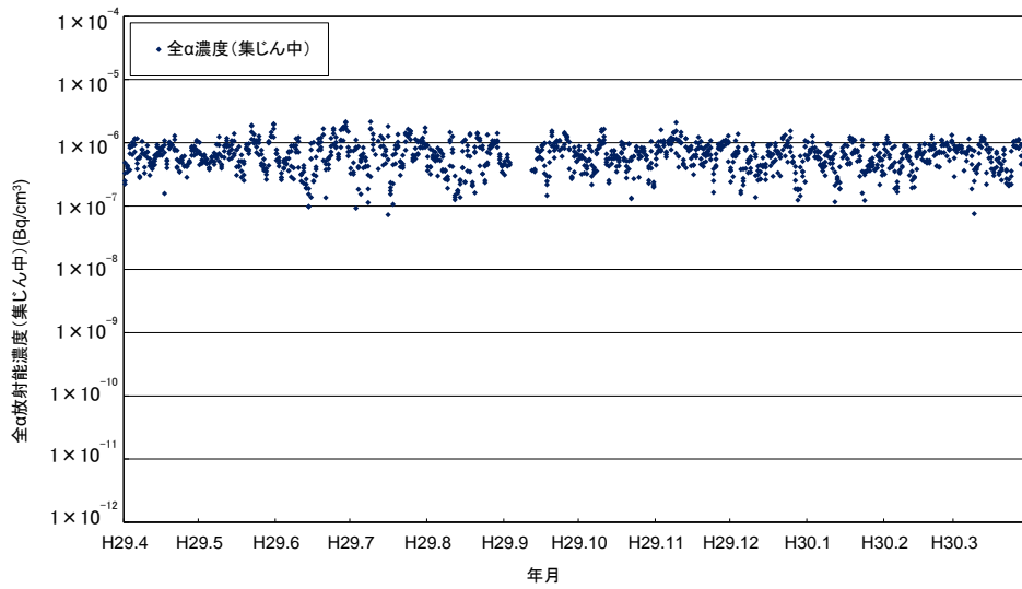
越前岬測定所における大気浮遊じん全α放射能濃度(集じん中)の経時変化
