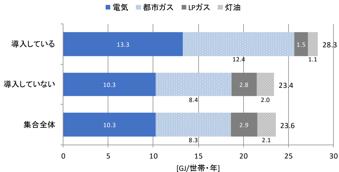
図 2-143 建て方別HEMSの使用有無別世帯当たり年間エネルギー種別消費量（集合）
