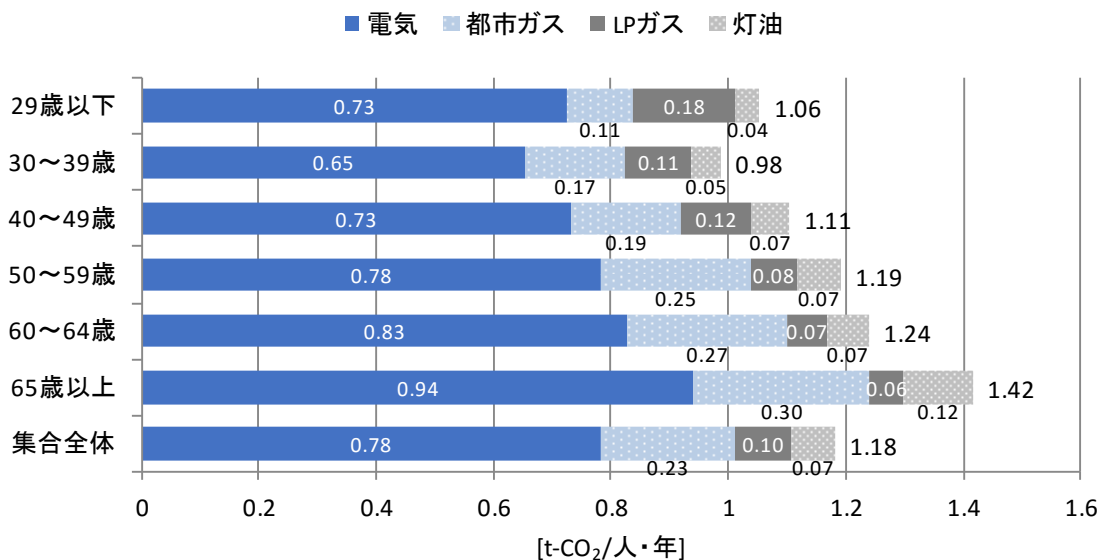
参考図 1-9 建て方別世帯主年齢別 1人当たり年間エネルギー種別 CO 2 排出量 (集合)
