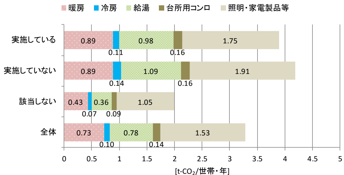
参考図 2-78 省エネルギー行動実施状況別世帯当たり年間用途別 CO 2 排出量<家族が続けて入浴するようにしている>
