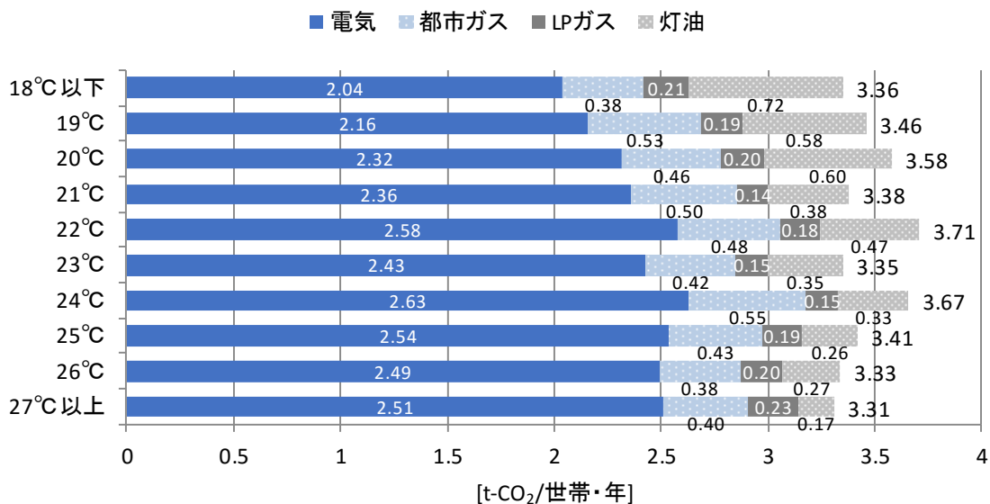
図 2-72 最もよく使う暖房機器の設定温度別世帯当たり年間エネルギー種別CO 2 排出量
