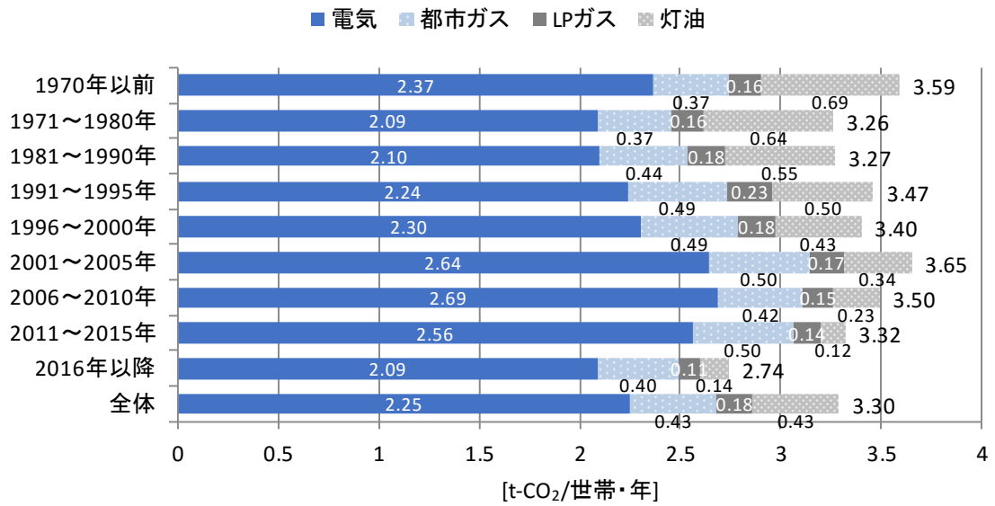
図 1-21 建築時期別世帯当たり年間エネルギー種別CO 2 排出量
