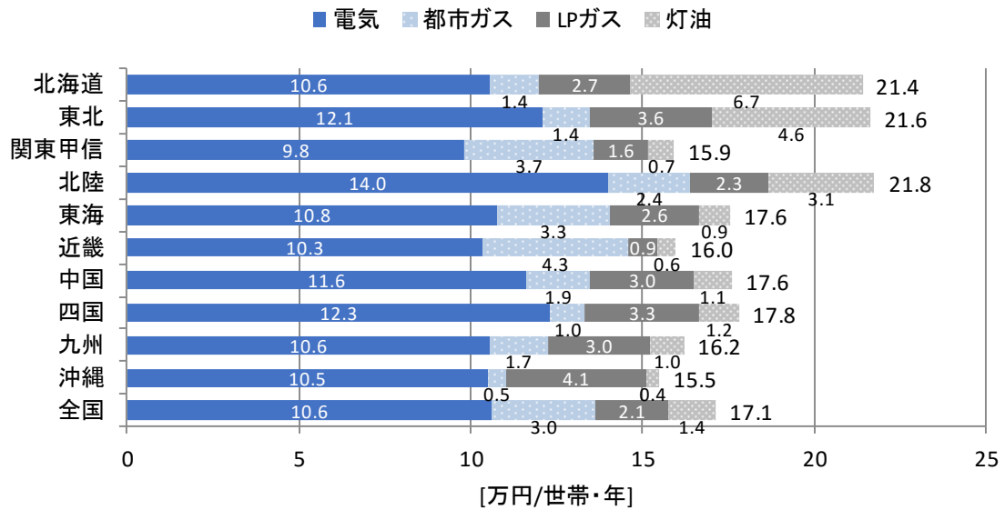
図 1-60 地方別世帯当たり年間エネルギー種別支払金額
