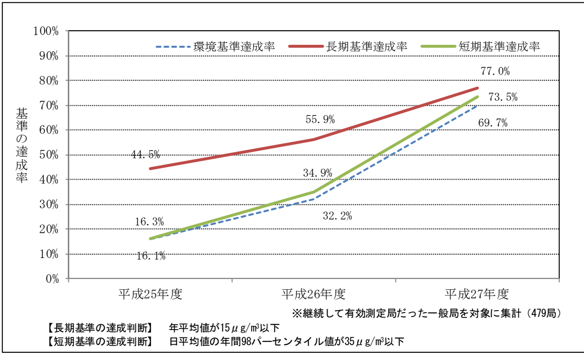
図 6-5 平成 25~27 年度連続有効測定局における環境基準達成状況の推移（一般局）
