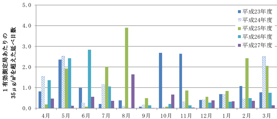
図 6-3 日平均値が 35 \mu\text{g}/\text{m}^3 を超えた延べ日数（一般局）
