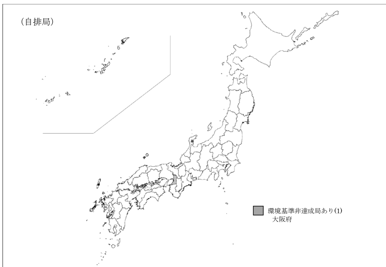
図 2 - 3 浮遊粒子状物質の環境基準非達成局の分布
