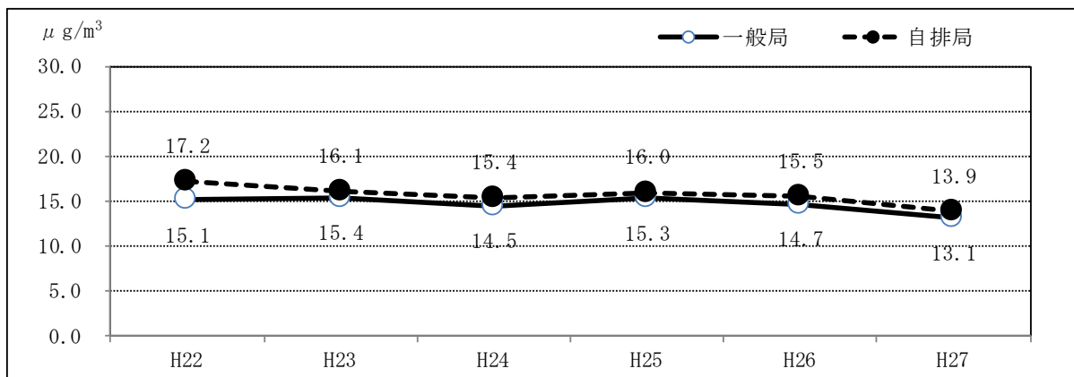
図6-1 微小粒子状物質の年平均値の推移
