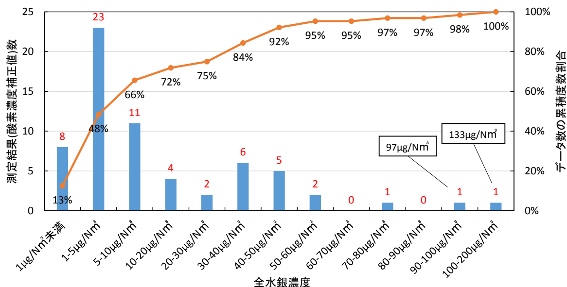
図Ⅱ-4-2-1 排ガス中全水銀濃度 ヒストグラム（一般廃棄物焼却炉）
