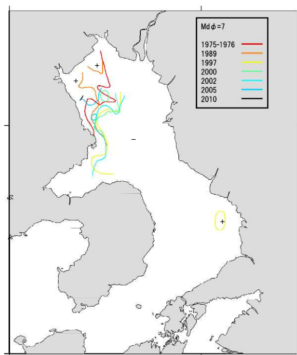
図 4.4.59 Md\phi=7 の等値線の比較
