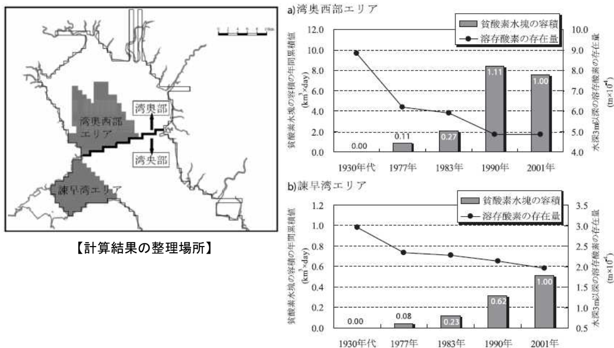
図 3.6.13 貧酸素水塊の容積の年間累積値と溶解酸素の存在量 (8 月平均値) の変化
