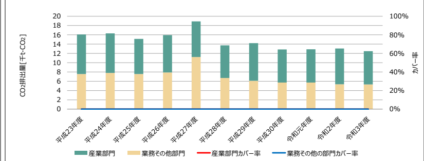
区域のエネルギー起源CO2排出量 (千t-CO2)
