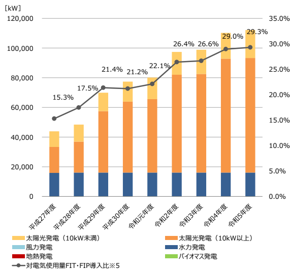
3) 区域の再生可能エネルギーの導入設備容量の推移 (累積)
