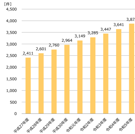
4) 区域の太陽光発電 (10kW未満※6) 設備の導入件数の推移 (累積)
