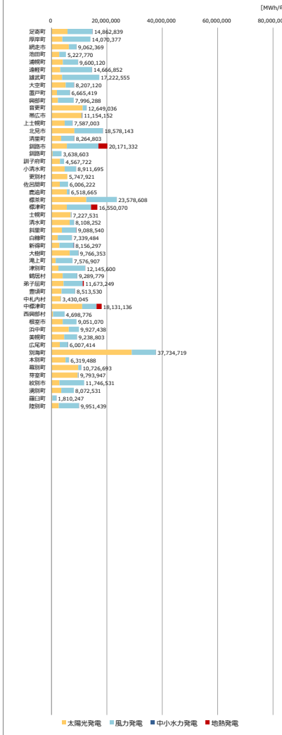
5) 同一都道府県内における他地方公共団体の再エネポテンシャル(発電電力量)の比較 [MWh/年]
