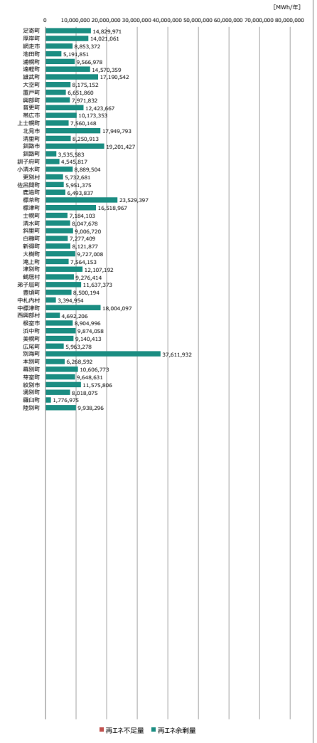
7) 同一都道府県内の他地方公共団体の再エネ不足量・余剰量の比較 [MWh/年]
