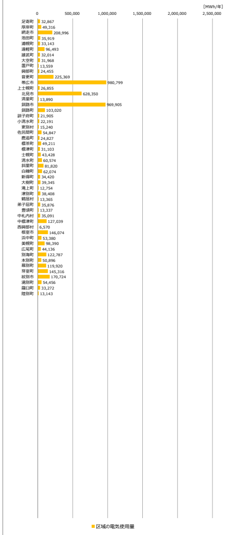
6) 同一都道府県内における他地方公共団体の電気使用量の比較 [MWh/年]
