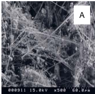
アスベストの処理前(A)後(B)の電子顕微鏡写真とX線回折(C). 処理後のアスベストは塊となり結晶構造は消失する。
