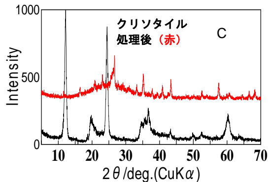
アスベストの処理前(A)後(B)の電子顕微鏡写真とX線回折(C). 処理後のアスベストは塊となり結晶構造は消失する。
