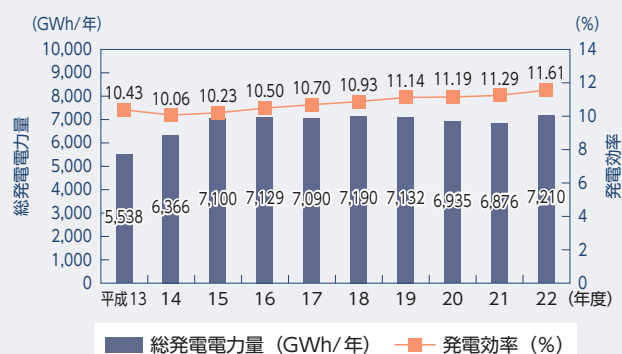
一般廃棄物処理施設の総発電電力量と発電効率の推移
