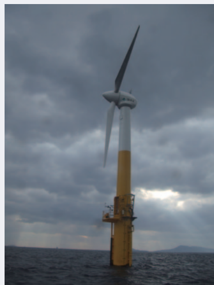
五島沖の浮体式洋上風力発電施設
