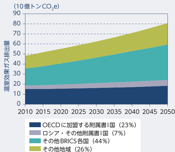
世界の二酸化炭素排出量予測
