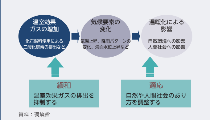
適応策と緩和策
