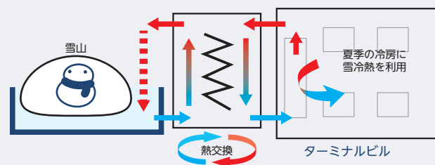
千歳空港の雪氷熱冷房システム
