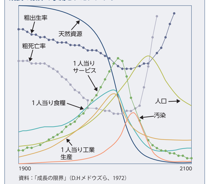
成長の限界で予測されたシナリオ
