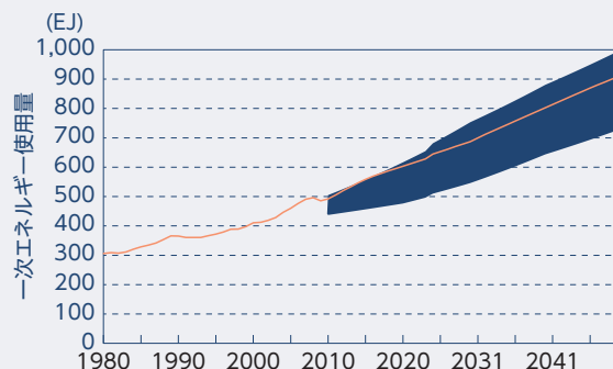
世界のエネルギー需要予測
