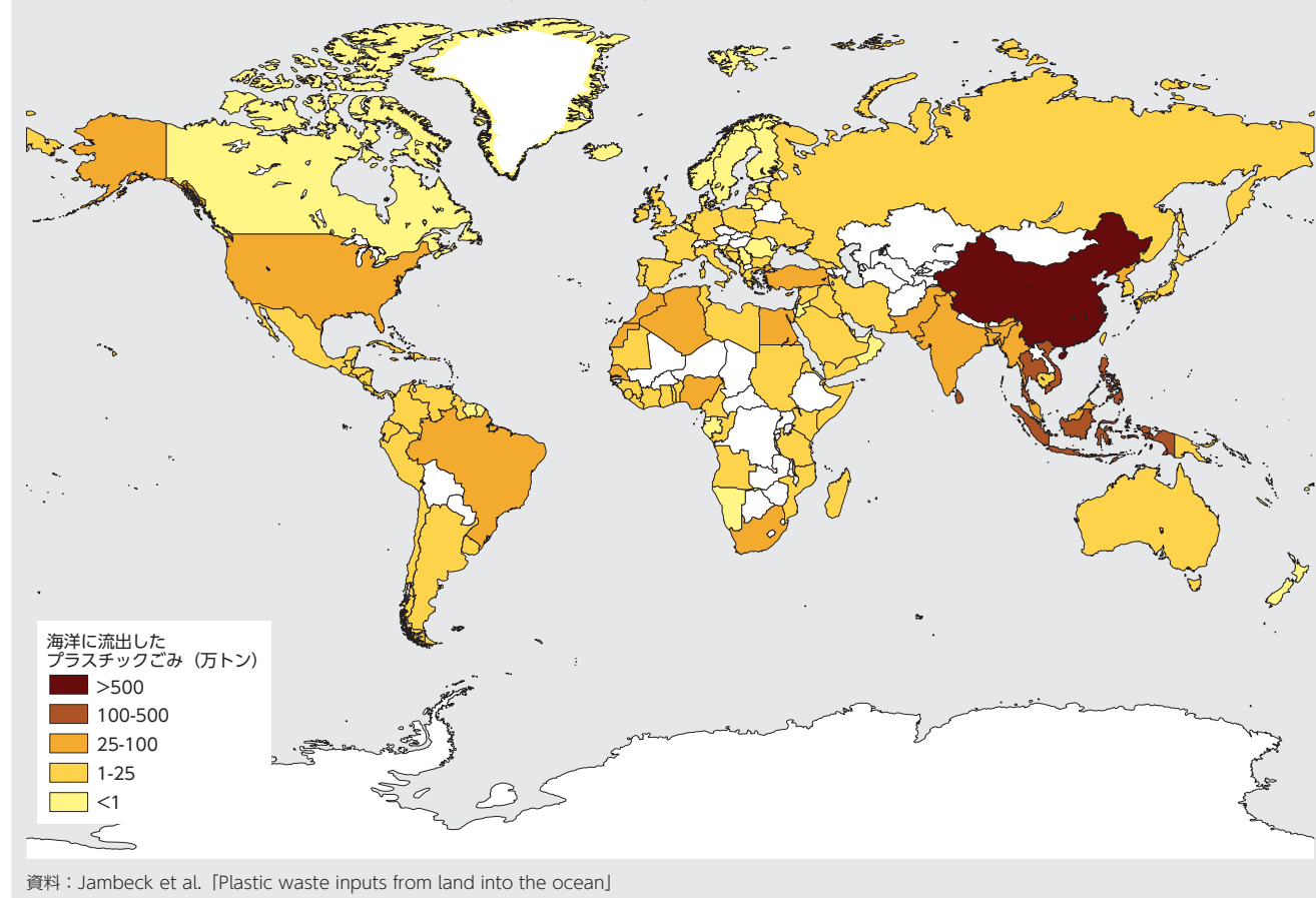
図1-2-12 海洋に流出したプラスチックごみ（2010年推計）
