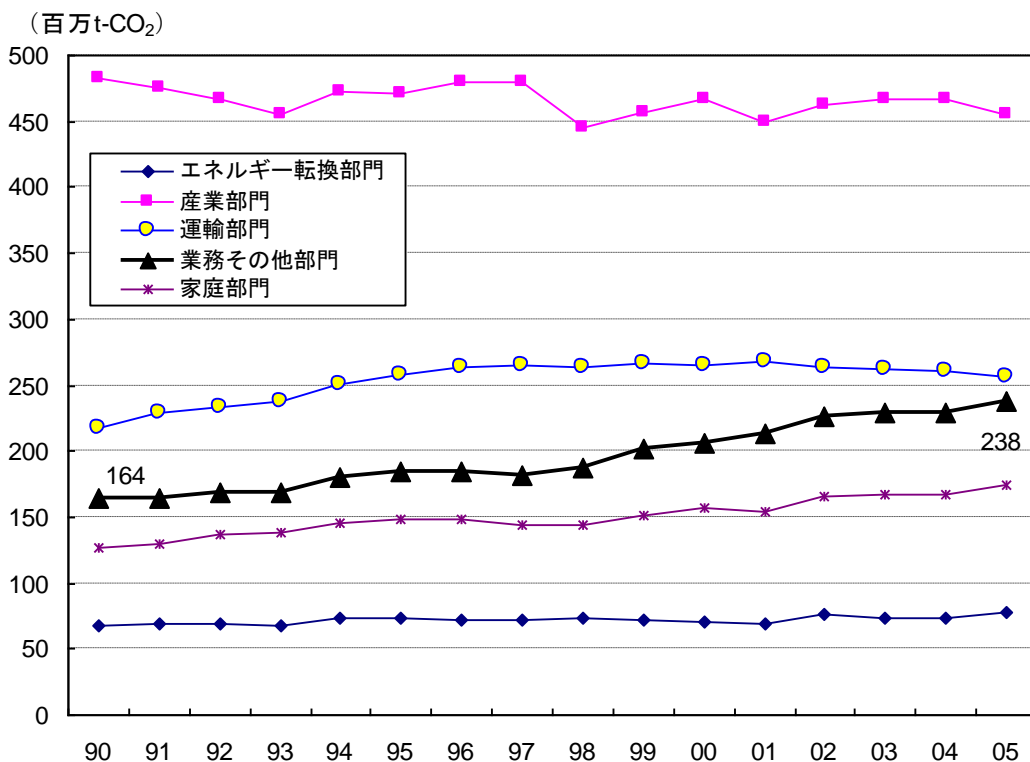
図VI-1-1 我が国における部門別エネルギー起源二酸化炭素排出量の推移
