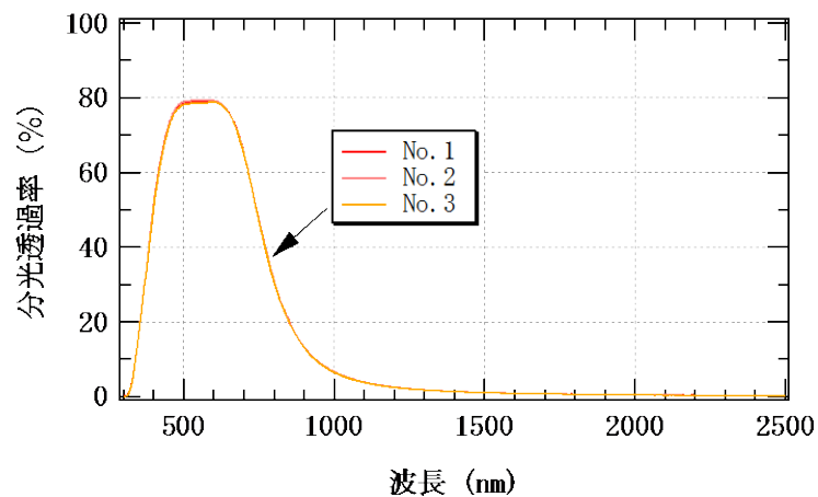
図 5-1 分光透過率測定結果（実証対象技術単体）
