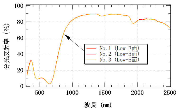
図 5-2 分光反射率測定結果（実証対象技術単体）
