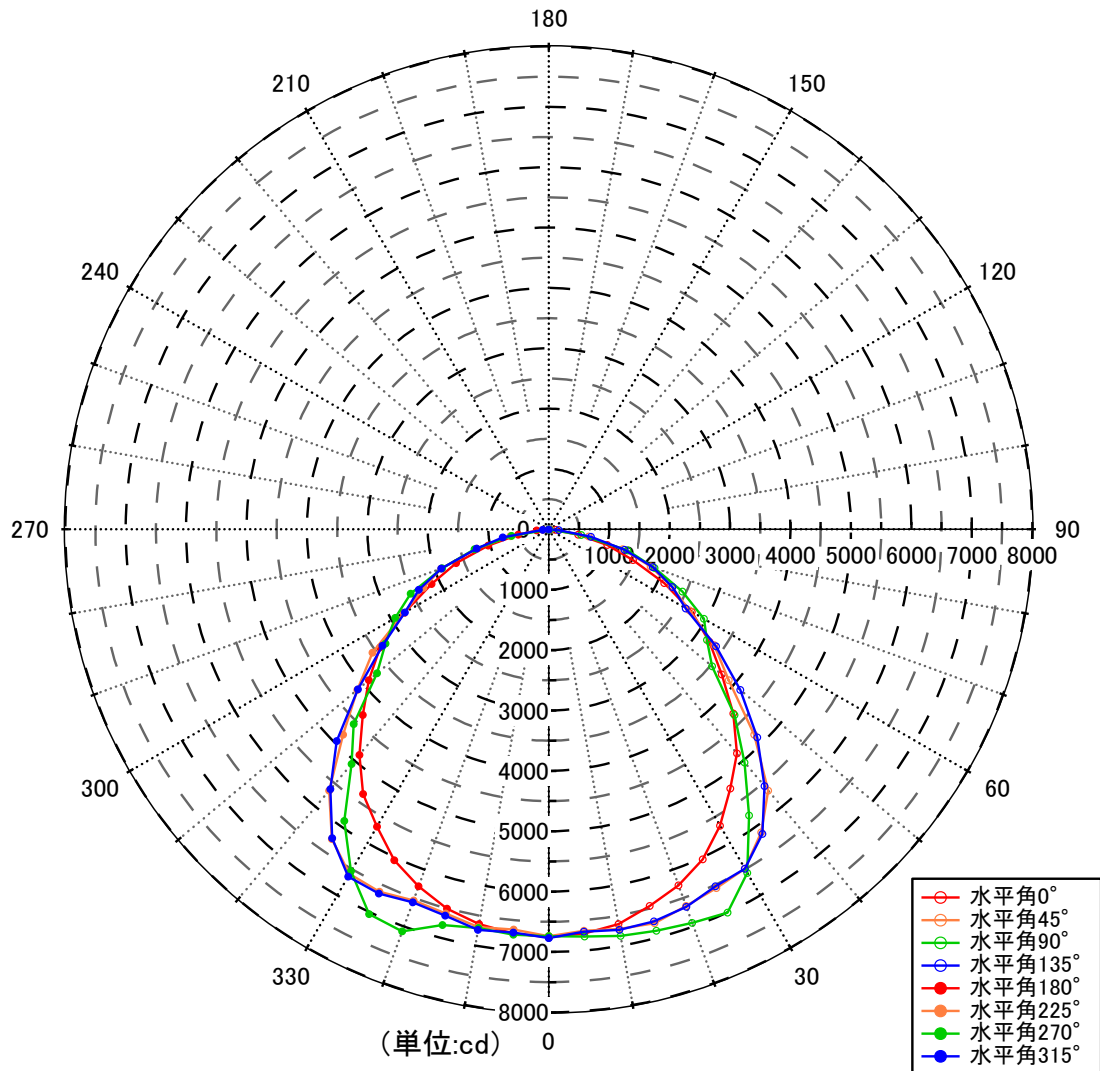
図 6-3 配光曲線
