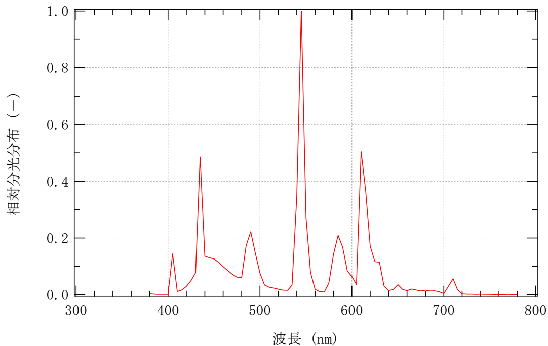
図 6-5 相対分光分布測定結果
