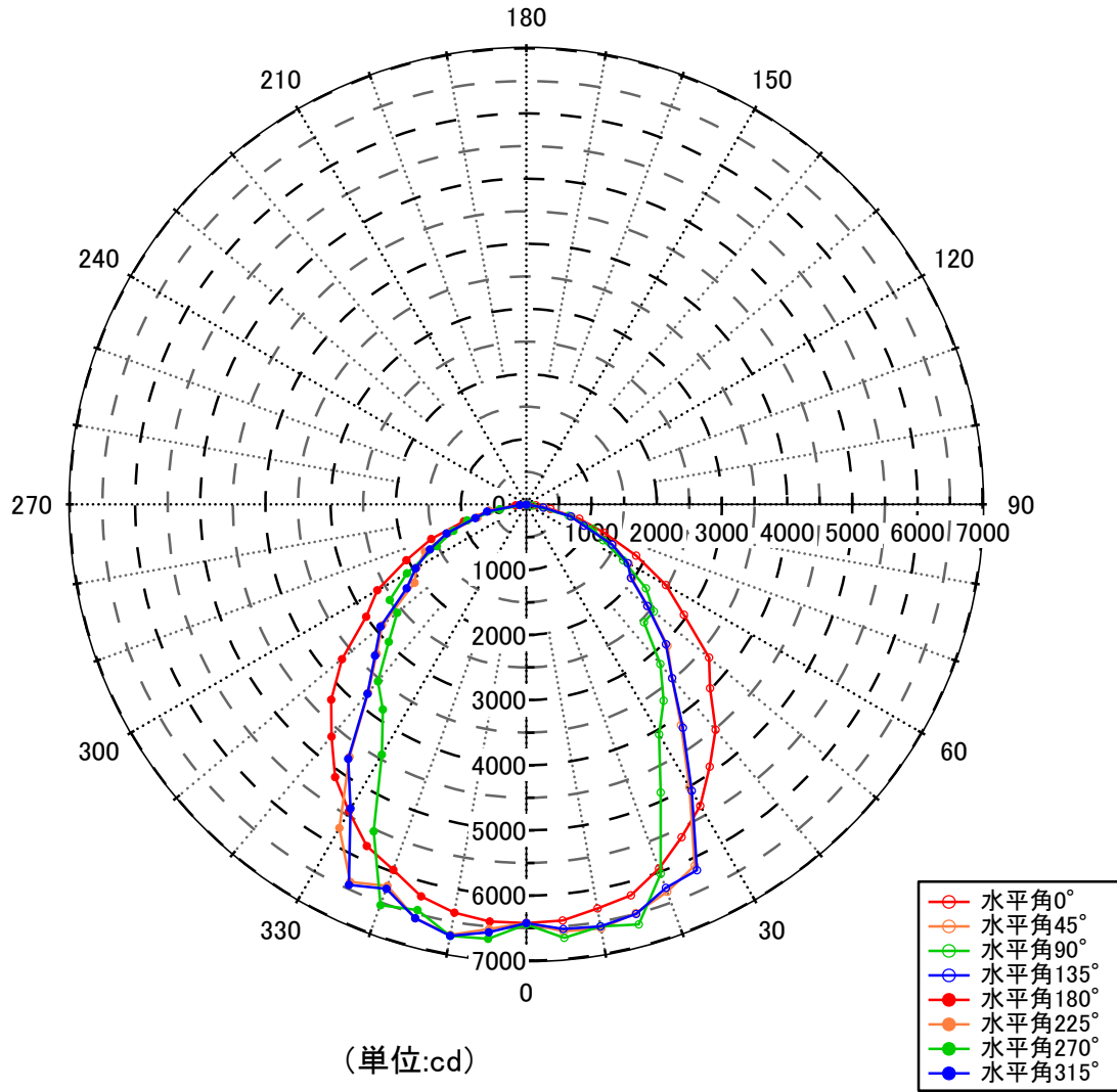
図 6-3 配光曲線
