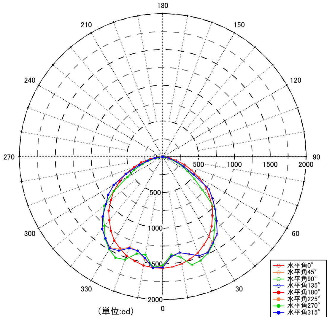
図 6-3 配光曲線
