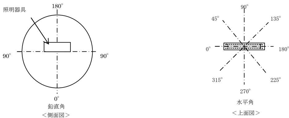
図 6-3 配光曲線
