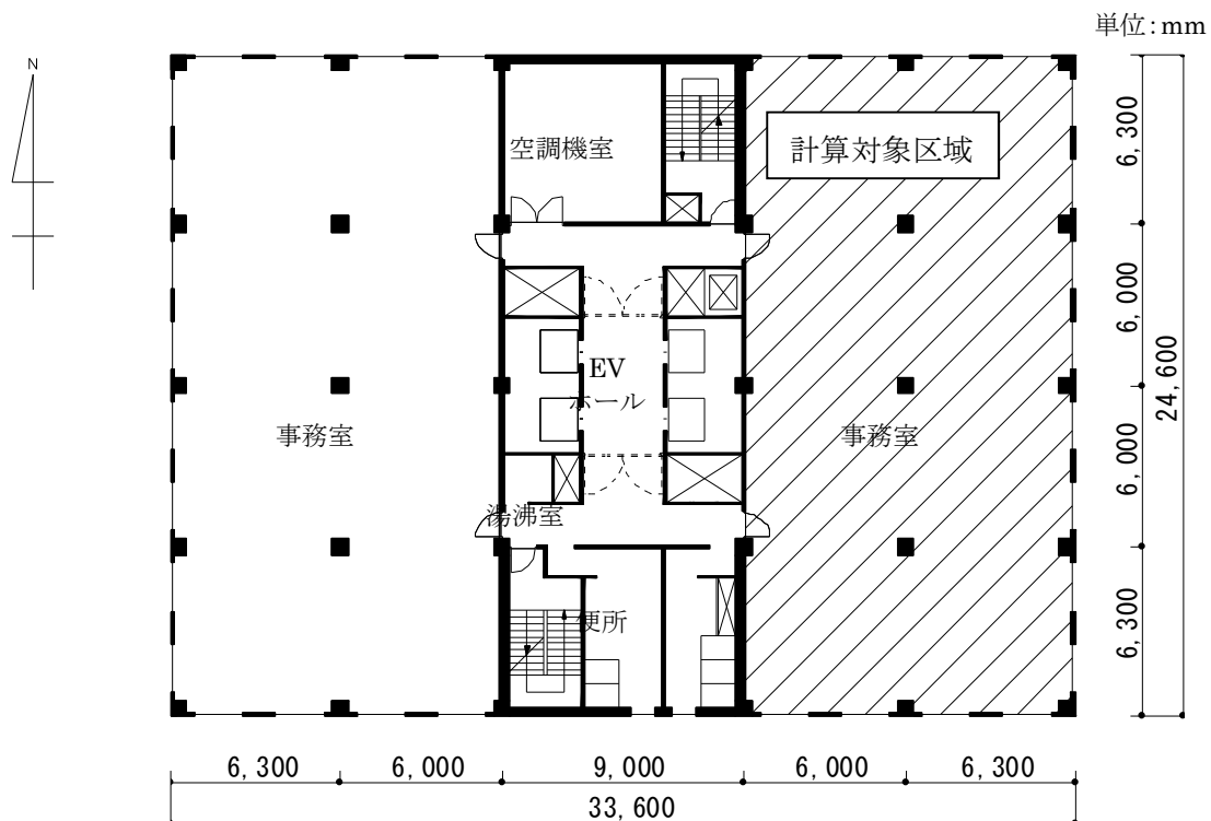
図 6-8 計算用オフィスモデル（平面図）
