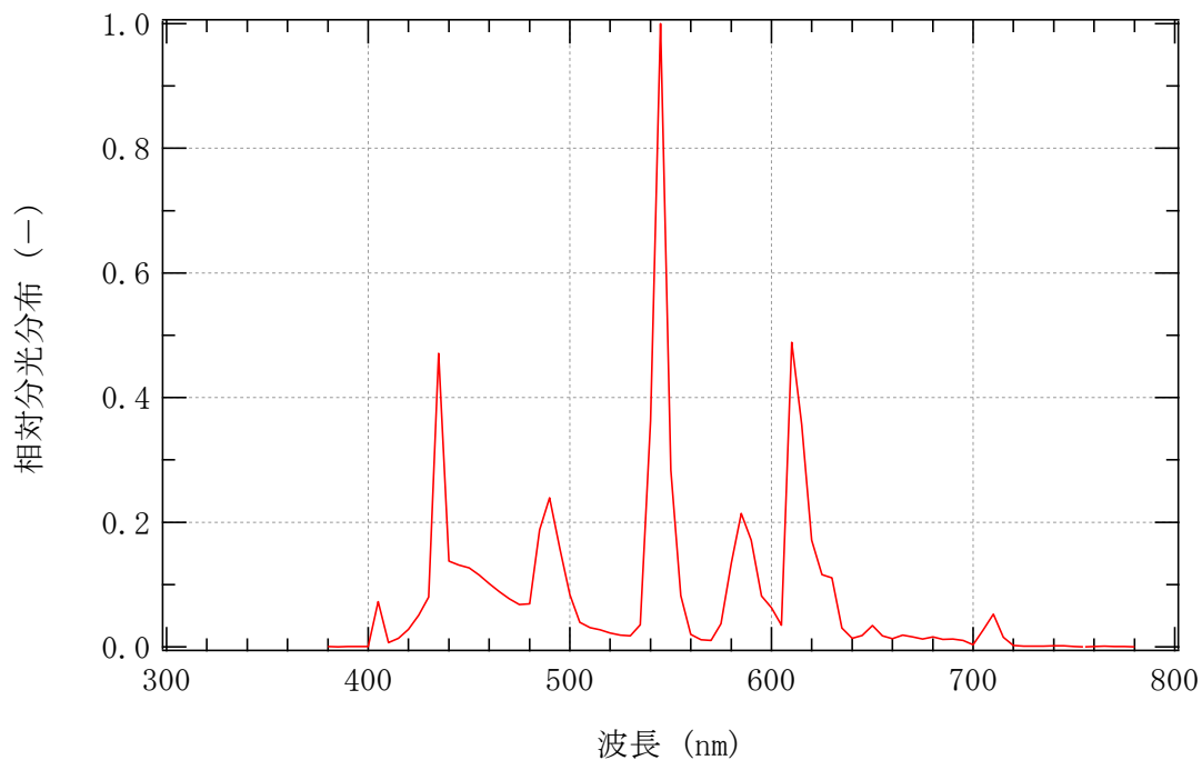
図 6-7 相対分光分布測定結果
