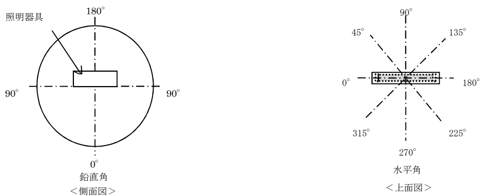
図 6-5 配光曲線
