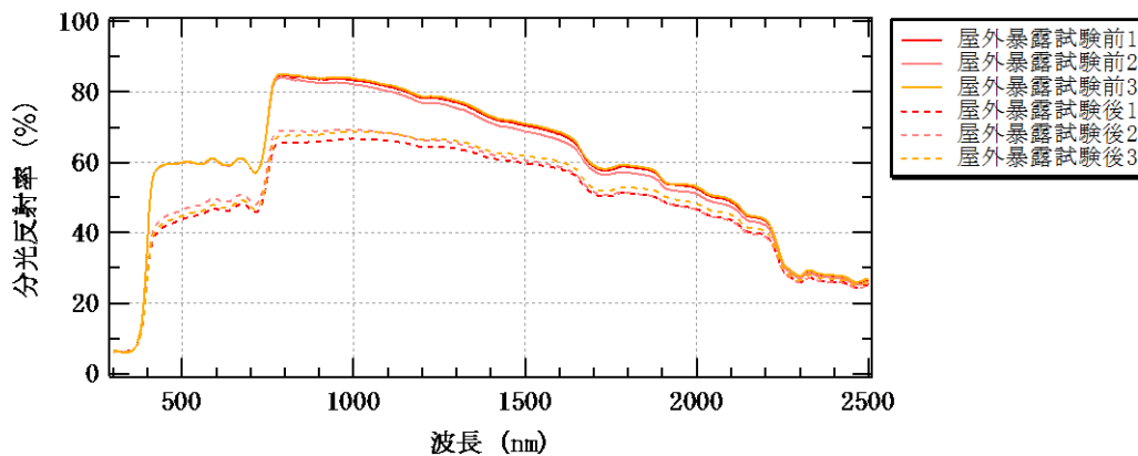
図 5-3 分光反射率測定結果(ホワイト)
