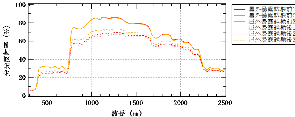
図 5-2 分光反射率測定結果(グレー)
