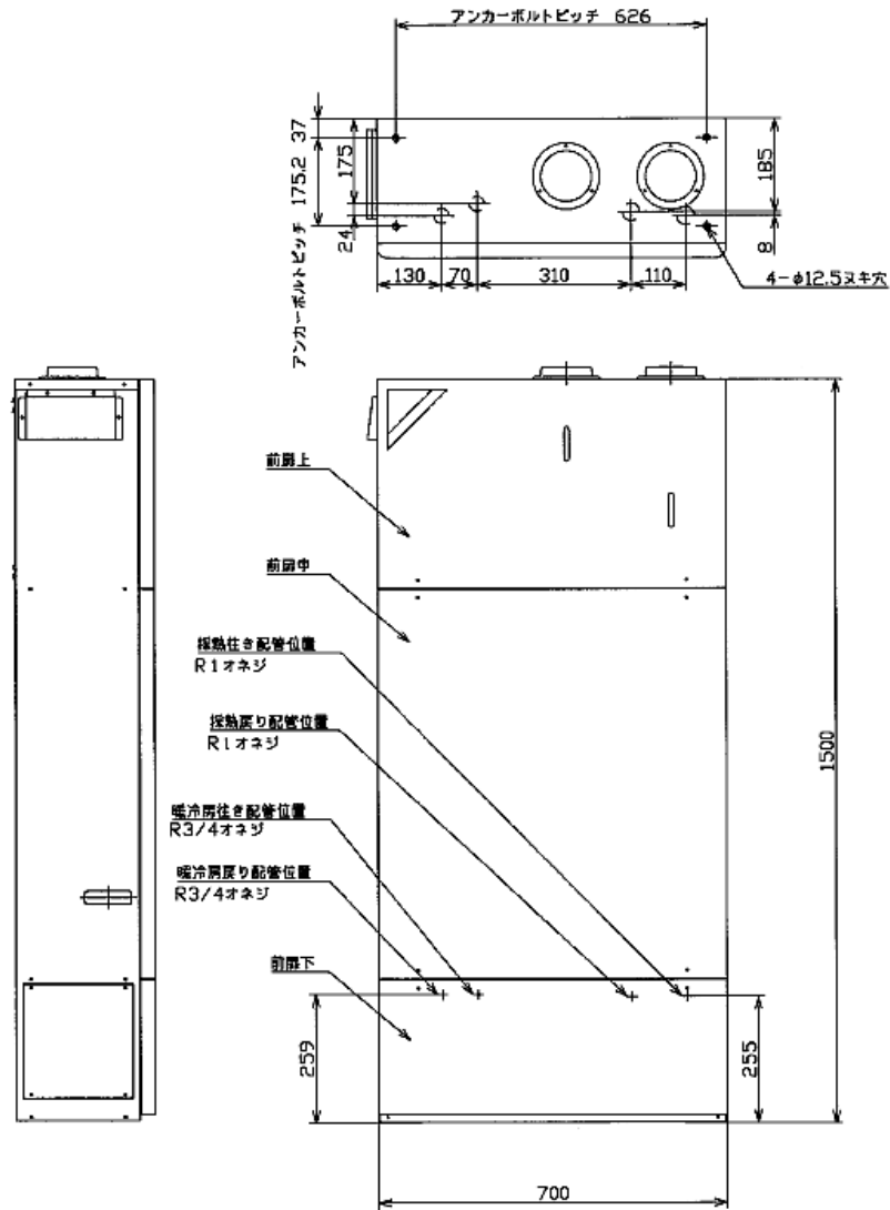
図 3-3 実証対象技術外形図 (地中熱ヒートポンプユニット GSHP-1001F)
