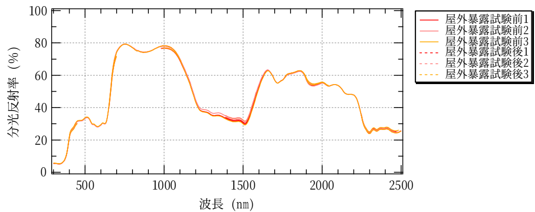
図 2 分光反射率測定結果（灰色）
