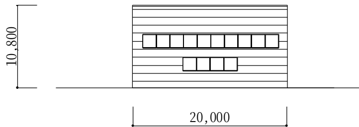
付図 2 計算用工場モデル（東側立面図）
