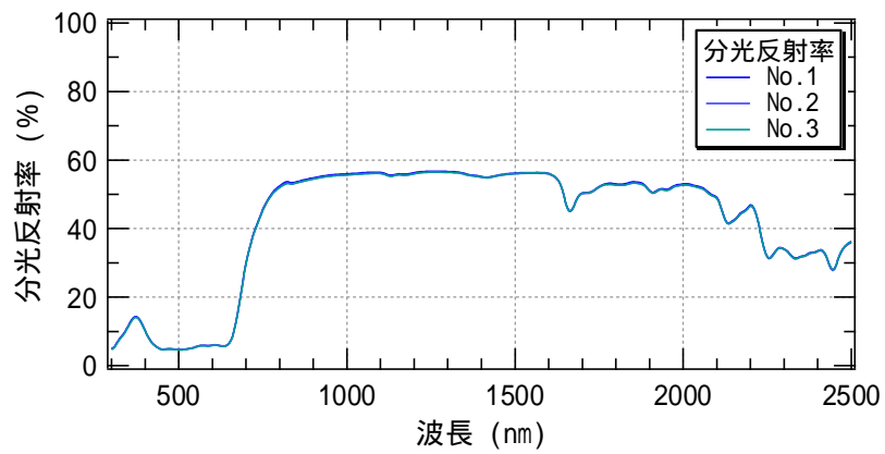
図 5-3 分光反射率測定結果 (色名 ダークブラウン)
