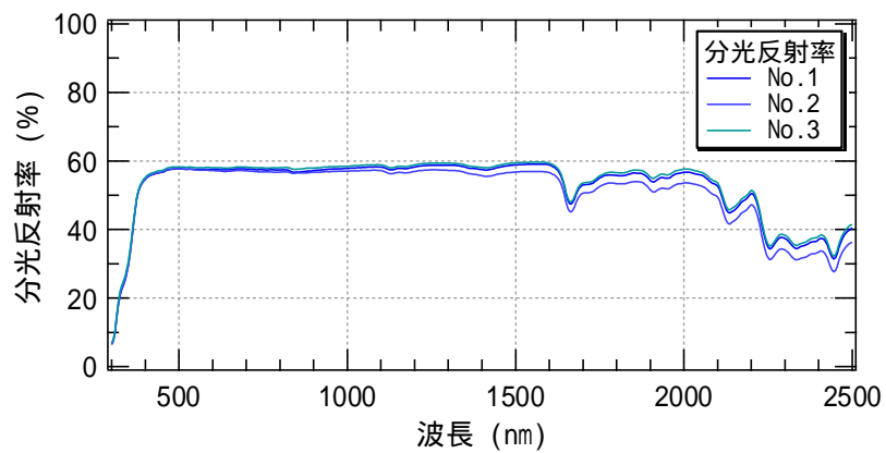
図 5-4 分光反射率測定結果 (色名 ホワイト)
