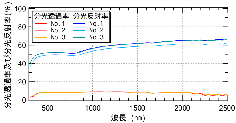
図 5-2 分光透過率及び分光反射率測定結果（色名 ホワイト ）
