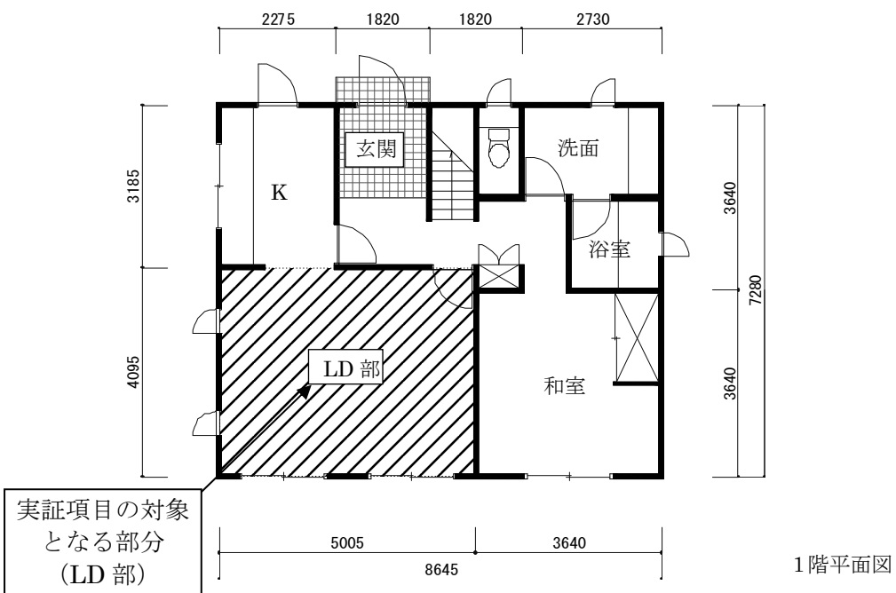
図 4-1 計算用住宅モデル (平面図)
