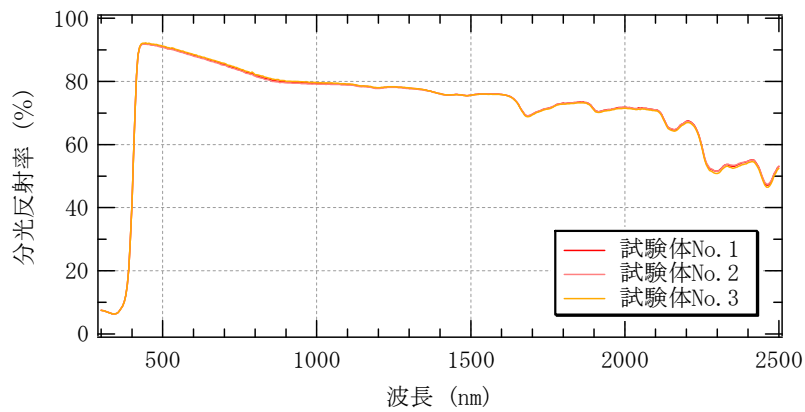
図 5-3 分光反射率測定結果 (C059S [ホワイト])
