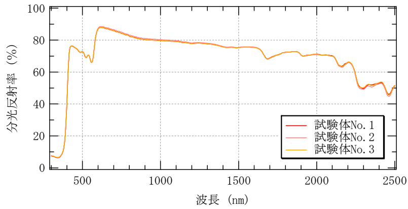
図 5-2 分光反射率測定結果 (C154S [ピンク])
