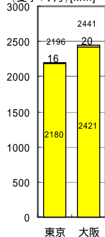
冷房負荷低減効果 (オフィス) (夏季1ヶ月)[kWh]
