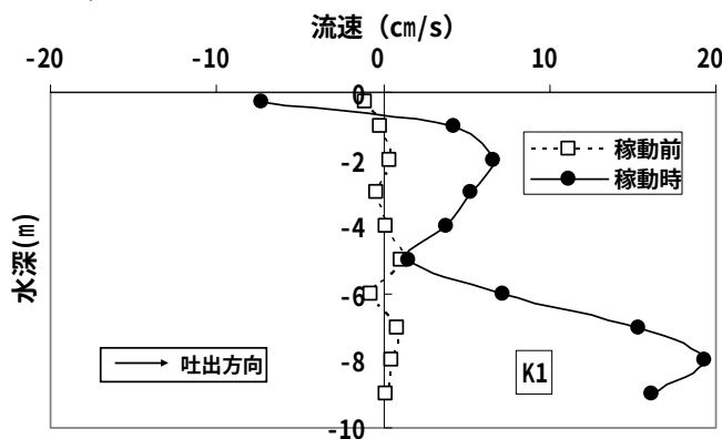
図 4-1-10 流向流速測定結果
