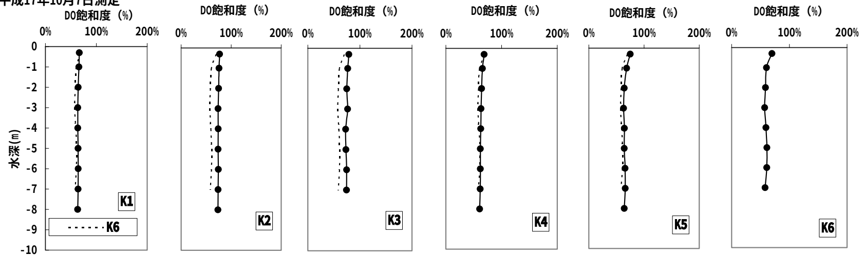
鹿川貯水池における DO 飽和度分布図 (平成 17 年 9 月 29 日, 10 月 7 日)
