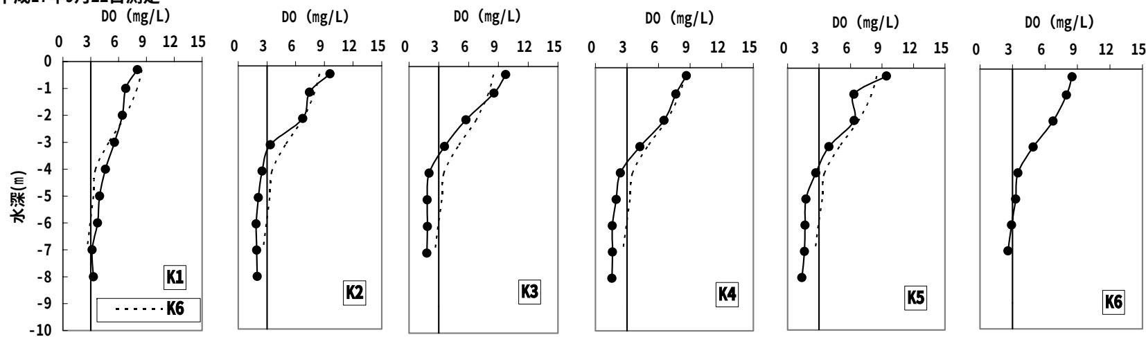
鹿川野水池における DO 分布図 (平成 17 年 9 月 16 日, 22 日)
