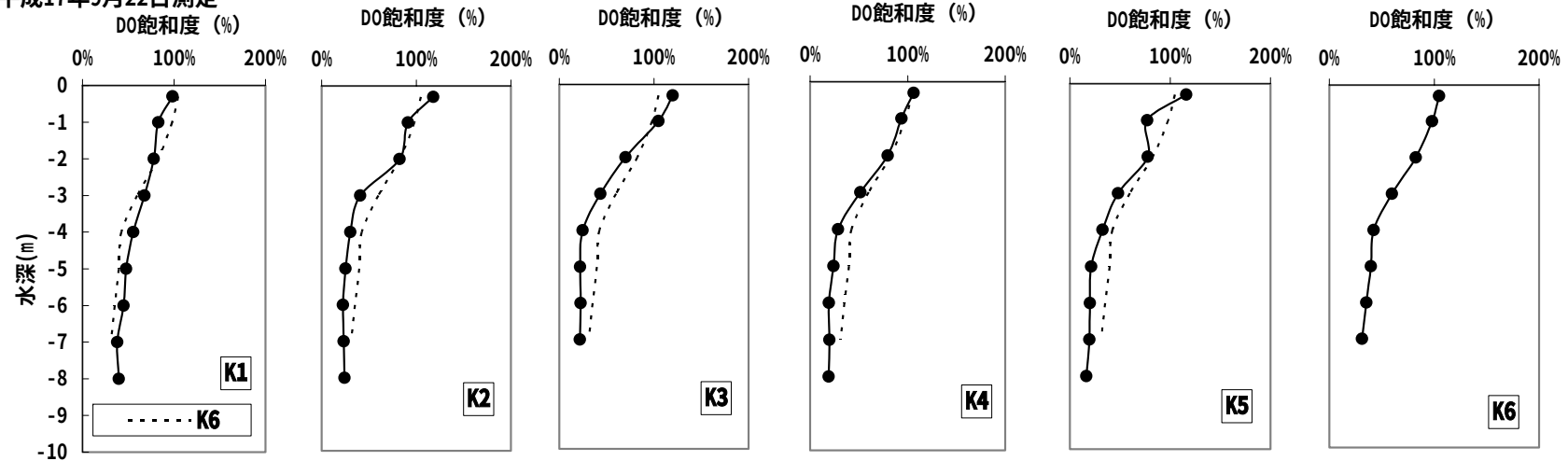
鹿川貯水池における DO 飽和度分布図（平成 17 年 9 月 16 日, 22 日）
