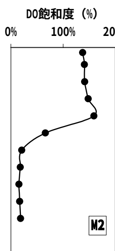
三高貯水池における DO 飽和度分布図 (平成 17 年 8 月 4 日, 11 日, 19 日, 29 日, 9 月 16 日, 22 日)
