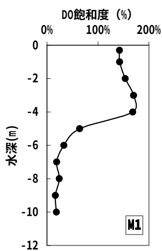
三高貯水池における DO 飽和度分布図 (平成 17 年 8 月 4 日, 11 日, 19 日, 29 日, 9 月 16 日, 22 日)
