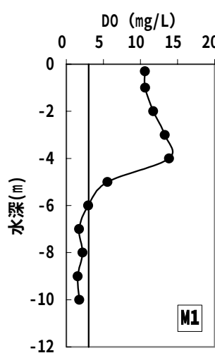
三高貯水池における DO 分布図 (平成17年8月4日, 11日, 19日, 29日, 9月16日, 22日)
