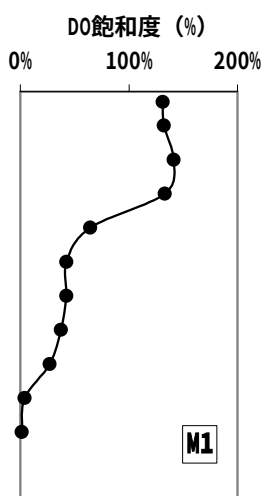
三高貯水池における DO 飽和度分布図 (平成 17 年 8 月 4 日, 11 日, 19 日, 29 日, 9 月 16 日, 22 日)
