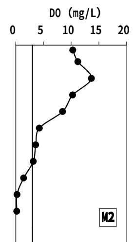
三高貯水池における DO 分布図 (平成17年8月4日, 11日, 19日, 29日, 9月16日, 22日)
