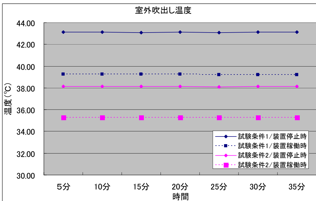
図 4 - 1 室外機吹出空気温度変化
