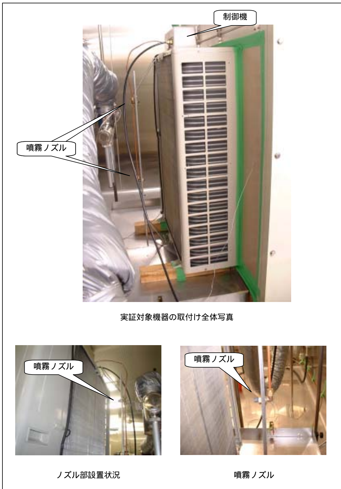
図 1 - 2 実証対象機器の設置状況
