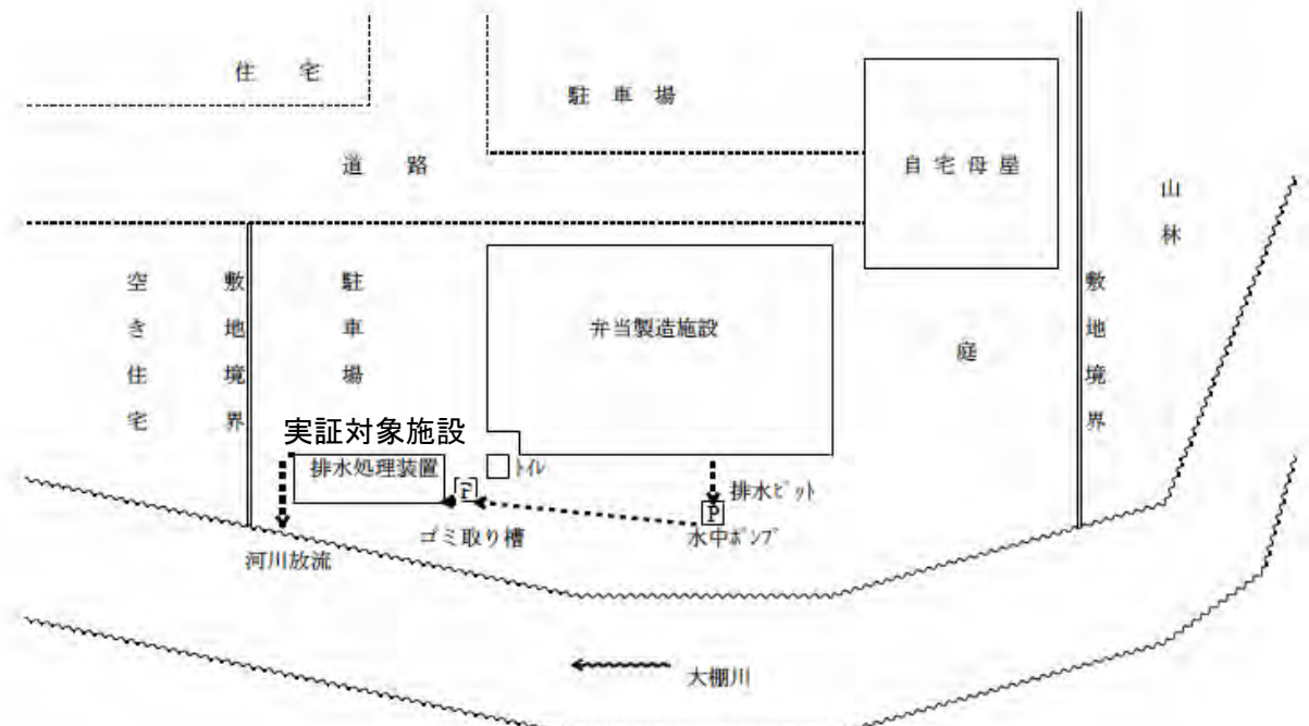
図1-1 処理装置配置図
