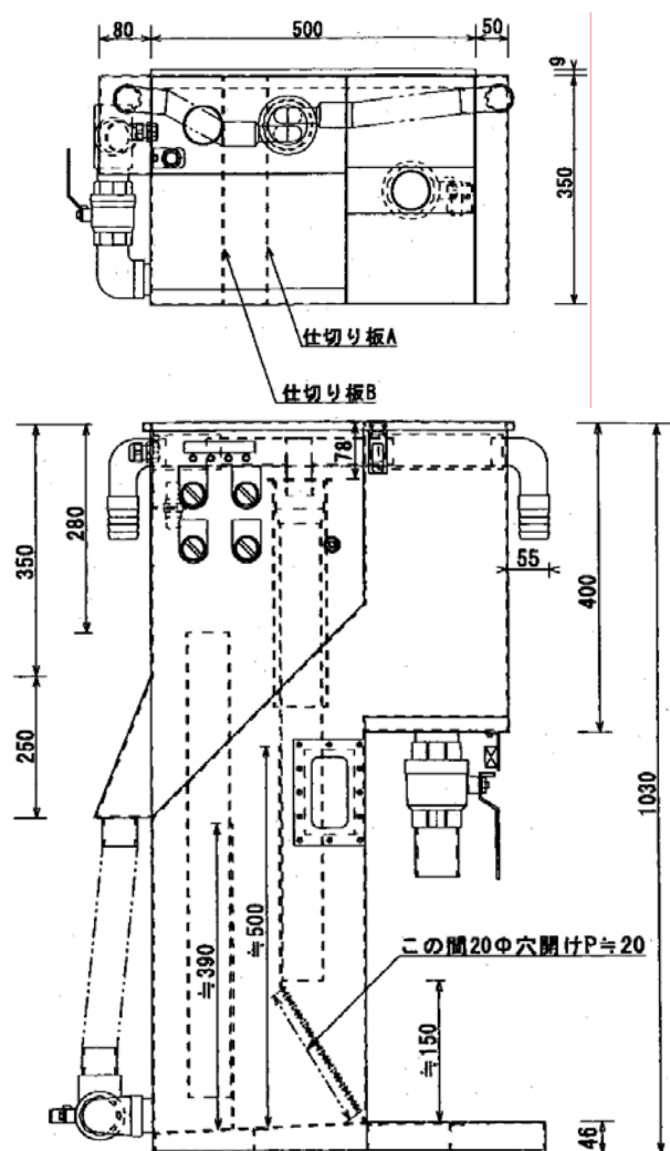
図1 - 2 実証対象機器の外観及び構造図
