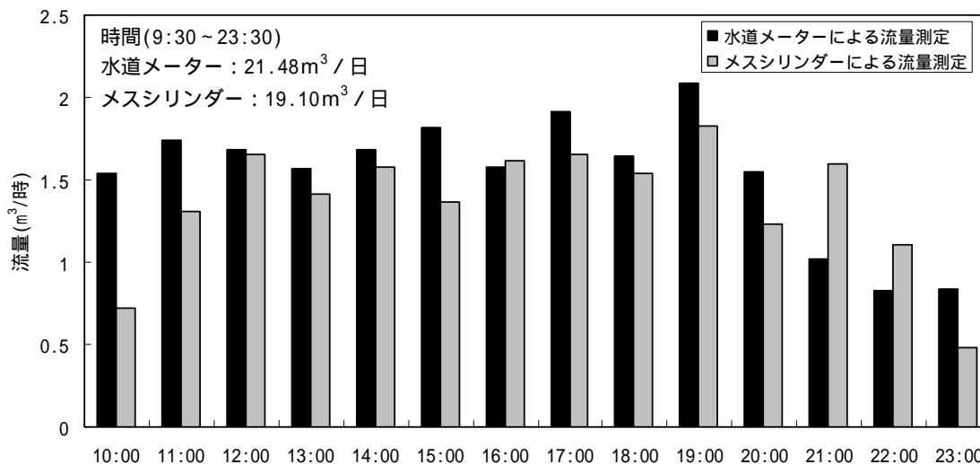
図4-3 日間水質試験における流量変動
