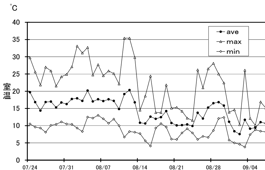
図6-5 室内温度
