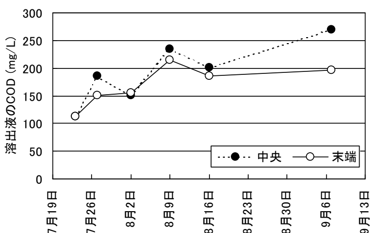
図6-18 CODの推移
