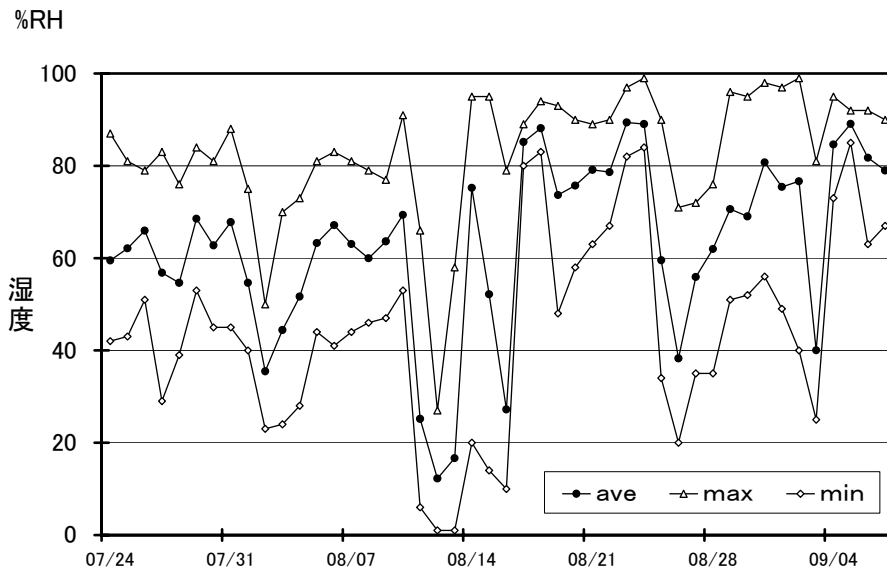
图6-6 室内湿度
