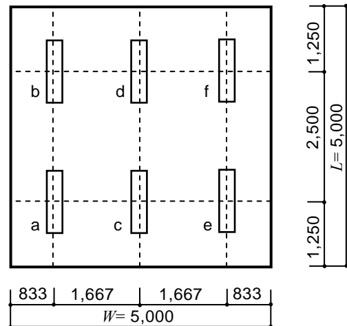
図 3 照明器具配置
