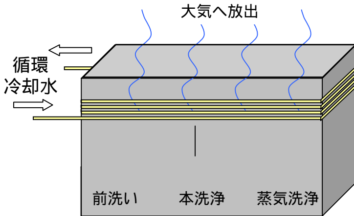
3槽式ジクロロメタン洗浄槽
