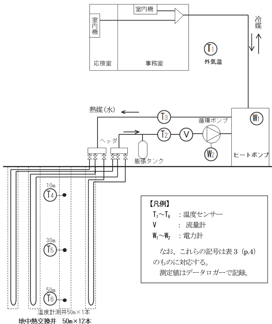
図 1 実証対象技術の概要
