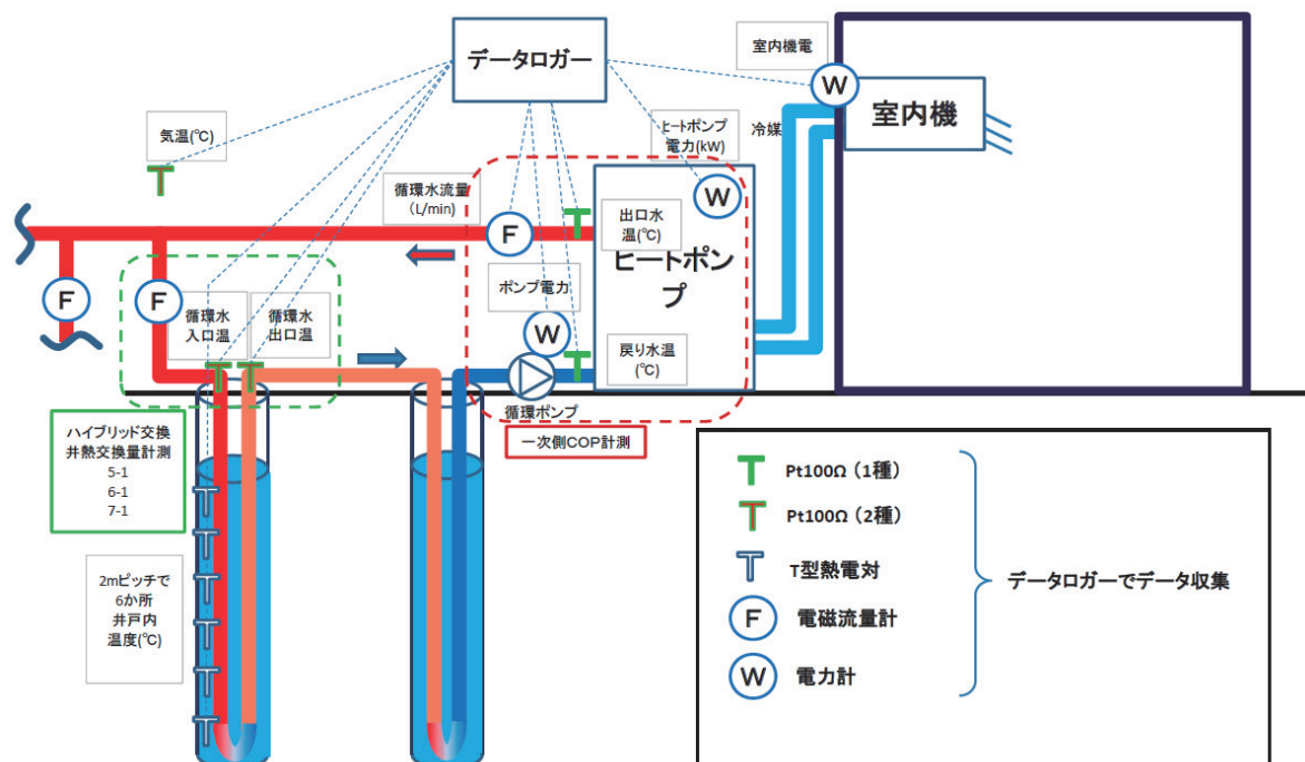
図3 実証対象技術の全体概要
