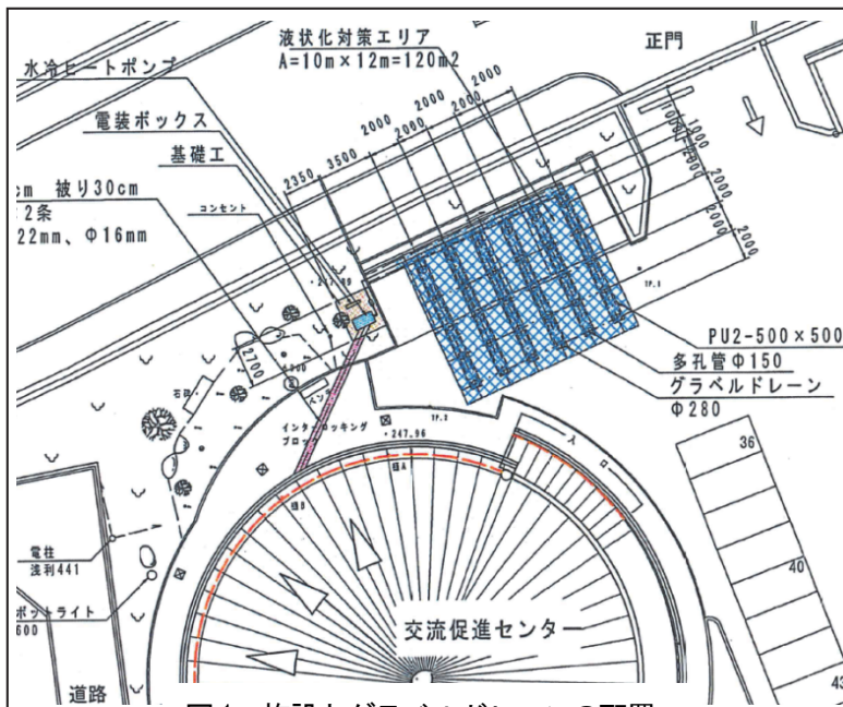
図1 施設とグラベルドレーンの配置
