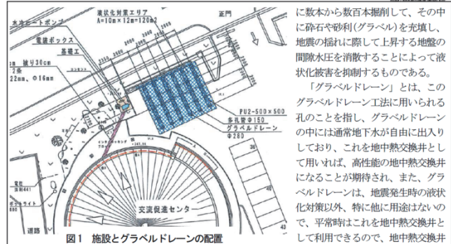
図1 施設とグラベルドレーンの配置
