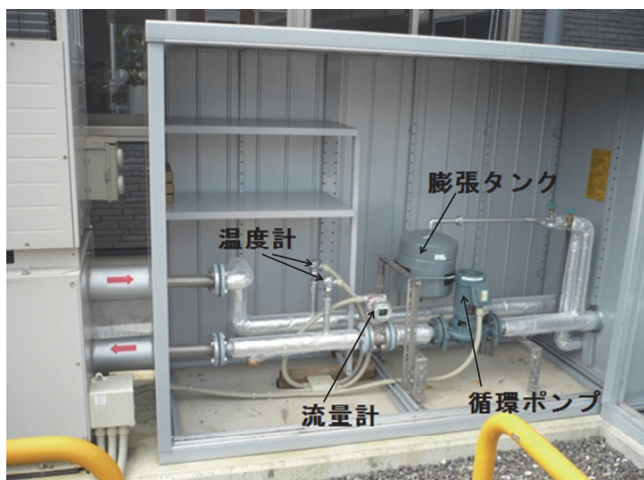
写真2 循環ポンプ、計測器等
