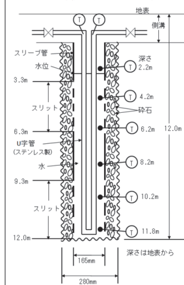
図2 地中熱交換井の構造概要
