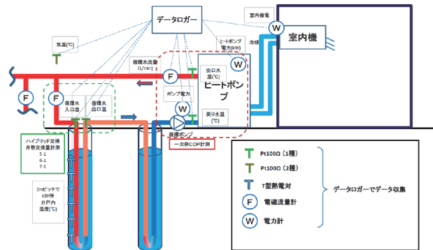
図3 実証対象技術の全体概要
