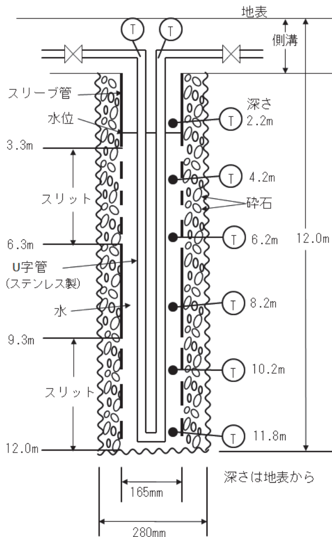
図2 地中熱交換井の構造概要
