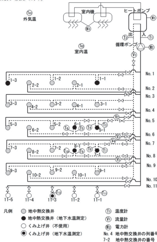
図4 実証試験実施設備と計測器の配置
