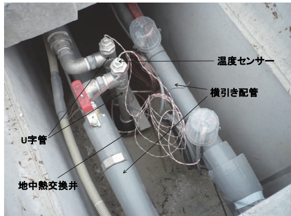
写真3 地中熱交換井の口元
