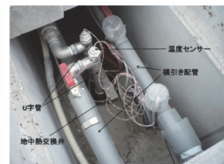
写真3 地中熱交換井の口元
