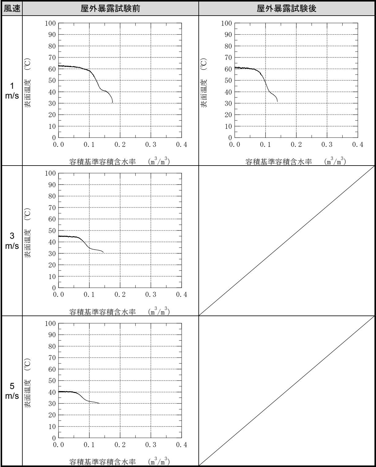
⑧ 表面温度と含水率の関係
