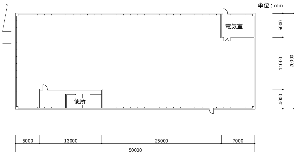
図 4-2 計算用工場モデル（平面図）
