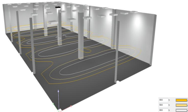
図 4 計算結果 - 作業面の照度分布（例）
