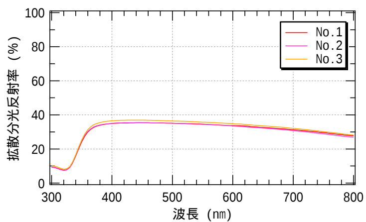
図-1 拡散分光反射率測定結果
