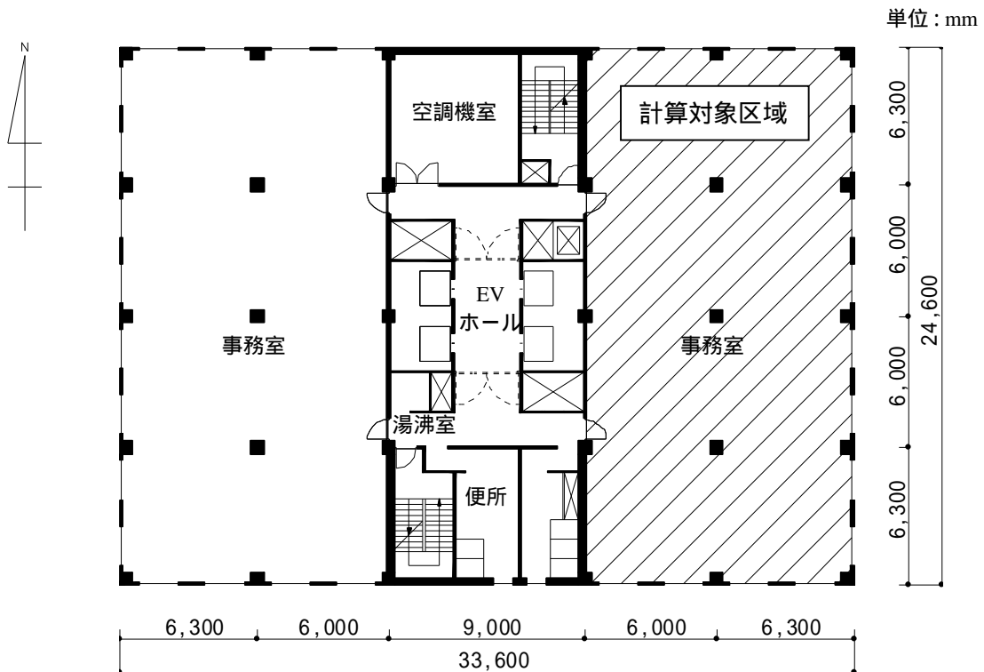
図 4-1 計算用オフィスモデル(平面図)
