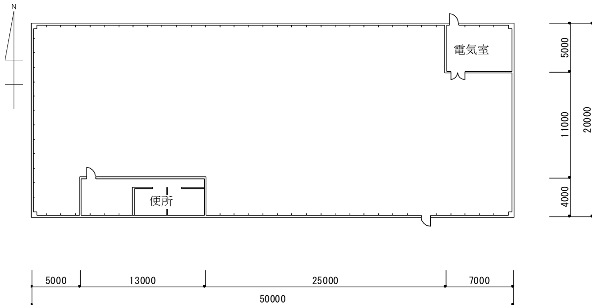
図 7 計算用工場モデル（平面図）
