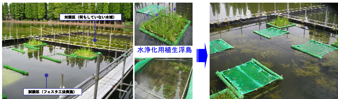
植生浮島により、短い期間で透明度が改善された水域（設置約1週間後） 沈水植物再生用浮島 沈水植物が再生され、水質が安定化した水域（設置約10ヵ月後）
