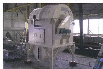
エスローテ0.5型沈殿槽付(フィリピン向け)
