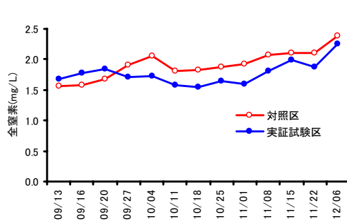
図6 実証試験区と対照区の全窒素の経時変化
