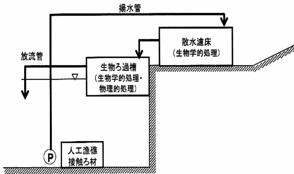
処理フロー図
