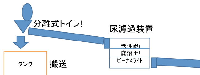
図2 現地浄化型簡易し尿処理
