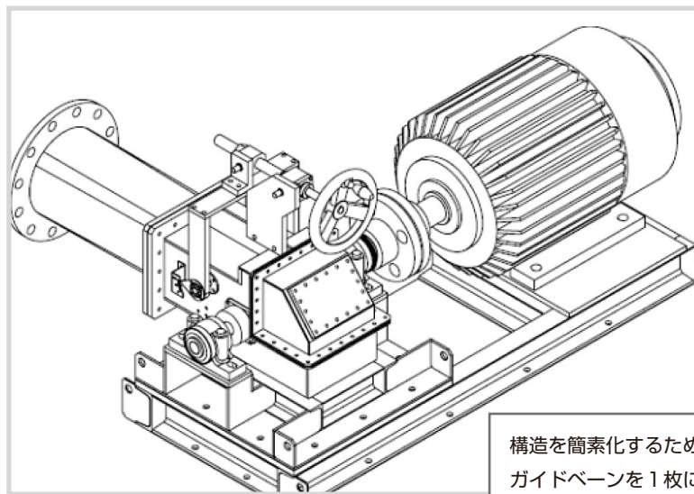
図1 水車外形図
