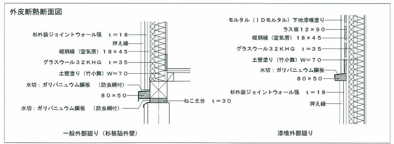
外壁詳細図 1:30
