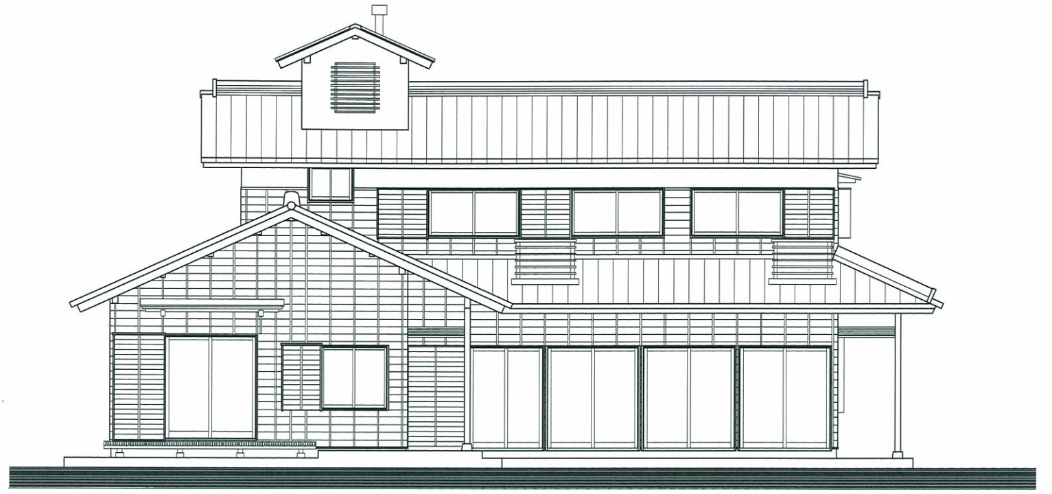
南立面図 1 : 100
