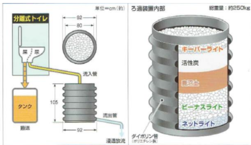
図 し尿分離式トイレ（モンライト）による処理の概要
