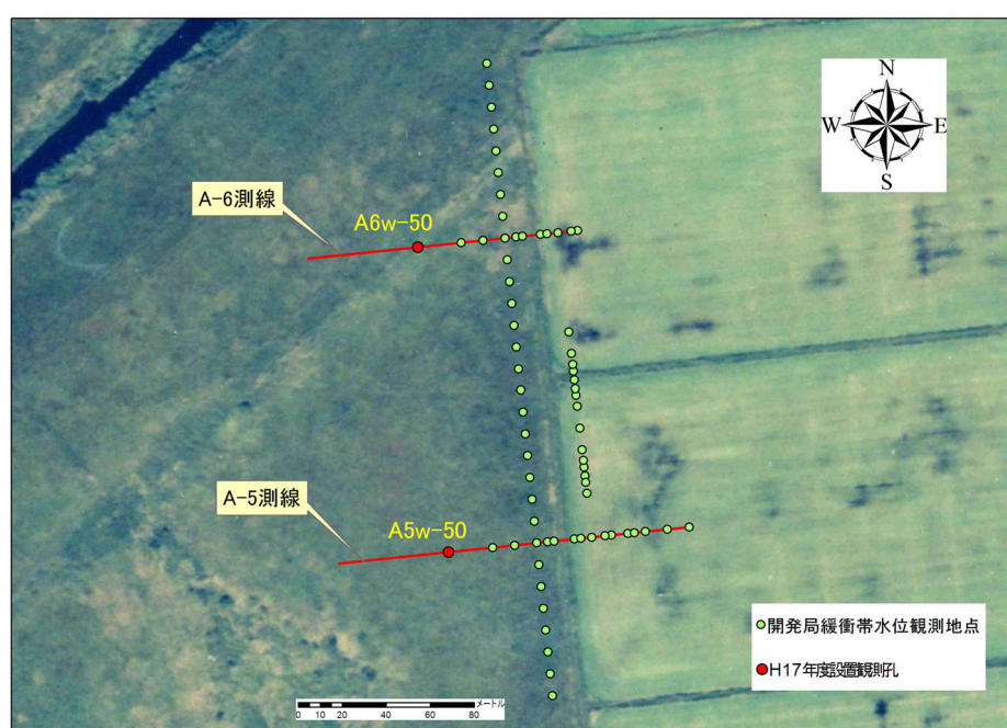
図 4.1.2 A-5 および A-6 測線の観測孔配置図
