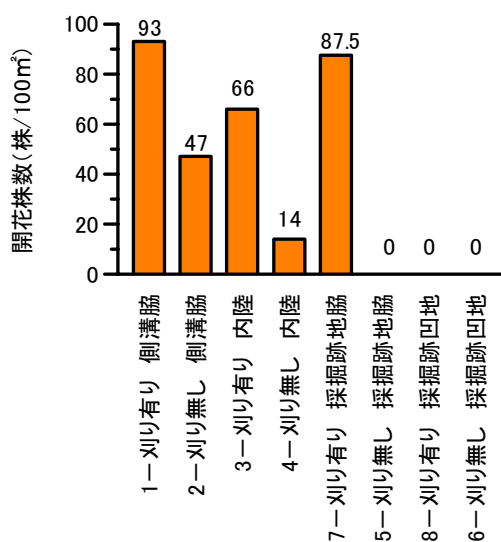
図 3.3.27 原生花園におけるエゾカンゾウ開花株数
