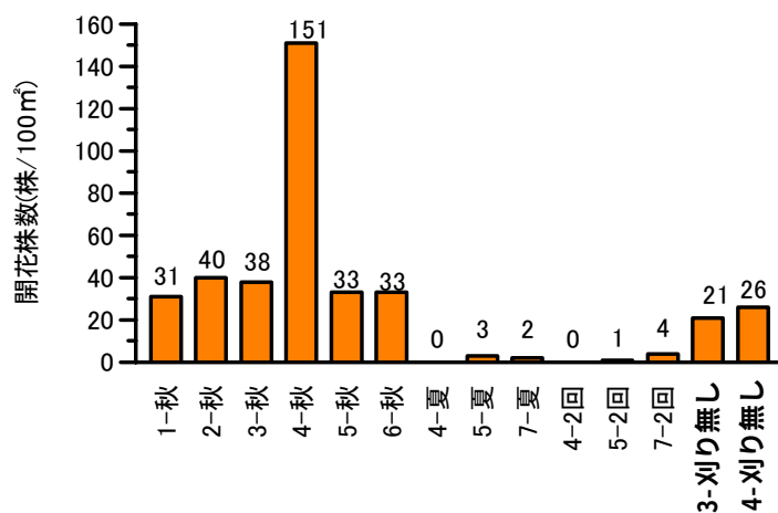
図 3.3.26 丸山におけるエゾカンゾウの開花株数
