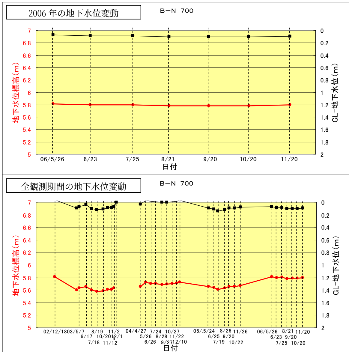
図 5.1.8 ゾーン⑤ (B-N 700 地点) の地下水位変動図
