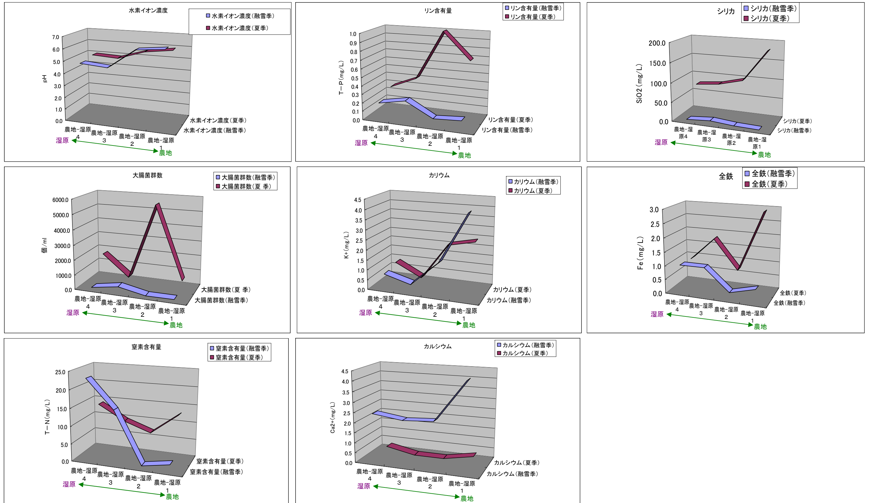
図 3.3.11 泥炭採掘地一隣接農地測線に沿った代表的な分析結果の比較図
