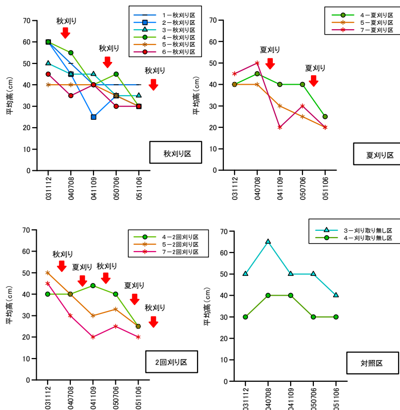
図 4.2.3 円山周辺におけるササ平均高の推移
