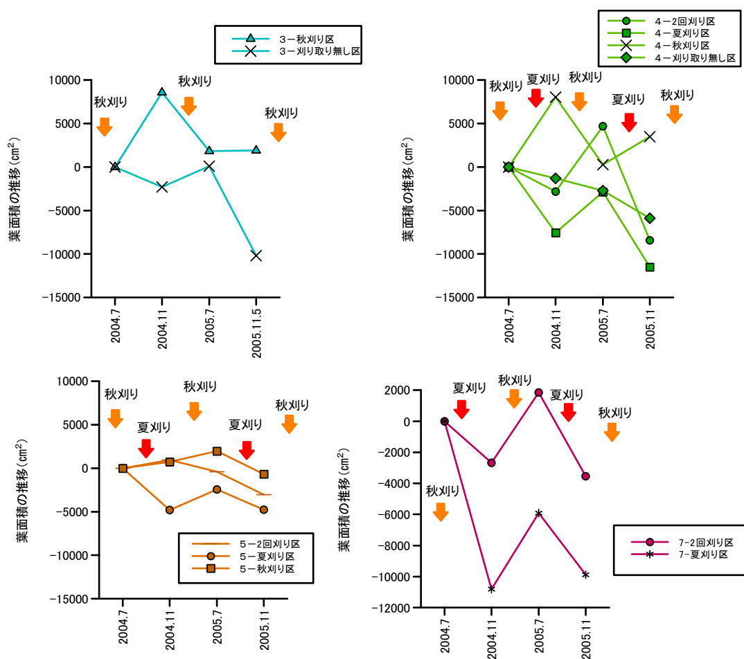
図 4.3.11 円山周辺における地点別葉面積の推移
