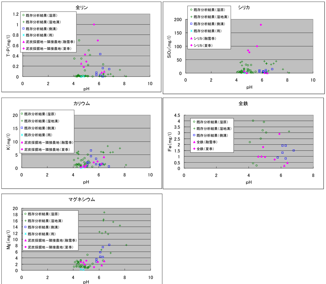
図 3.3.12 泥炭採掘地－隣接農地測線の水質分析結果と既存分析結果との比較
