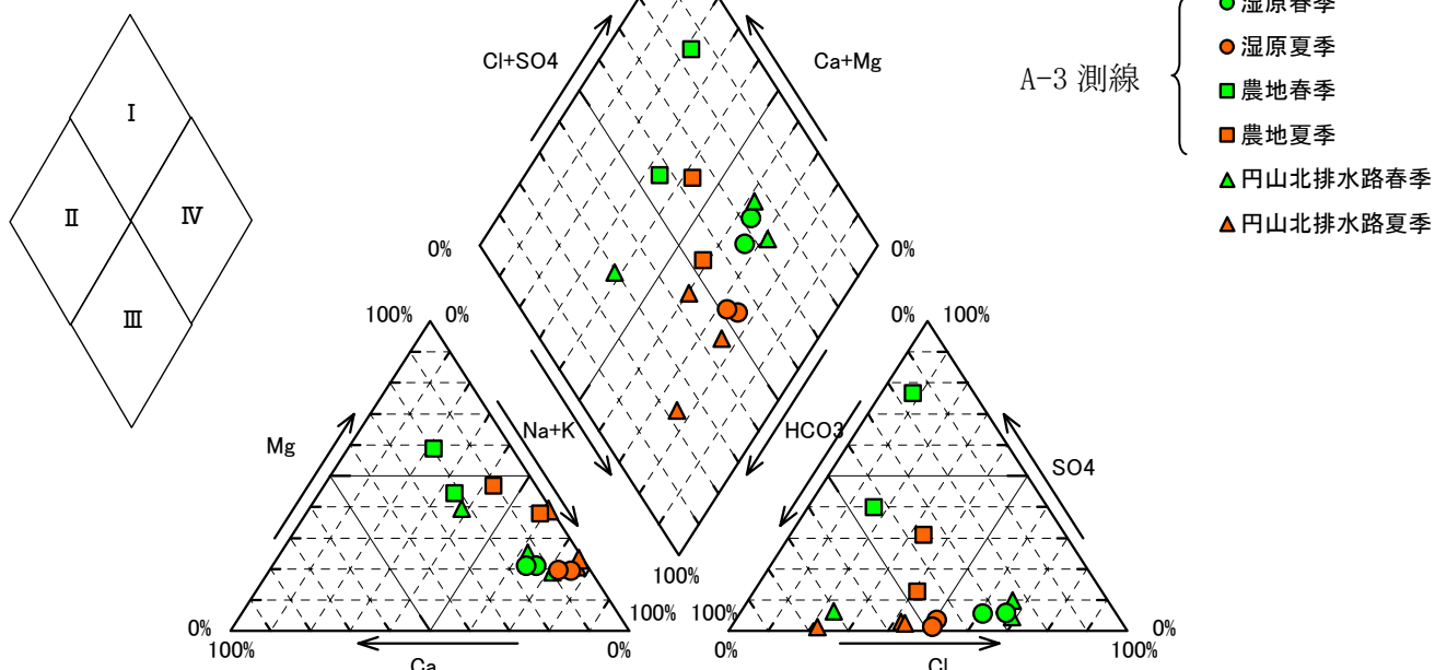
図 3.3.5 円山北部排水路及びA3測線の分析結果のトリリニアードイヤグラム
