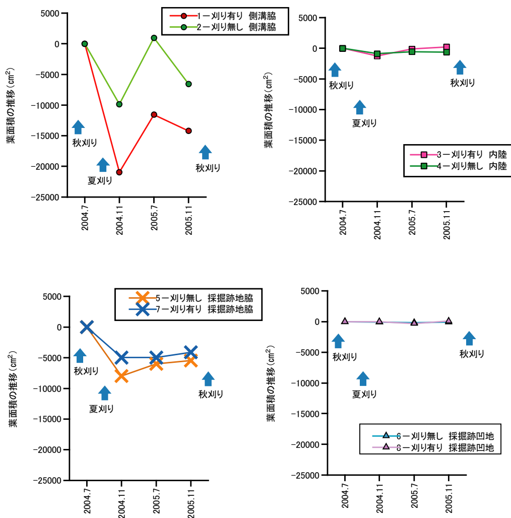
図 4.3.12 原生花園における地点別 1 m² 当り葉面積の推移
