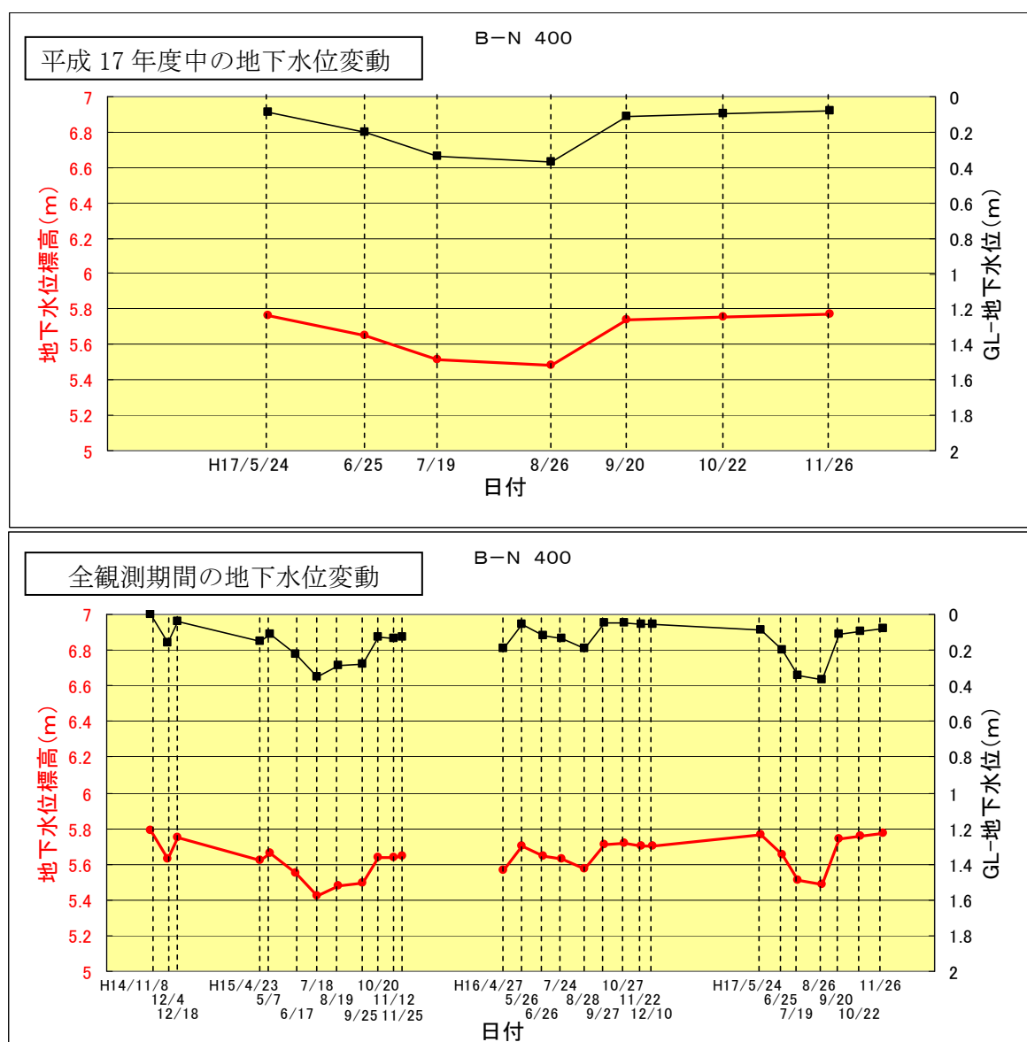
図 2.6.7 ゾーン④（B-N 400地点）の地下水位変動図
