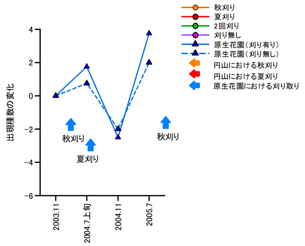
図 4.3.14 原生花園における 出現種数の変化
