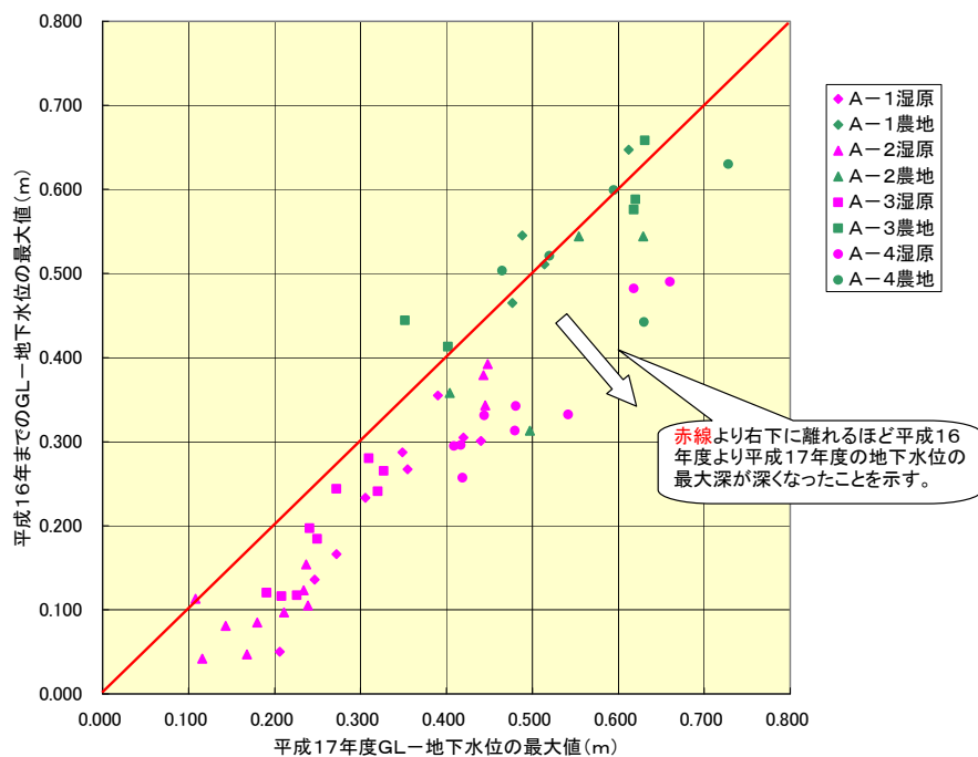
図 2.5.15 平成17年度と平成16年度の地下水位最深値の相関図
