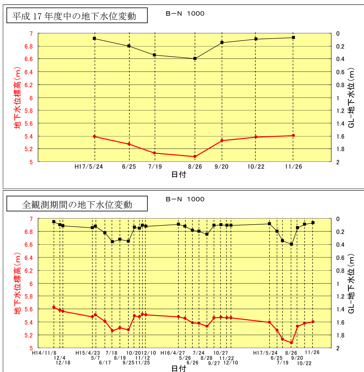
図 2.6.10 ゾーン⑥（B-N 1000地点）の地下水位変動図
