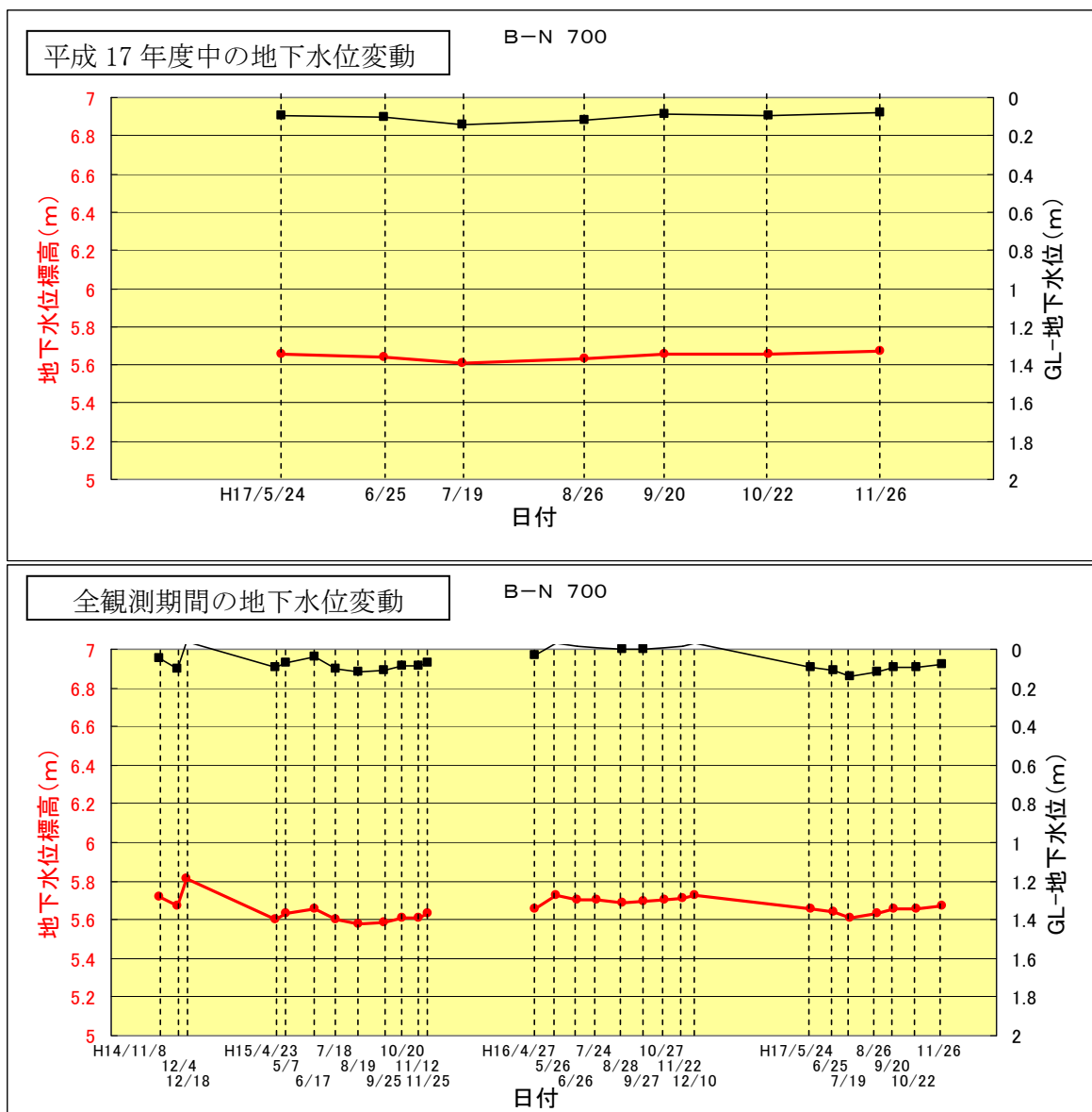
図 2.6.9 ゾーン⑤ (B-N 700 地点) の地下水位変動図
