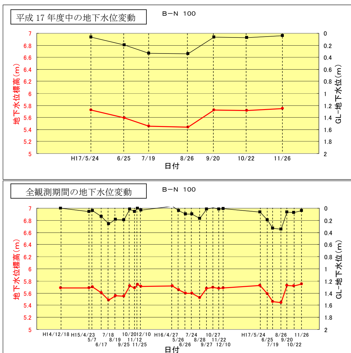
図2.6.6 ゾーン③（B-N 100地点）の地下水位変動図
