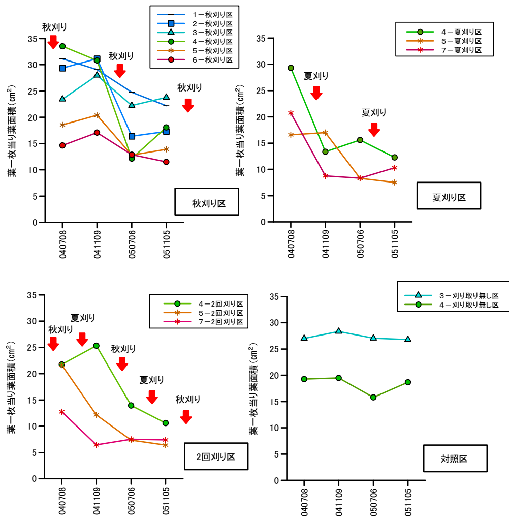
図 4.2.8 円山周辺におけるササの葉 1 枚当りの葉面積
