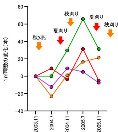
図 4.3.3 円山周辺における刈り取り条件別 1 m 2 当りササ稈数の推移
