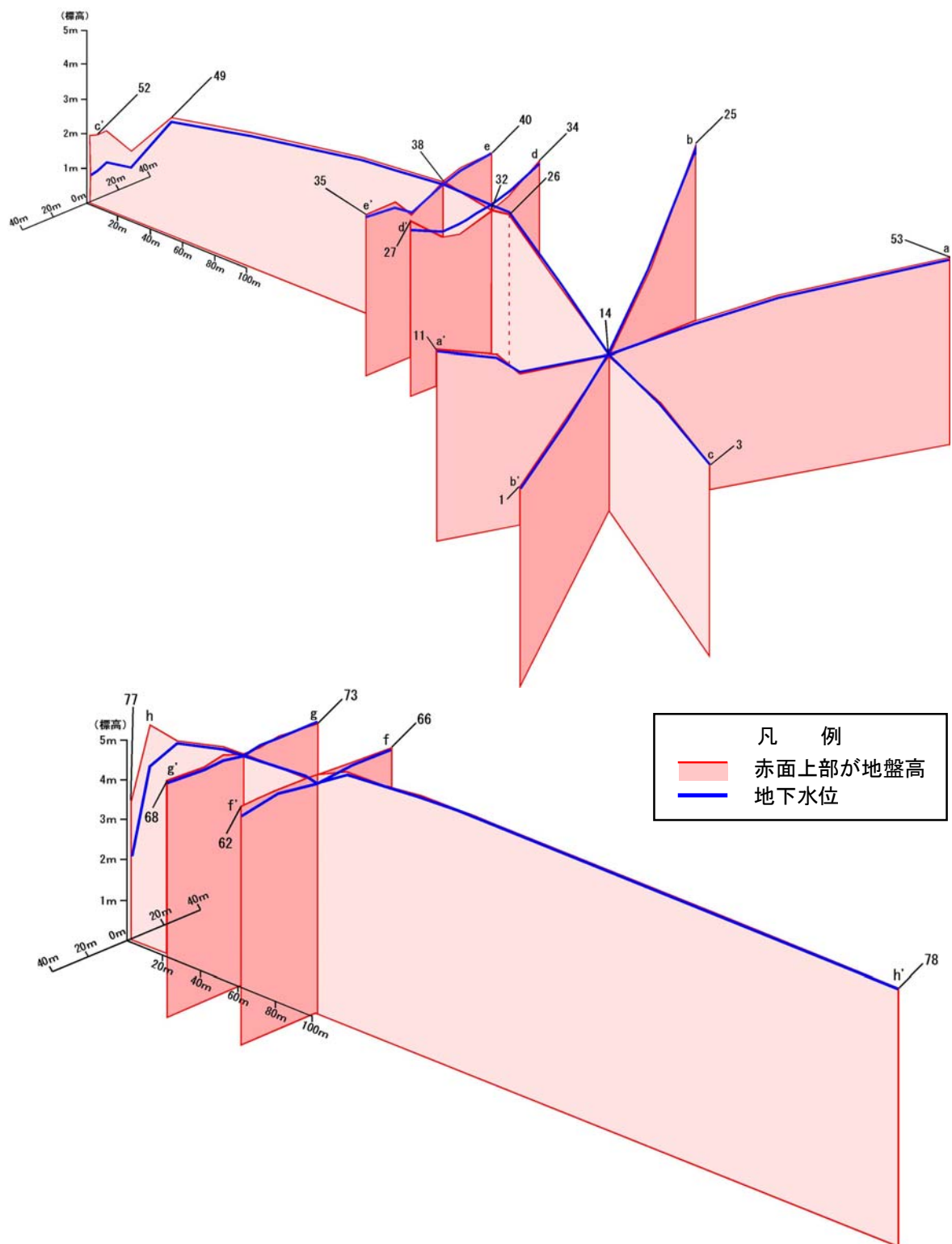
図 2.8.15 水抜き水路 1・2 地点の地下水断面ブロックダイヤグラム (平成 17 年 11 月 26 日地下水位)
