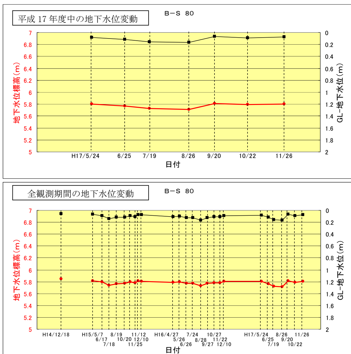
図 2.6.5 ゾーン②（B-S 80地点）の地下水位変動図
