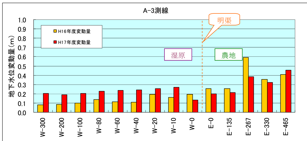
図 2.5.12 A－3 測線における平成 16 年度と平成 17 年度の変動量の比較
