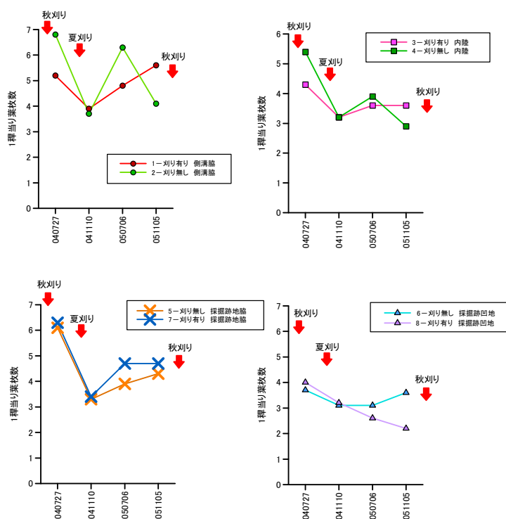
図 4. 2. 15 原生花園におけるササ 1 稈あたりの葉の枚数の推移
