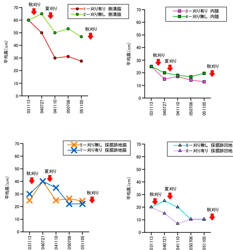
図 4.2.12 原生花園におけるササ平均高の推移
