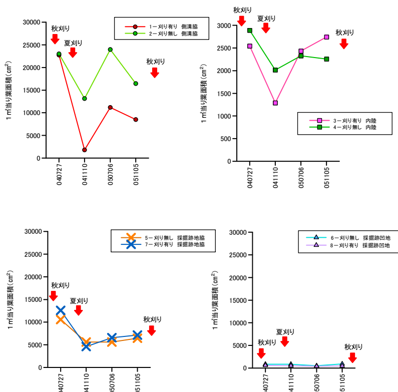
図 4. 2. 17 原生花園における 1 m 2 当りササ葉面積の変化
