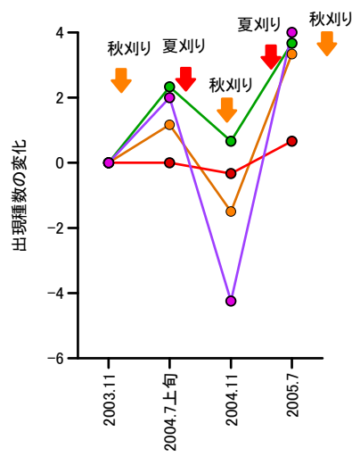
図 4.3.13 円山における刈り取り条件別 出現種数の変化
