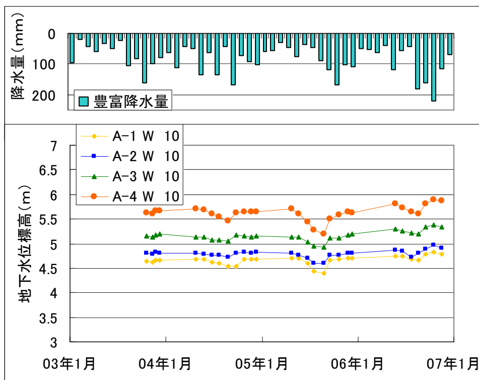
図 4.3.11 各測線 W 10m地点地下水位変動
