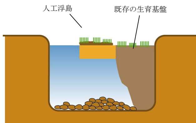
図 10.3.7 人工浮島設置イメージ
