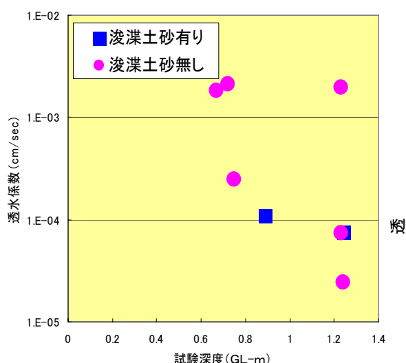
図 7.2.24 試験深度と透水係数の関係
