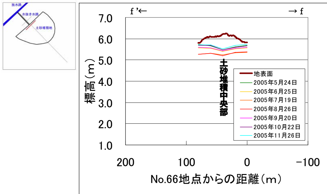
図 7.2.10 水抜き水路 2 f-f' 断面における地下水位分布
