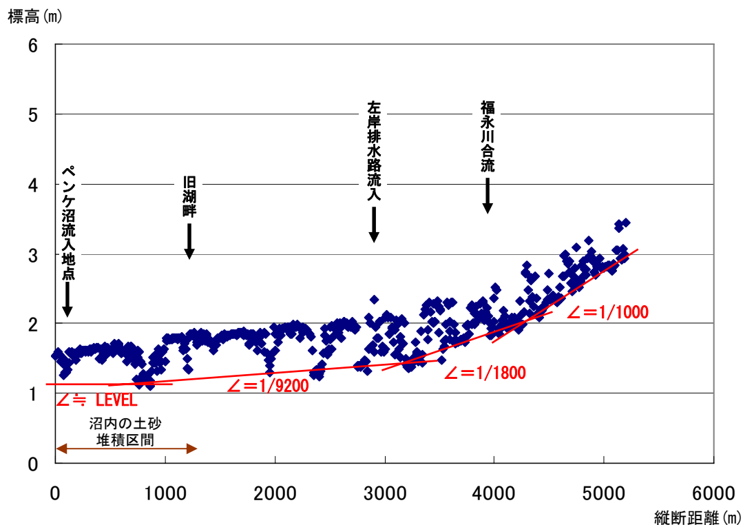
図 9.2.2 下エベコロベツ川の縦断標高分布
