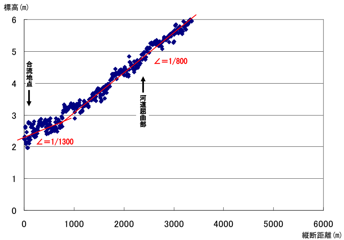
図 9. 2. 3 福永川の縦断標高分布
