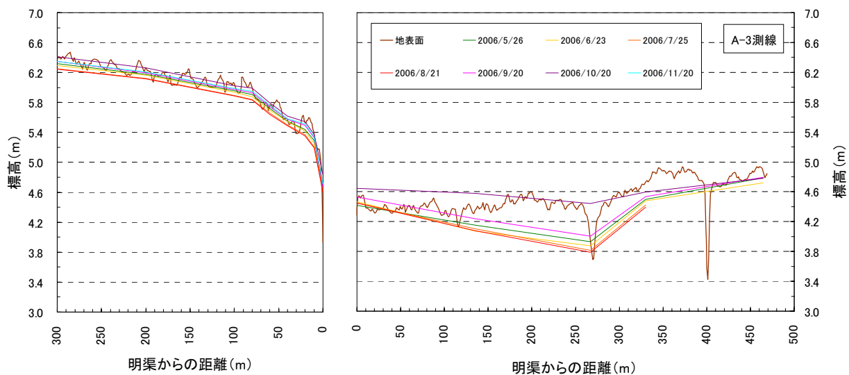
図 4.3.6 A－3 測線の地形と地下水位分布（2006 年）
