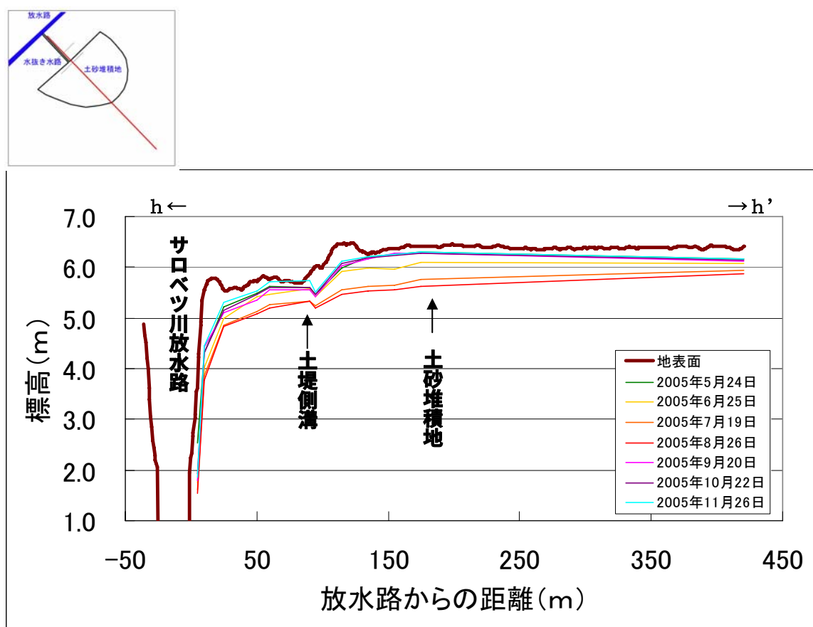
図 7.2.12 水抜き水路 2 h-h' 断面における地下水位分布
