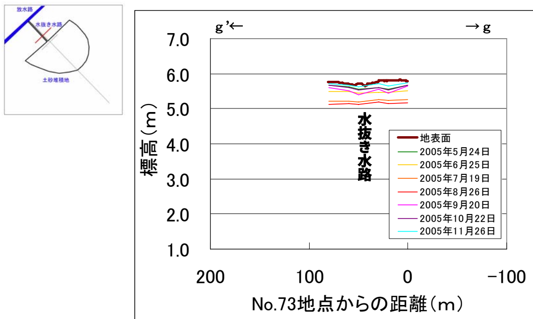
図 7.2.11 水抜き水路 2 g-g' 断面における地下水位分布
