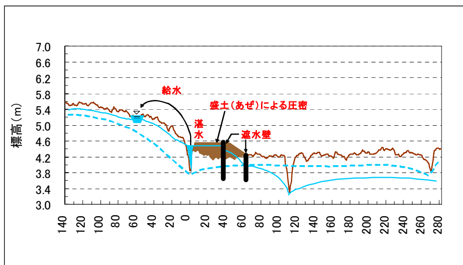
図 8.3.3(1) 緩衝帯の整備イメージ
