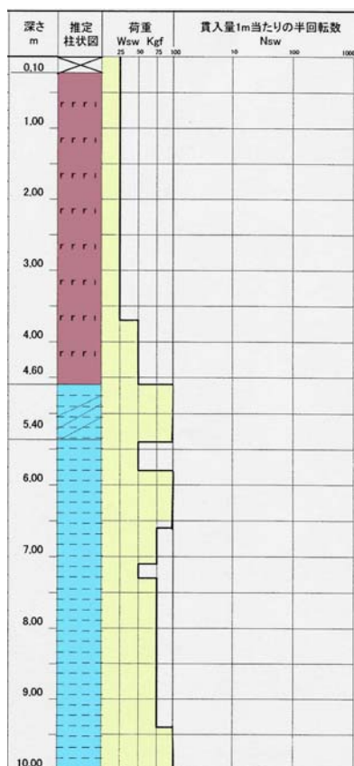
図 7.3.9 堰上げ試験候補地①における スウェーデン式サウンディング結果
