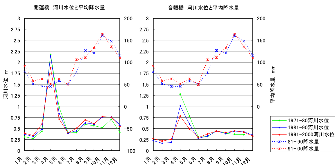
図 3.4.5 開運橋、音類橋における河川水位の変遷 (降水量は豊富の値)
