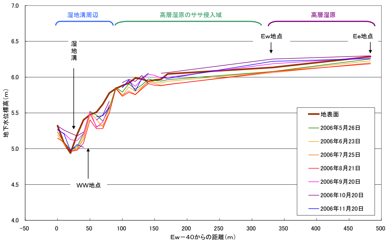
図 4.3.29 2006 年の E 測線の地下水位分布
