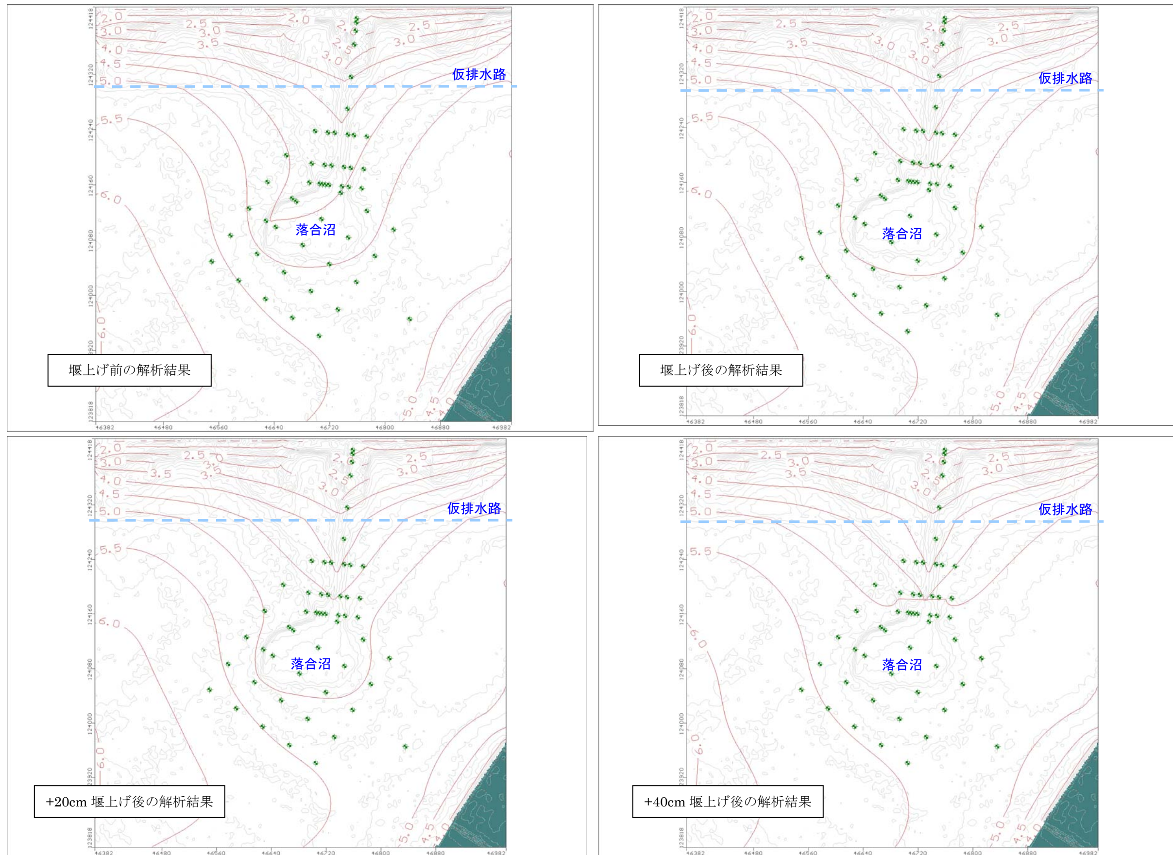
図 7.5.20 地下水流動解析による水抜き水路 1 実証試験地の堰上げ前後の地下水位等高線の予測図
