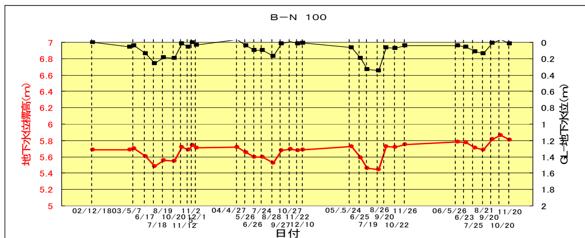
図 4.3.18 ゾーン③（B-N 100地点）の地下水位変動図
