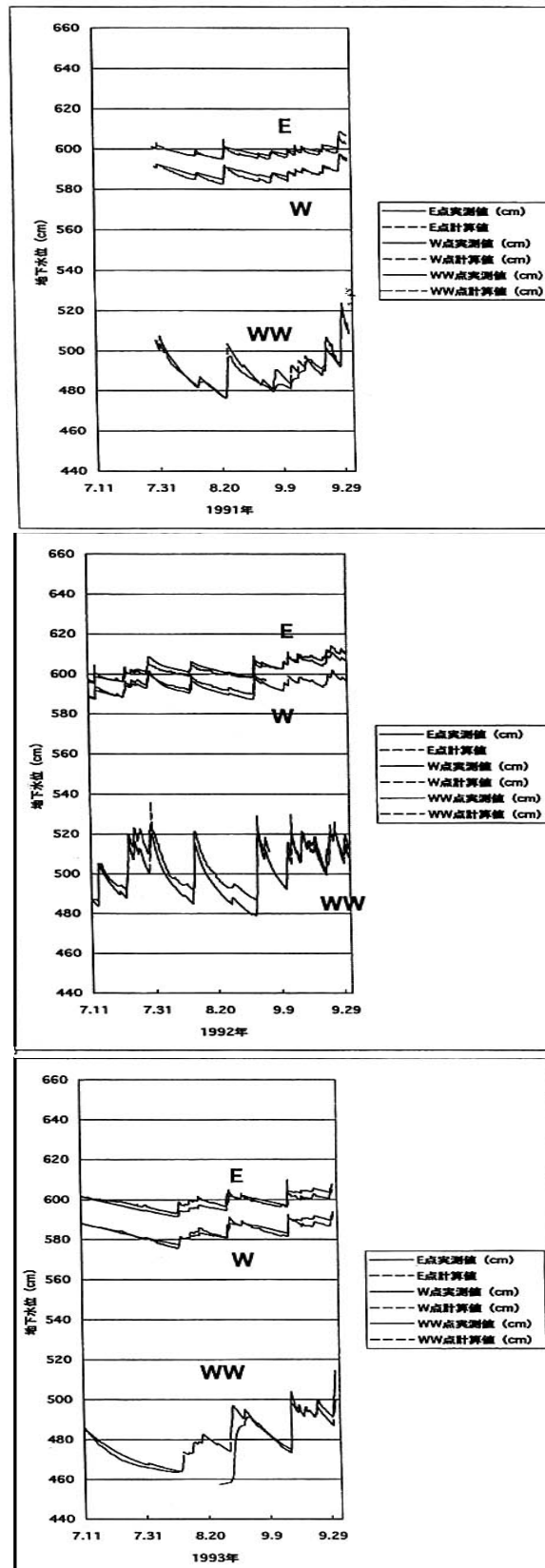
图 6.2.13 地下水位观测结果
