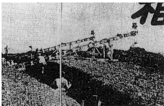
図 3.1.5 仮水路（仮排水路）の掘削状況
