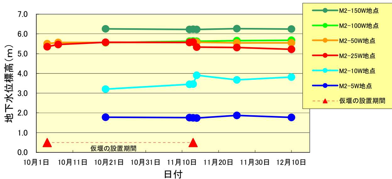
図 7.3.5 10月4日～12月10日までの各地点の地下水位の変化グラフ
