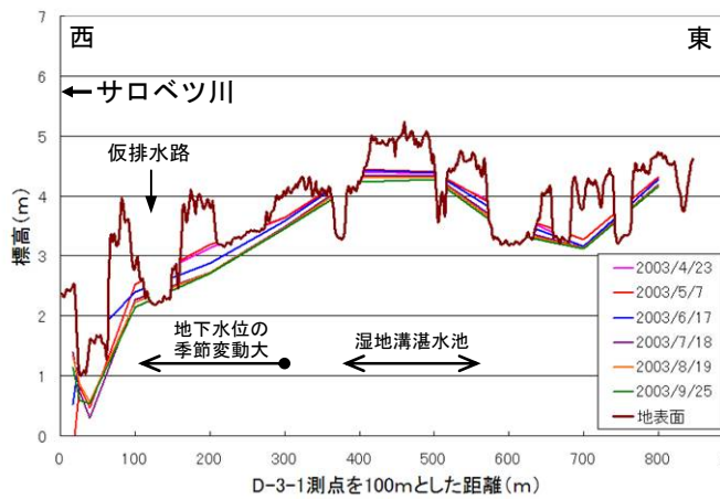
図 5.2.15 D-3 測線の地下水位分布
