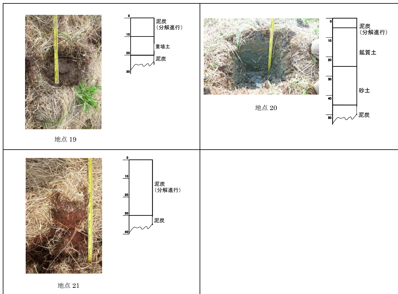
図 7.2.19 (4) 土壌断面結果
