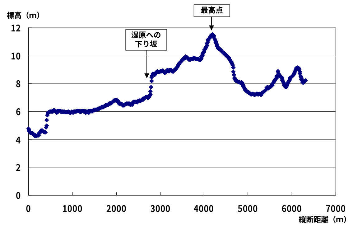
図 6.2.18 レーザー計測データから読み取った円山道路の縦断標高
