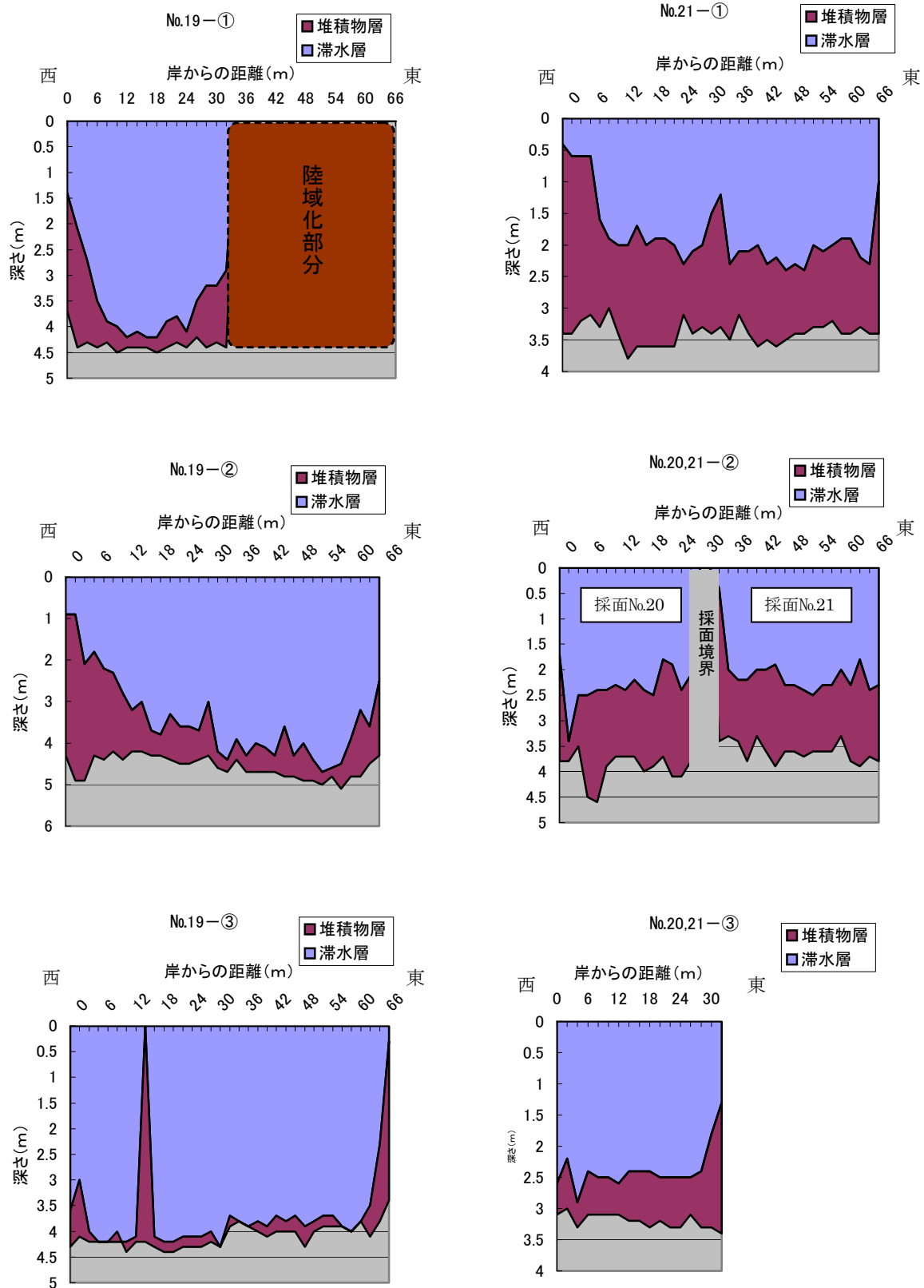
図 10.3.11 横断測線における地形・ブロック状泥炭堆積計測結果
