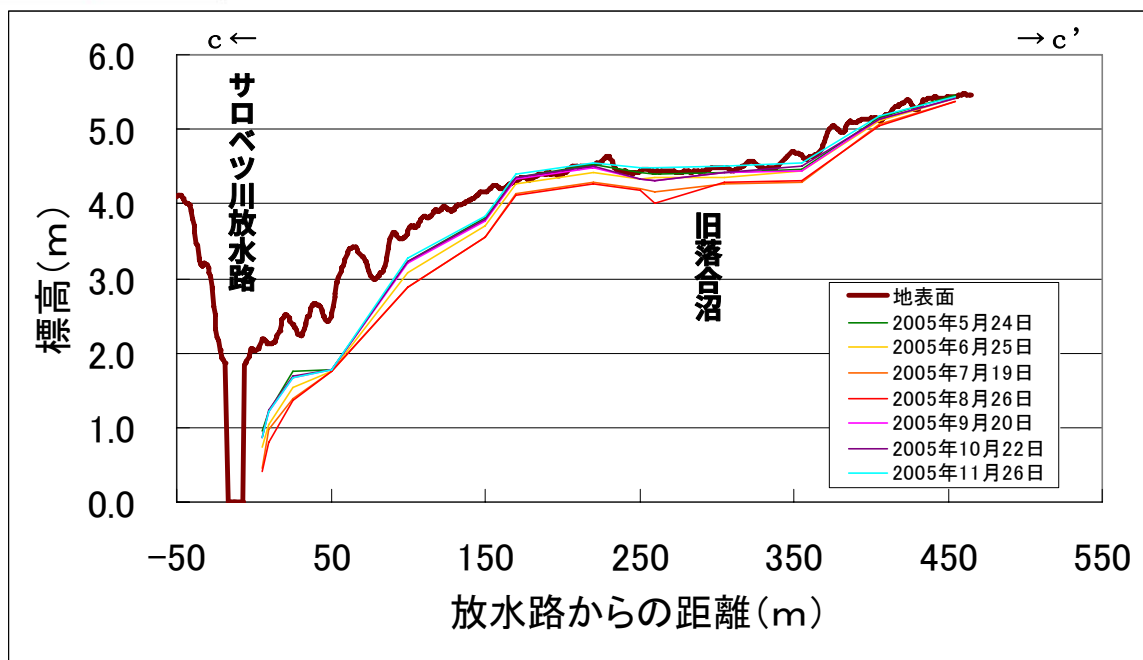
図 7.2.6 水抜き水路 1 c-c' 断面における地下水位分布
