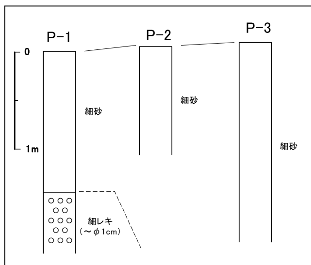
図 9. 1. 20 自然堤防部の断面観察結果
