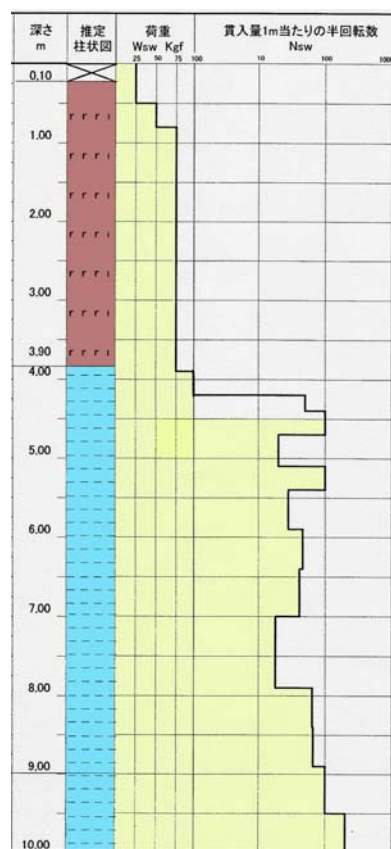
図 7.3.10 堰上げ試験候補地②における スウェーデン式サウンディング結果
