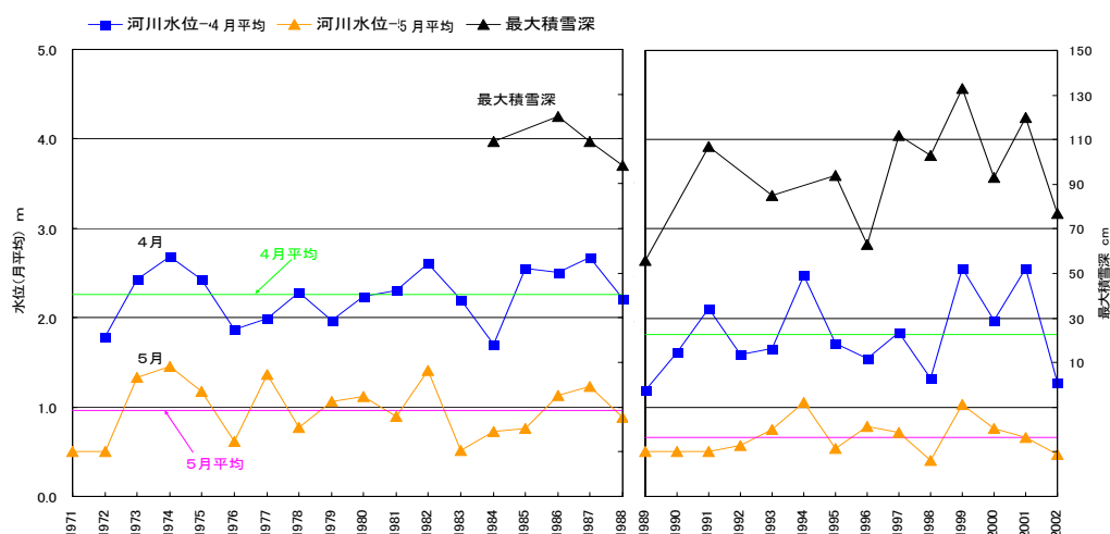
図 3.4.2 河川水位の変遷（開運橋）
