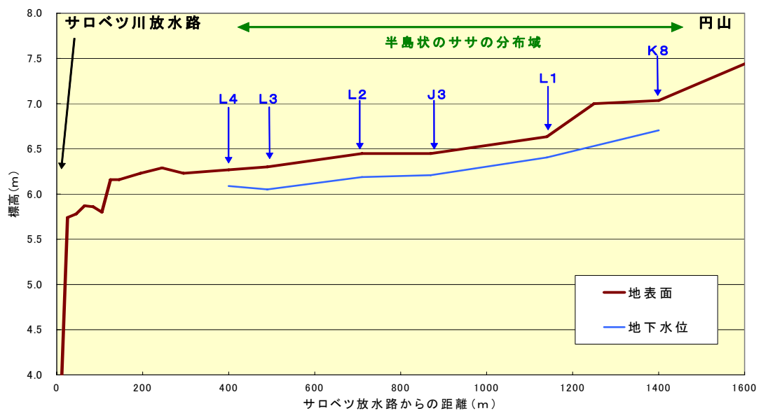
図 5.2.7 丸山からサロベツ川放水路に至る断面の地下水位分布
