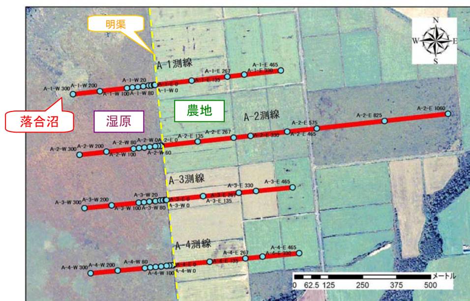
図 4.3.2 A測線における地下水位観測測線と観測孔位置
