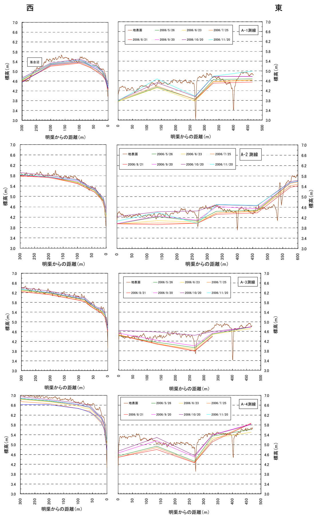
図 8.2.5 A-1～A-4 測線における地下水位観測結果
