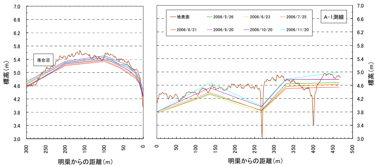
図 4.3.4 A－1 測線の地形と地下水位分布（2006 年）
