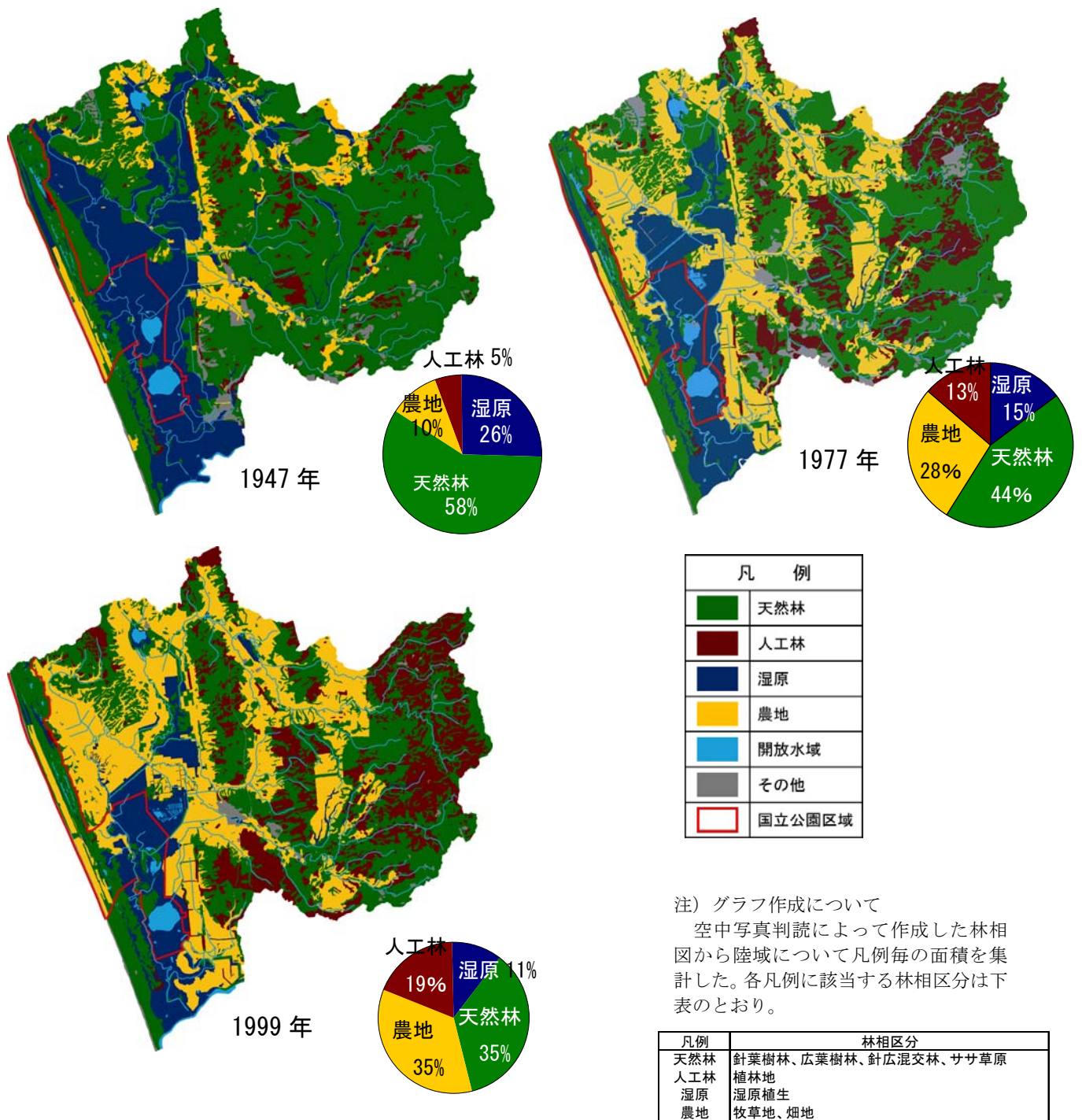
図 3.2.3 流域林相図
