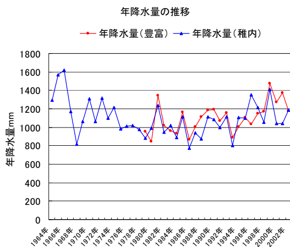
図 3.4.3 年降水量の変遷（豊富・稚内）
