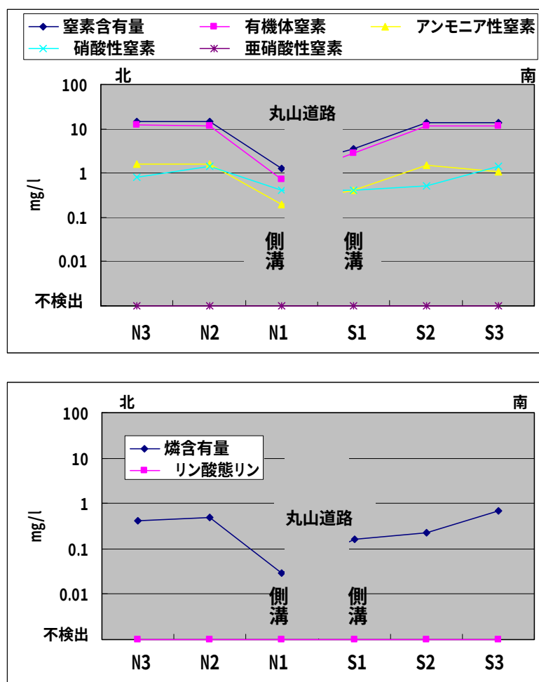
図 6.2.7 SP-2 測線方向の濃度分布（窒素・リン）
