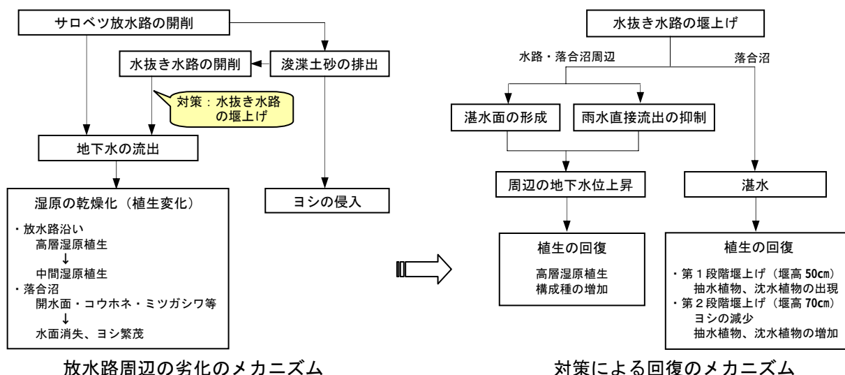
図 7.4.2 放水路周辺の劣化のメカニズムと対策による回復のメカニズム
