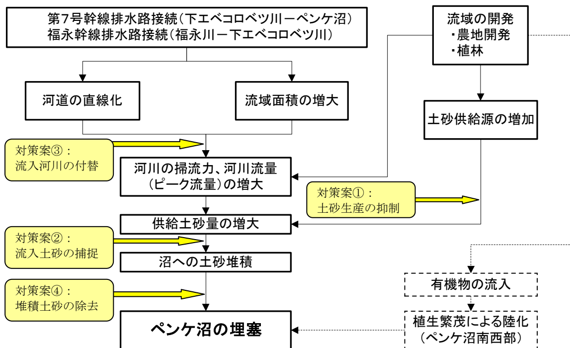
図 9. 2. 1 想定される劣化のメカニズムと対策案
