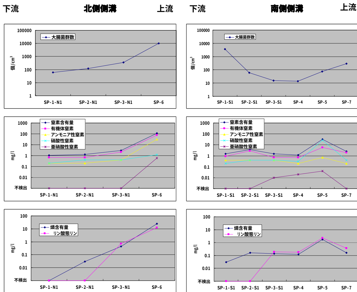
図 6.2.5 道路縦断方向の濃度分布
