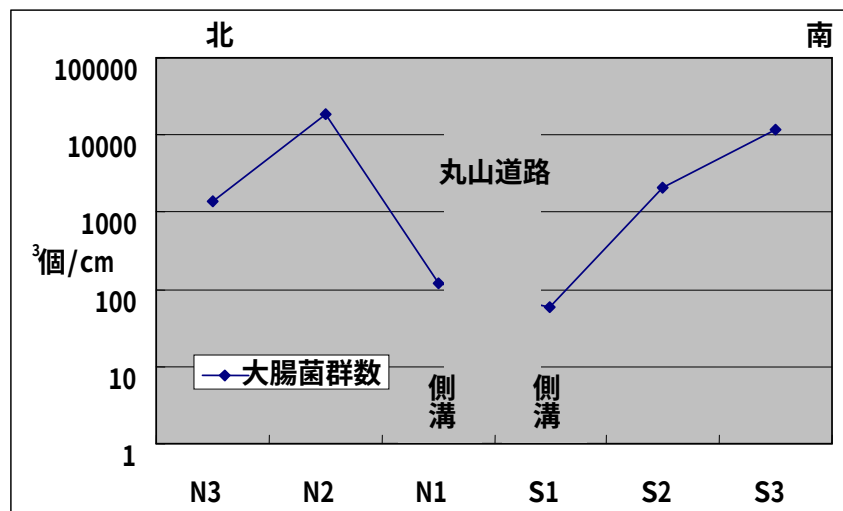
図 6.2.6 SP-2 測線方向の濃度分布（大腸菌群）
