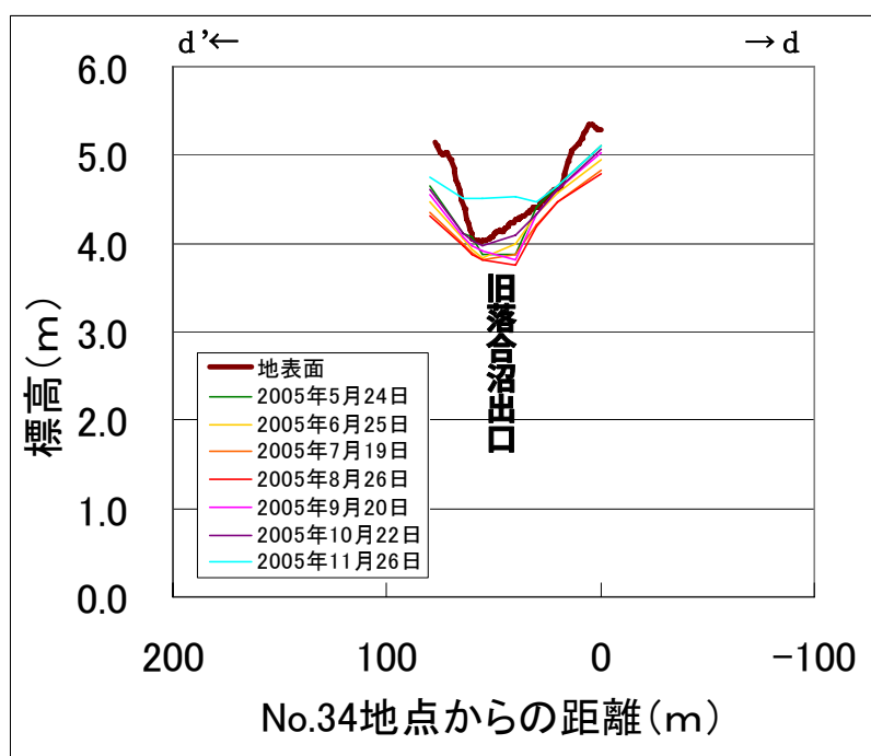
図 7.2.7 水抜き水路 1 d-d' 断面における地下水位分布
