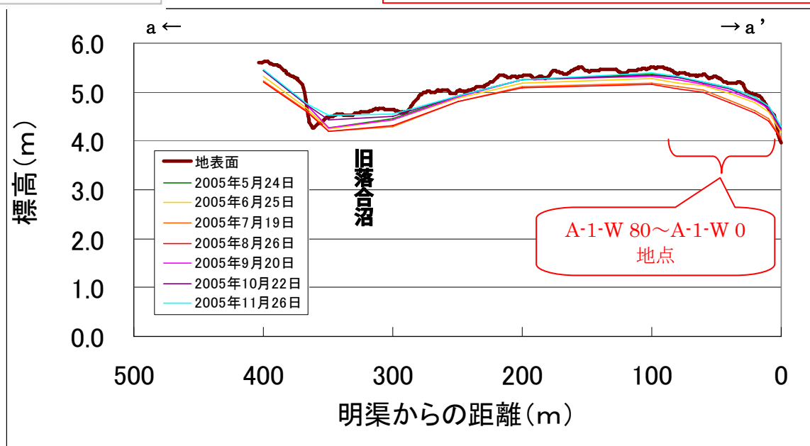
図 7.2.4 水抜き水路 1 a-a' 断面における地下水位分布
