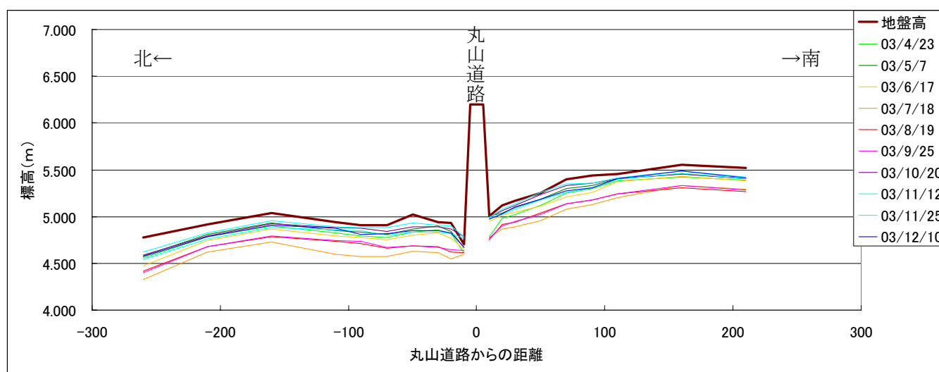
図 4.3.23 C測線の地下水位分布（2003 年）
