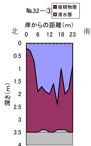
図 10.3.13 横断測線における地形・ブロック状泥炭堆積計測結果
