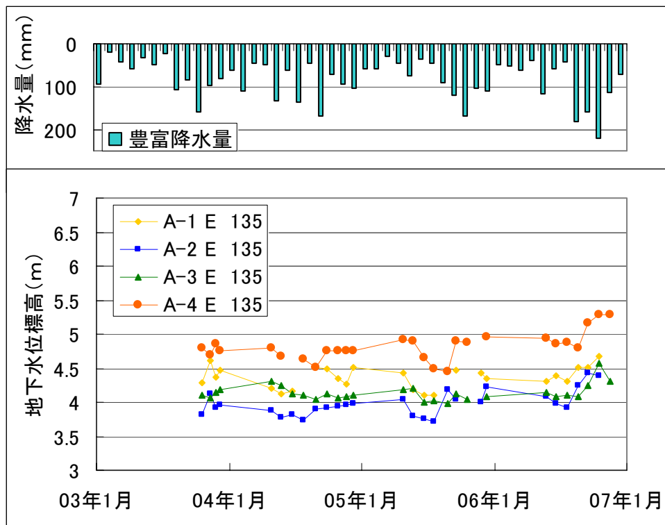
図 4.3.12 各測線 E 135m地点地下水位変動
