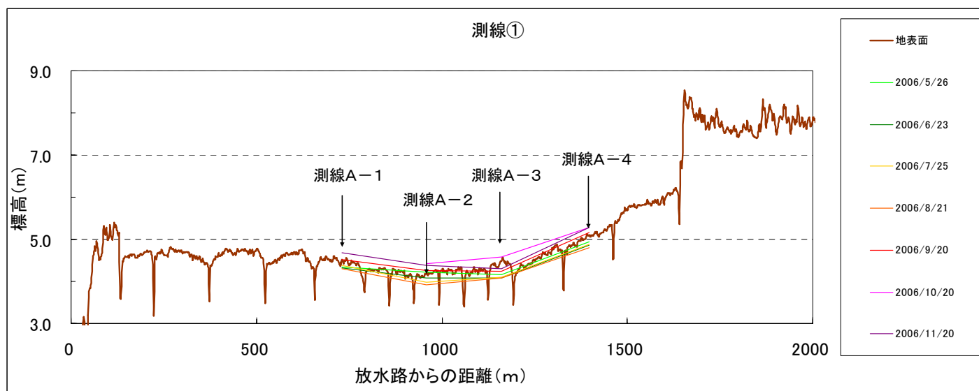
図 4.3.9 測線①における地形と地下水位分布（2006 年）
