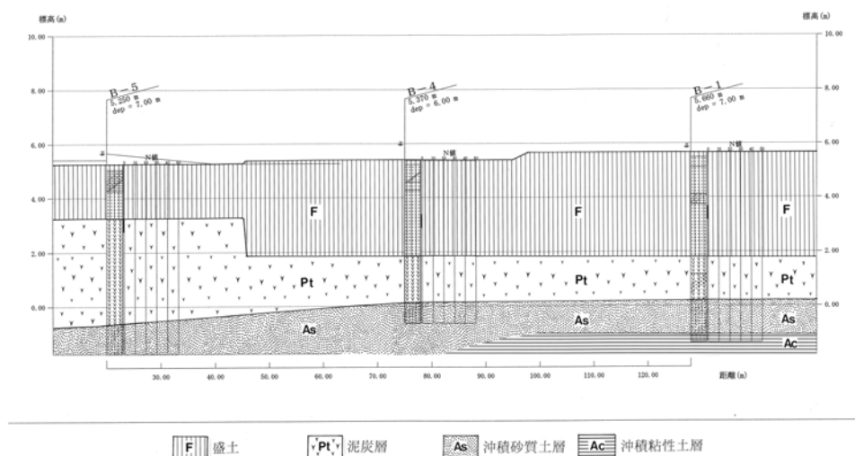
図 6.3.3 東西方向の土質断面図
