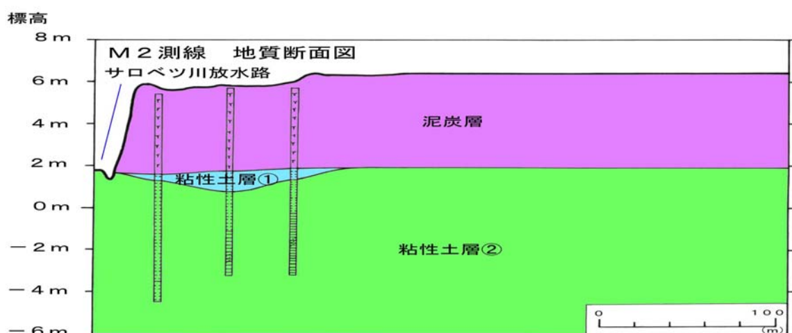
図 7.3.8 M2 測線の地質断面図
