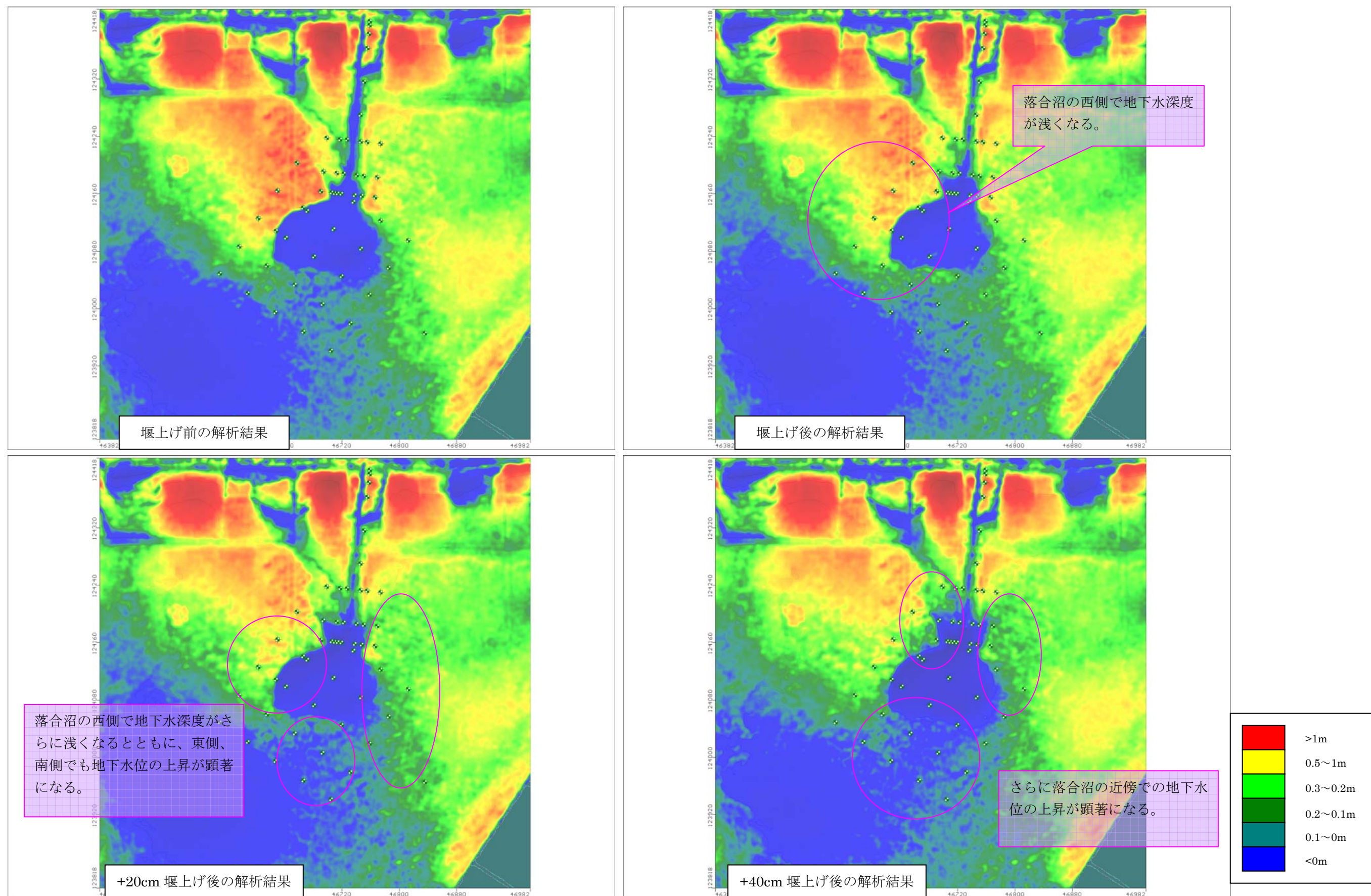
図 7.5.21 地下水流動解析による水抜き水路 1 実証試験地の堰上げ前後の地下水位深度の予測分布
