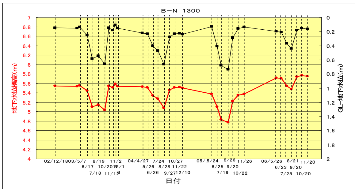
図 4.3.22 ゾーン⑦（B-N 1300地点）の地下水位変動
