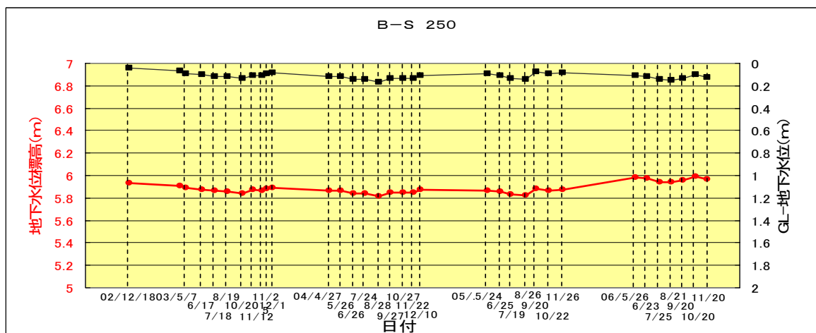
図 4.3.16 ゾーン①（B-S 250地点）の地下水位変動図
