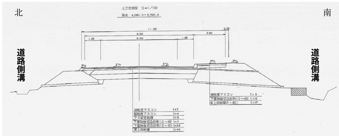
図 6.2.2 丸山道路盛土の標準断面（道路台帳より転載・加筆）
