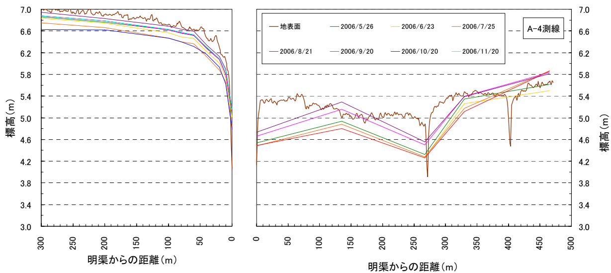
図 4.3.7 A－4 測線の地形と地下水位分布（2006 年）
