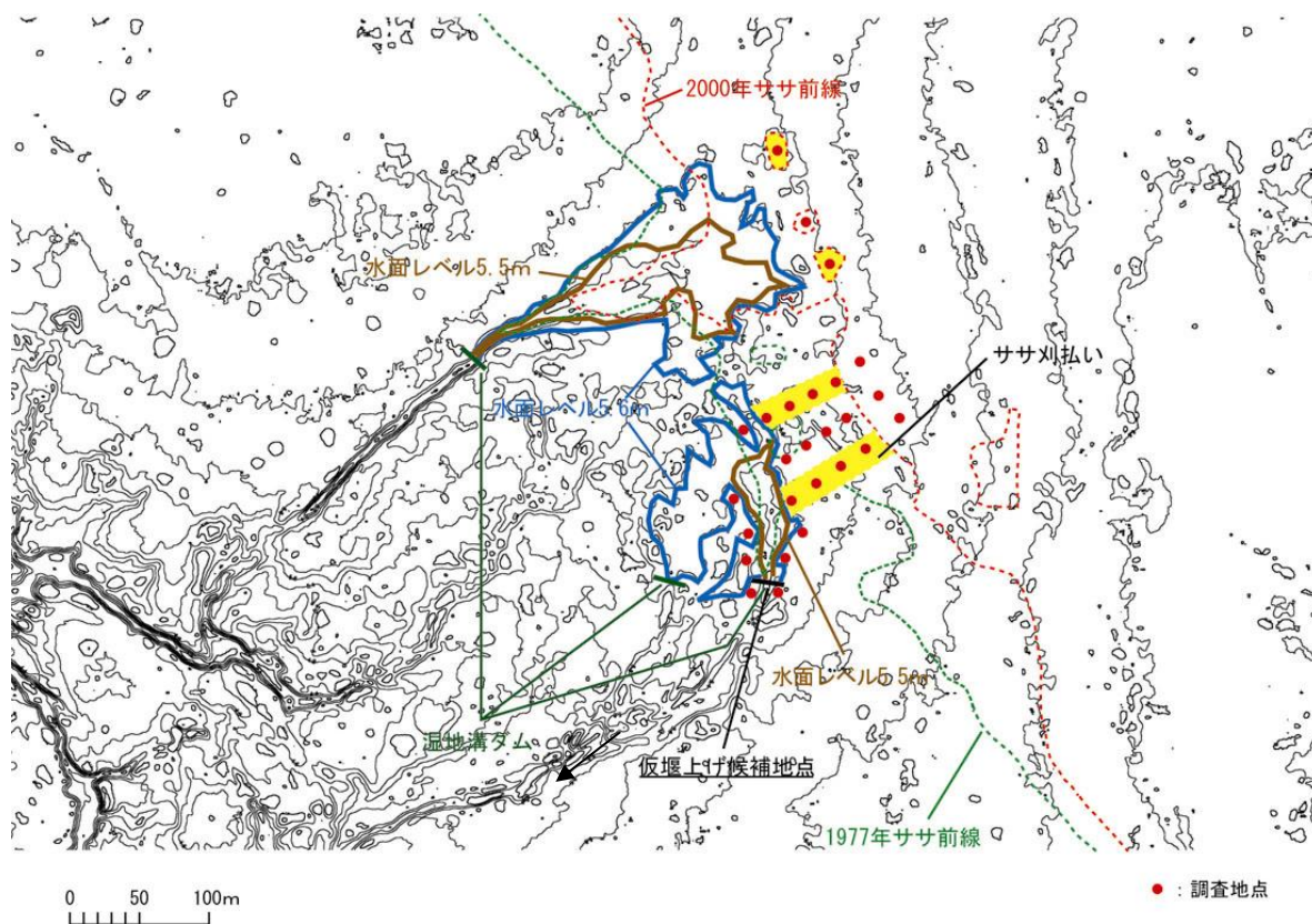
図 5.4.4 湿地溝源頭部を対象とした対策イメージと調査地点
