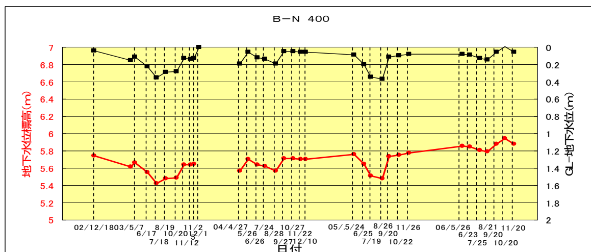
図 4.3.19 ゾーン④（B-N 400地点）の地下水位変動図
