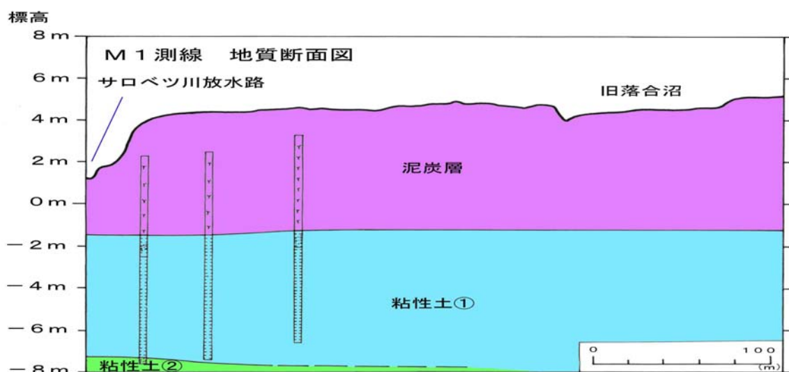
図 7.3.7 M1 測線の地質断面図
