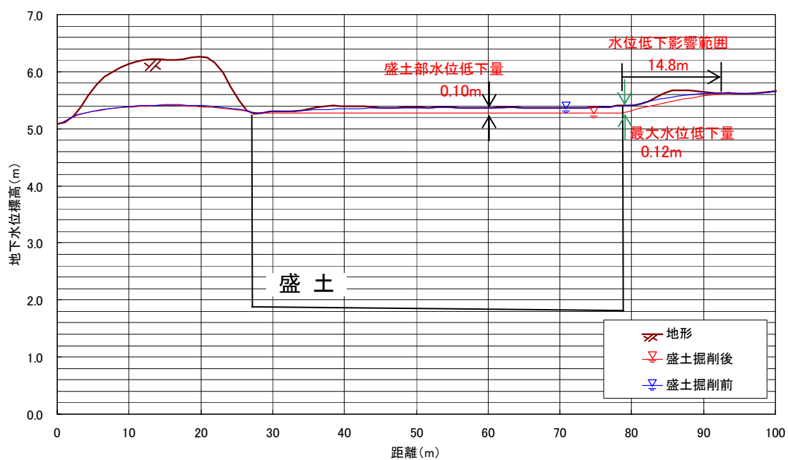
図 6.3.5 地下水位流動解析による掘削前後の地下水位
