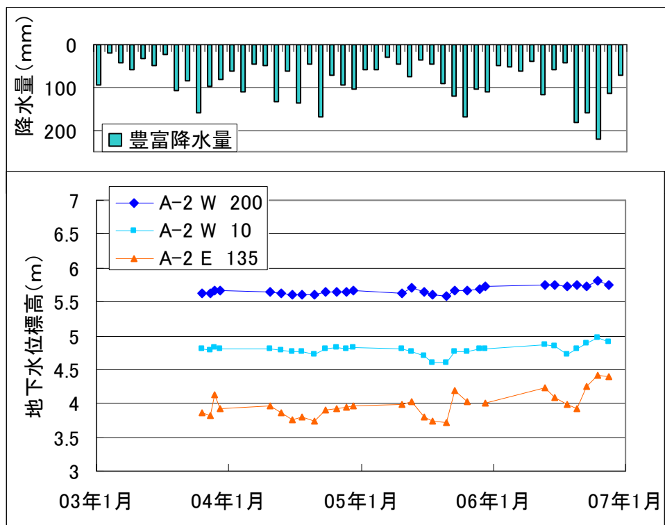
図 4.3.13 A-2 測線代表地点の地下水位変動
