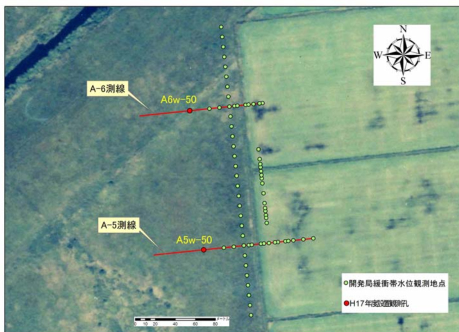
図 4.3.3 A-5およびA-6測線の観測孔配置図
