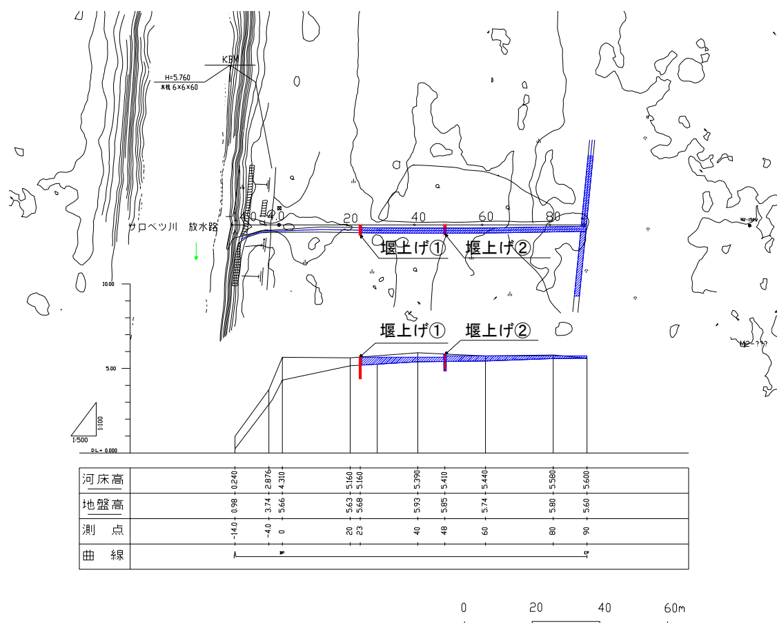
図 7.4.6 水抜き水路②堰上げ計画
