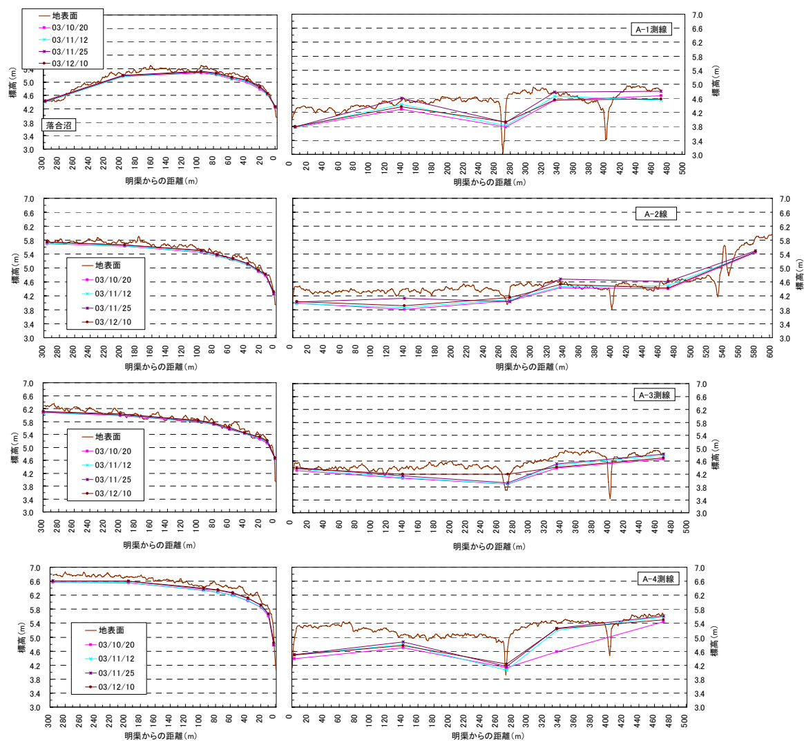
図 8.3.4 A-1～A-4 測線における地下水位観測結果
