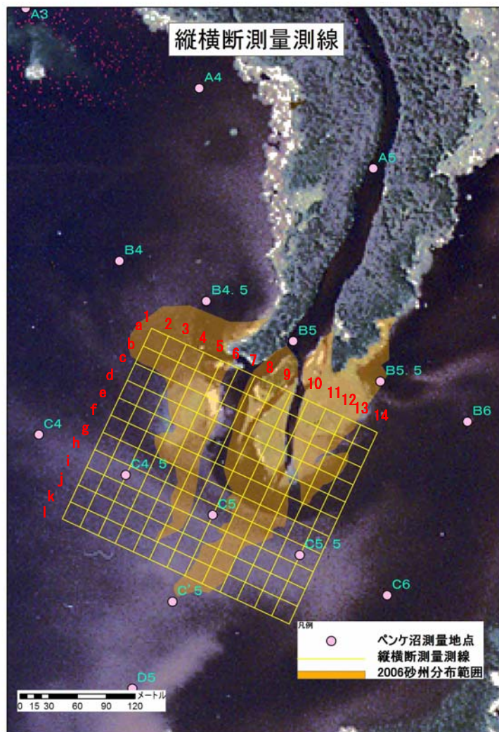
図 9.1.23 ペンケ沼砂州先端部における縦横断測量測線（空中写真は 2000 年撮影）
