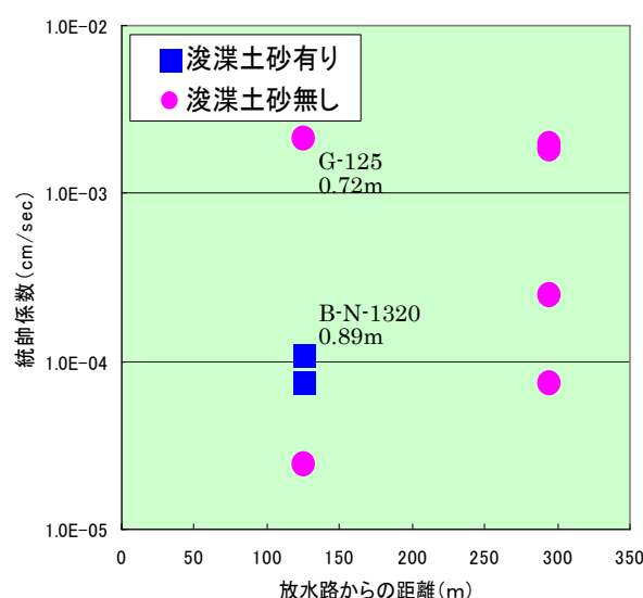
図 7.2.25 放水路からの距離と透水係数の関係
