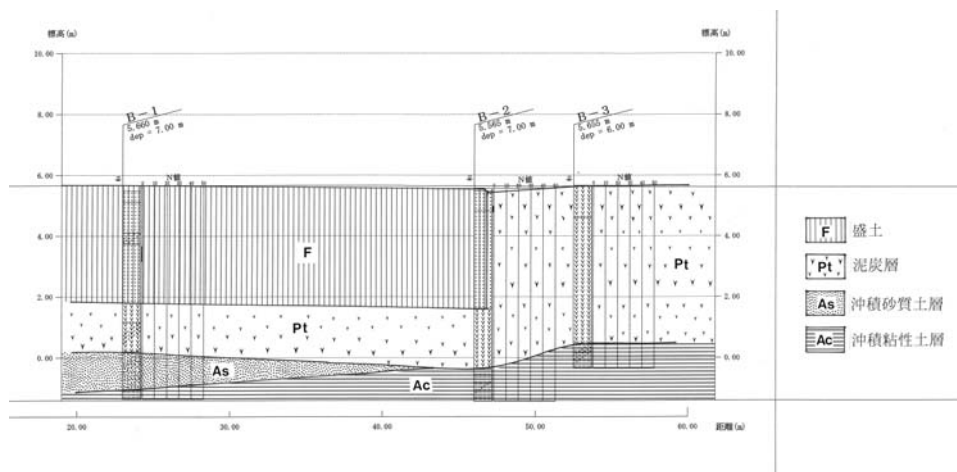
図 6.3.2 南北方向の土質断面図
