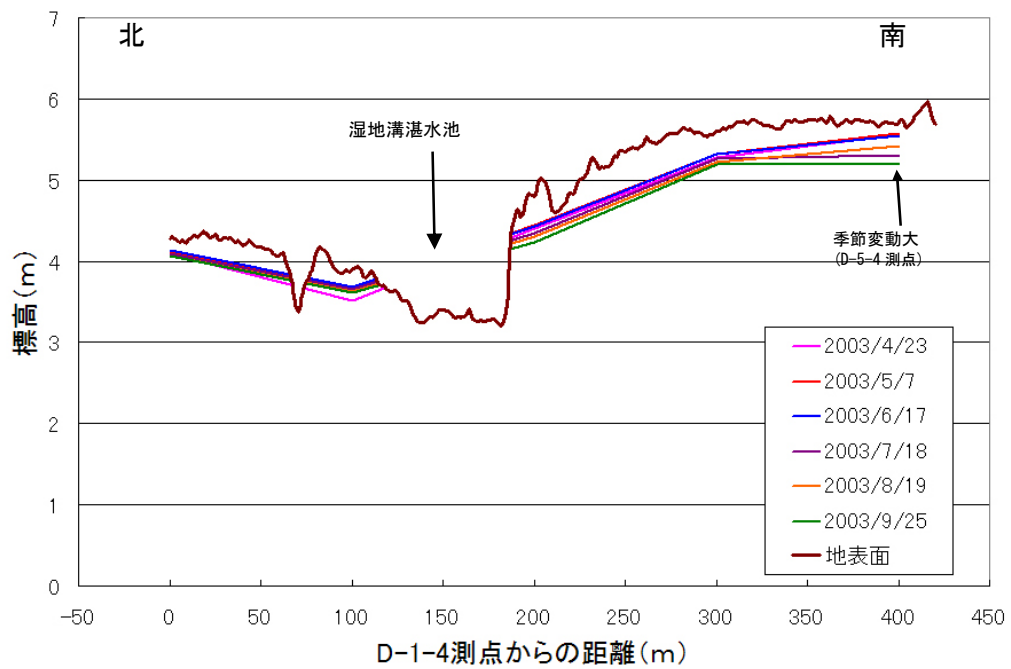
図 4.3.26 D-1-4 測線の地下水位分布 (2003 年)
