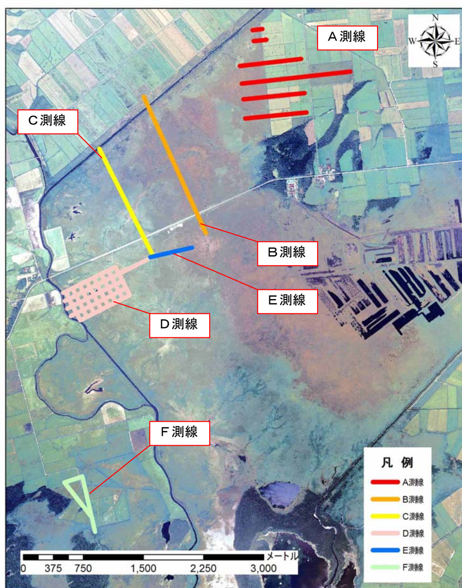
図 4.3.1 各観測測線の配置図
