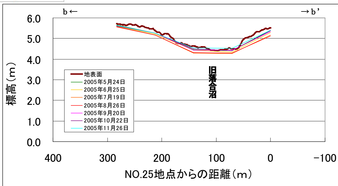
図 7.2.5 水抜き水路 1 b-b' 断面における地下水位分布
