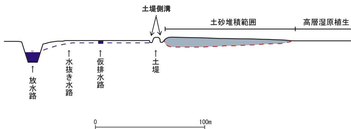
図 7.2.2 放水路周辺の断面模式
