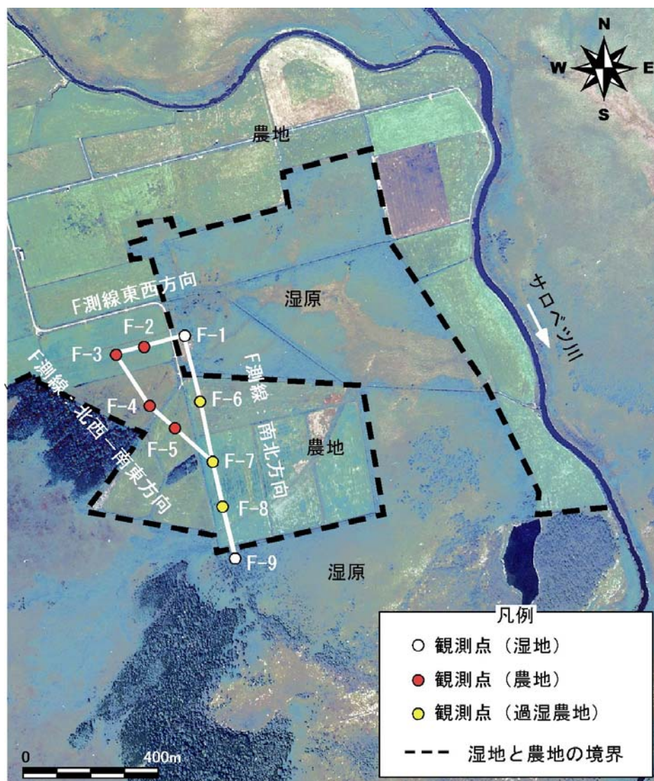
図 4.3.31 F 測線の観測孔配置と領域区分
