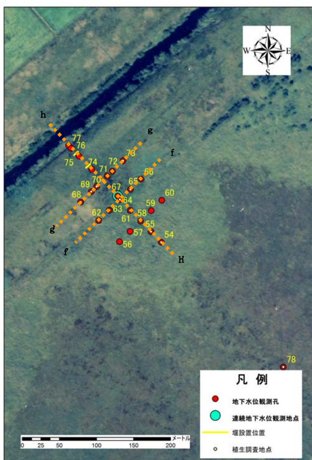
図 7.5.2 水抜き水路 2 堰上げ実証試験地における観測孔位置
