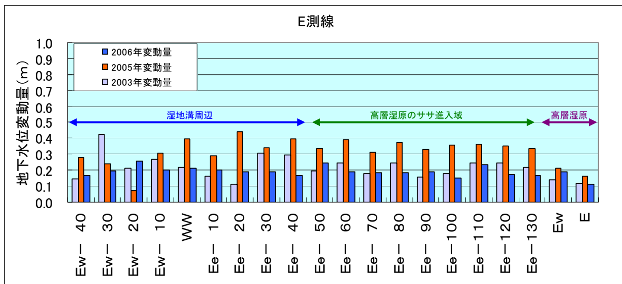
図 4. 3. 30 E測線における 2003 年、2005 年、2006 年の地下水位変動量の比較
