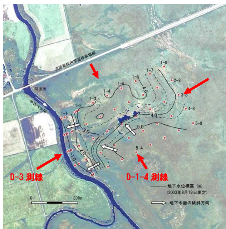
図4.3.24 D測線における地下水位の平面分布
