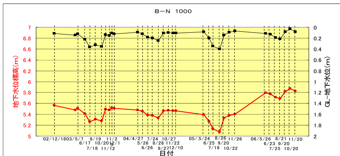
図 4.3.21 ゾーン⑥（B-N 1000地点）の地下水位変動図
