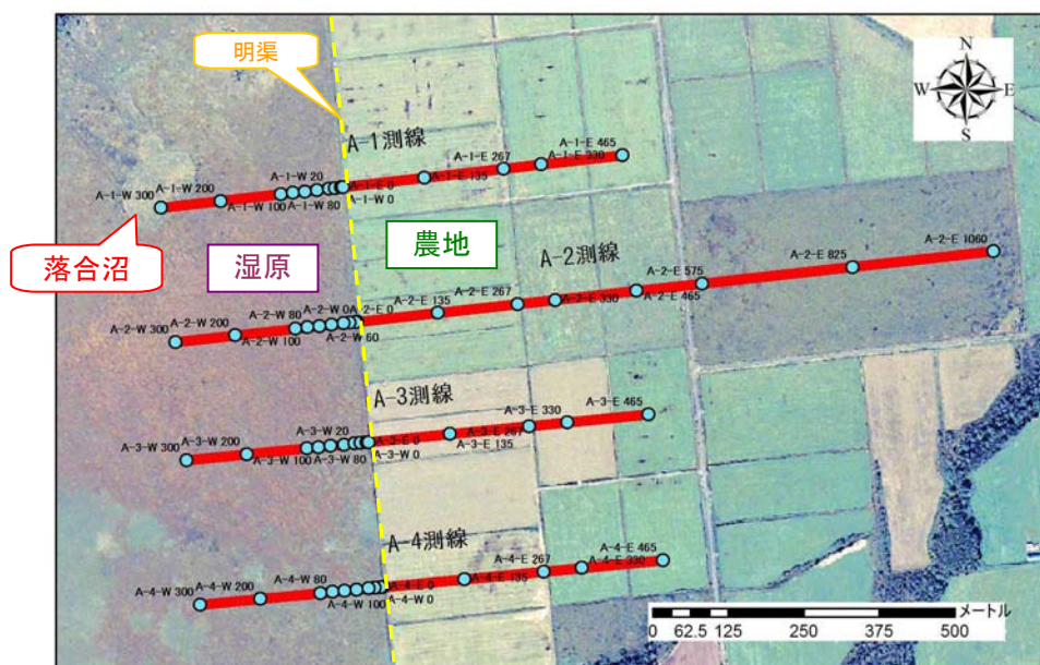
図 8.2.4 A 測線における地下水位観測測線と観測孔位置
