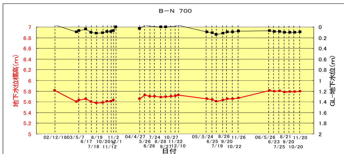
図 4.3.20 ゾーン⑤（B-N 700地点）の地下水位変動図
