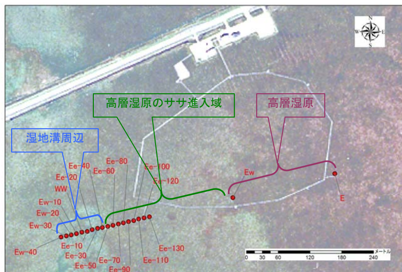
図 4.3.27 E測線の観測孔配置と領域区分
