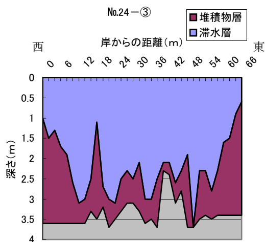
図 10.3.12 横断測線における地形・ブロック状泥炭堆積計測結果
