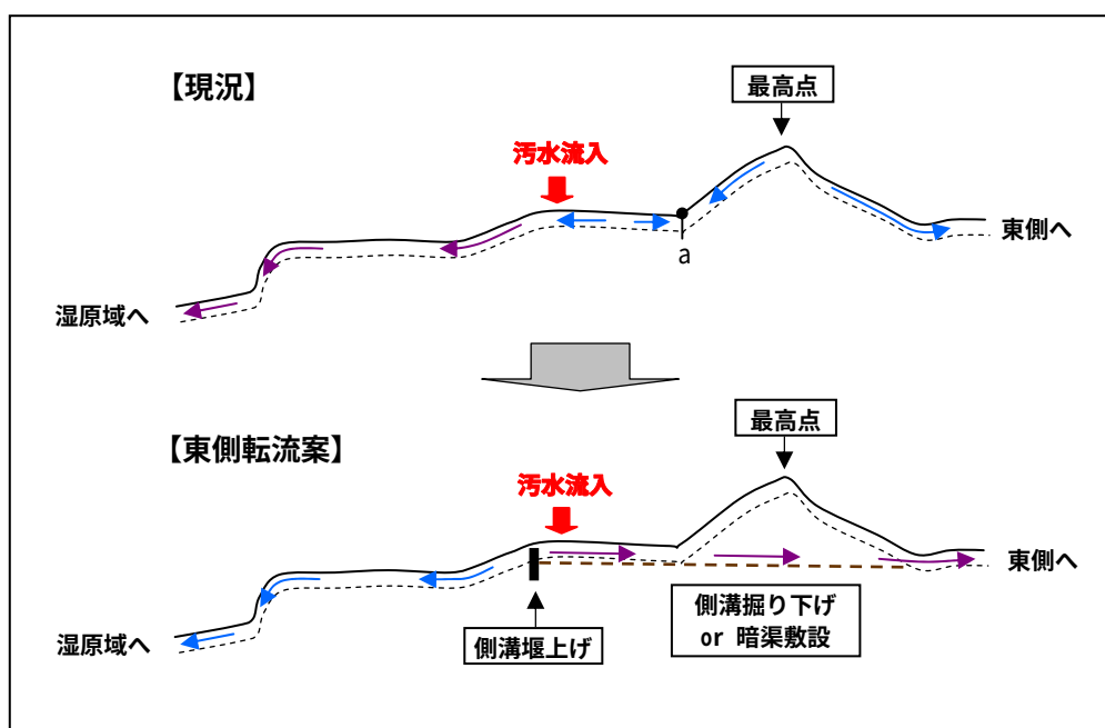
図 6.2.20 ①東側転流案のイメージ
