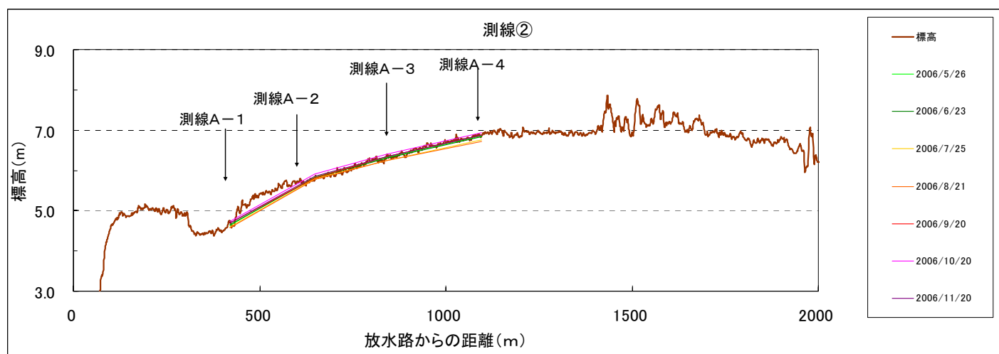
図 4.3.10 測線②における地形と地下水位分布（2006 年）
