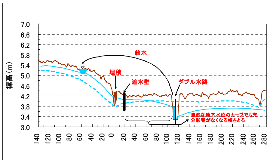
図 8.3.3(2) 緩衝帯の整備イメージ
