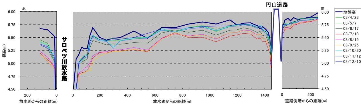
図 7.2.3 地下水位計測結果（B測線）
