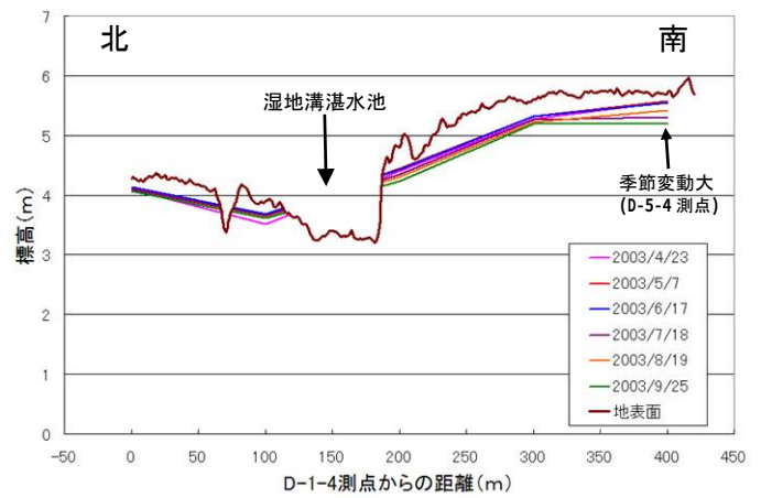
図 5.2.16 D-1-4 測線(D-3 測線に直交方向)の地下水位分布
