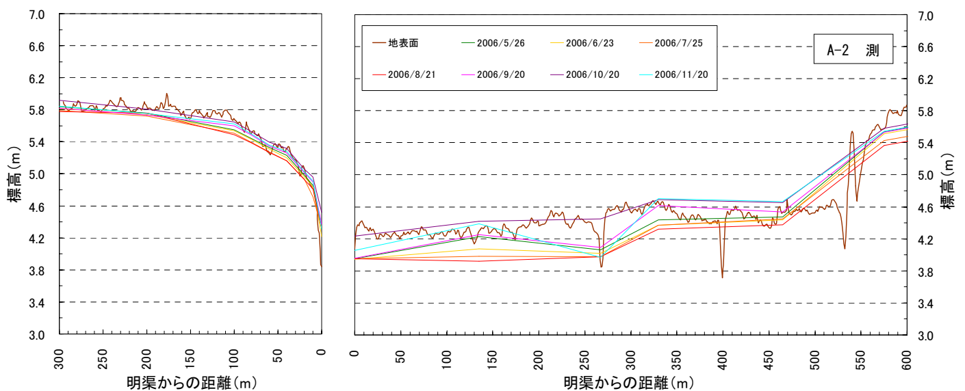
図 4.3.5 A－2 測線の地形と地下水位分布（2006 年）
