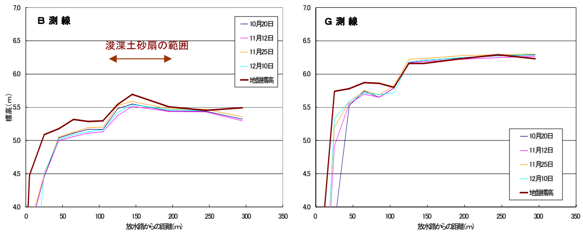
図 7.2.26 B測線及びG測線における地下水位分布
