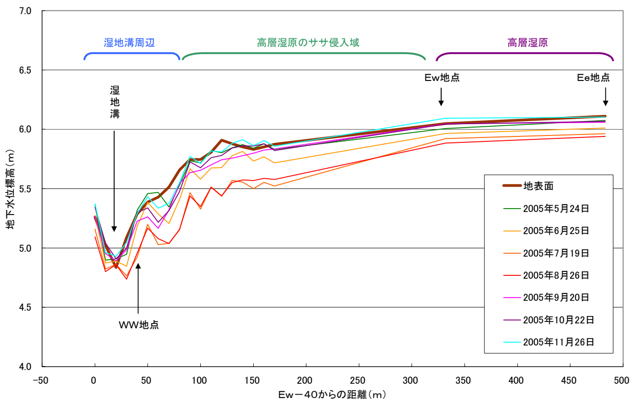
図 4.3.28 2005 年の E 測線の地下水位分布
