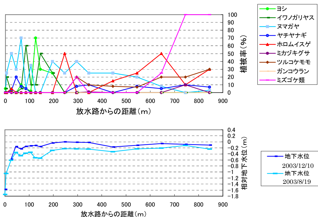
図 7.2.30 B測線における地下水位と主な種の植被率
