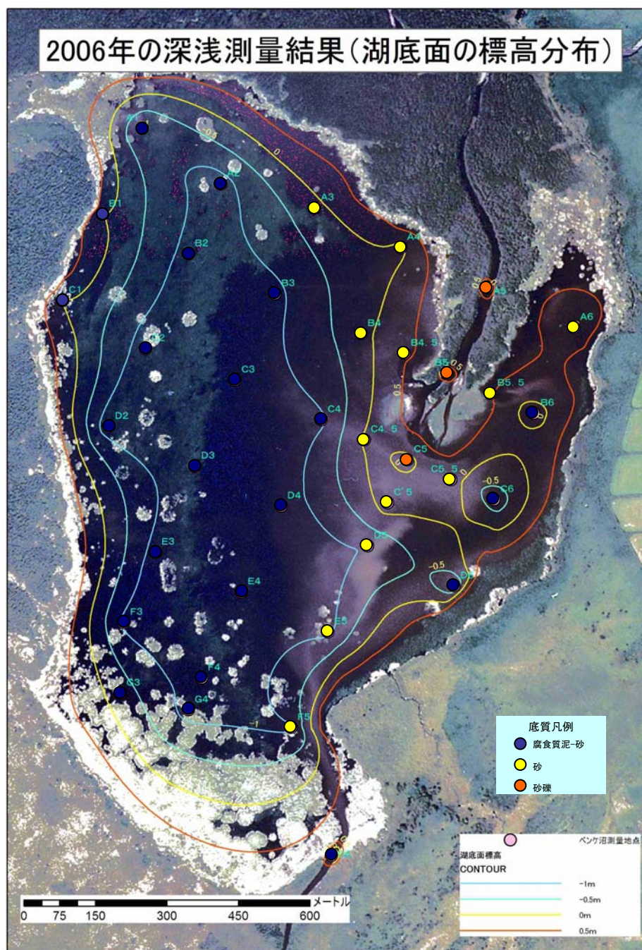
図 9.1.30 2006 年のペンケ沼湖底面標高コンター
