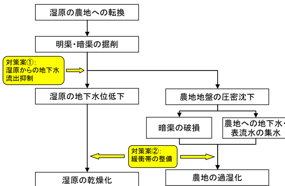
図 8.3.1 推定される劣化のメカニズムと対策
