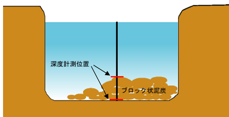
図 10.3.9 深度およびブロック状泥炭堆積厚の計測位置
