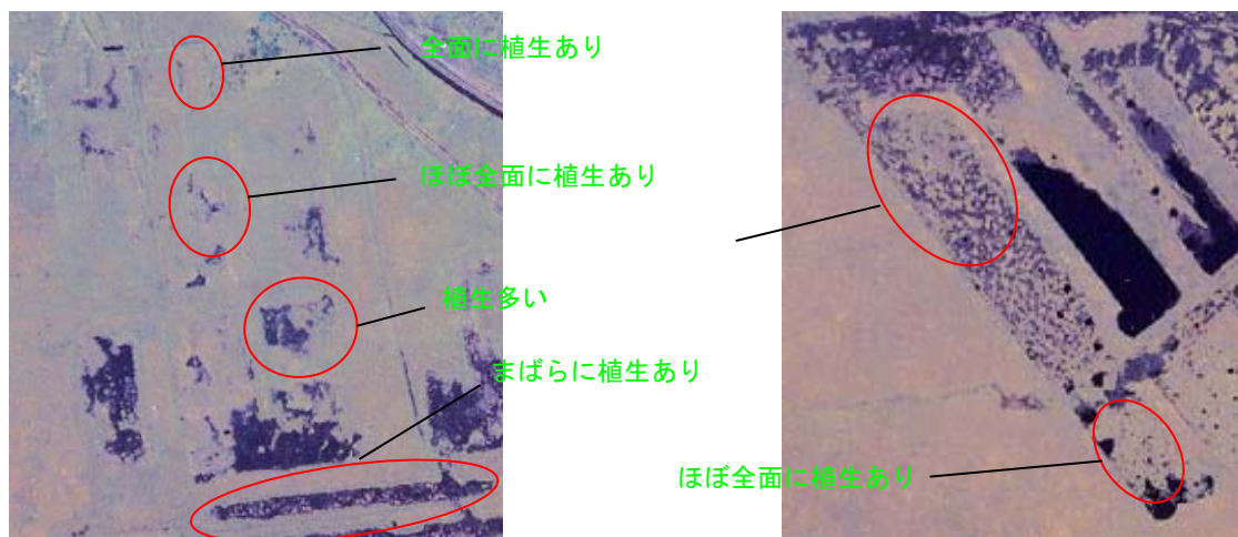
図 10.2.21 植生の変遷
