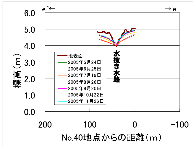
図 7.2.8 水抜き水路 1 e-e' 断面における地下水位分布
