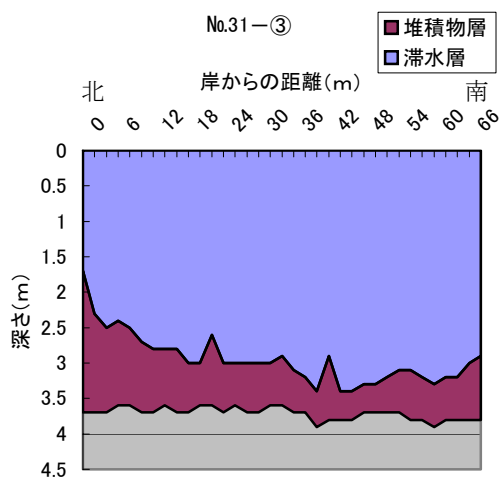
図 10.3.13 横断測線における地形・ブロック状泥炭堆積計測結果
