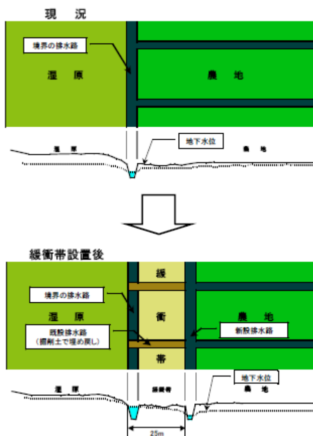
図 8.5.1 北海道開発局による緩衝帯整備のイメージ
