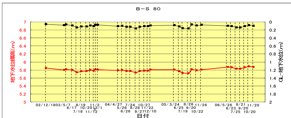
図 4.3.17 ゾーン②（B-S 80地点）の地下水位変動図
