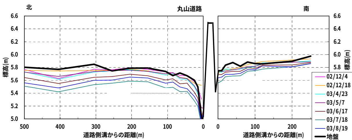
図 6.2.3 丸山道路周辺の地下水位の断面分布（B 側線）
