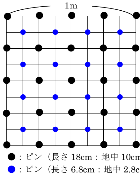
図 10.2.26 計測用ピンの配置
