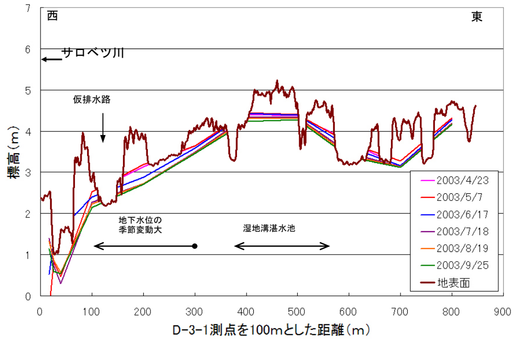
図 4.3.25 D-3 測線の地下水位分布 (2003 年)
